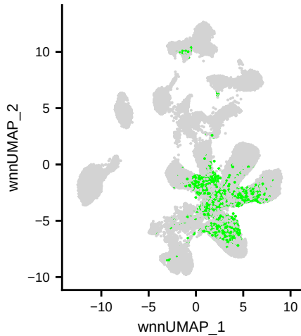
GPR151
