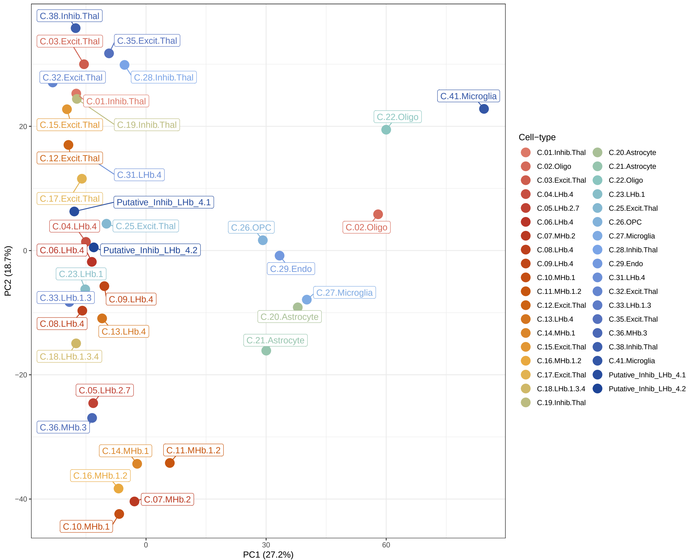
Pseudobulk PCA of all Multiome Fine Clusters
