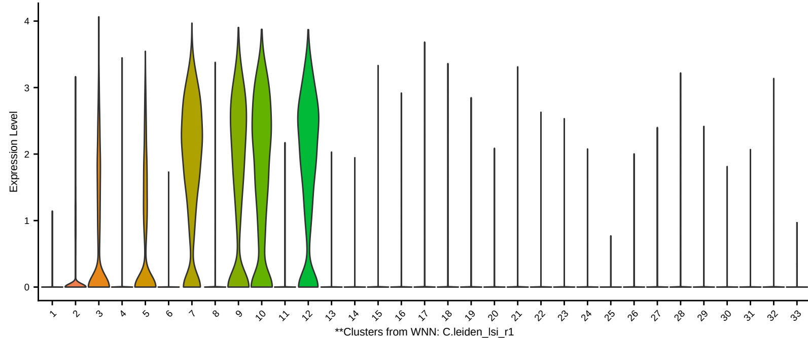
GPR151
