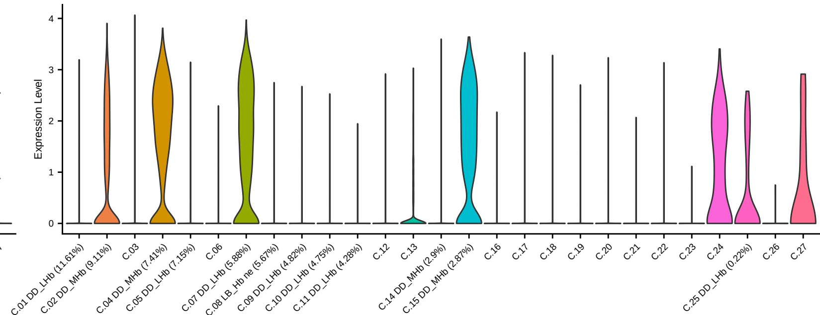
GPR151
