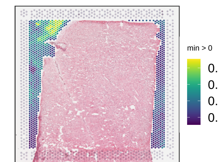
Br5460 expr_chrM_ratio
