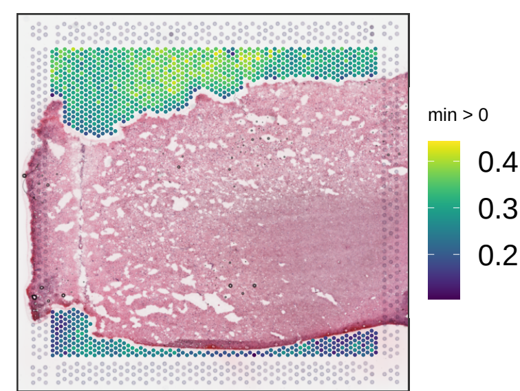
Br1039 expr_chrM_ratio
