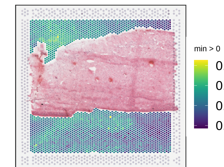
Br5367 expr_chrM_ratio
