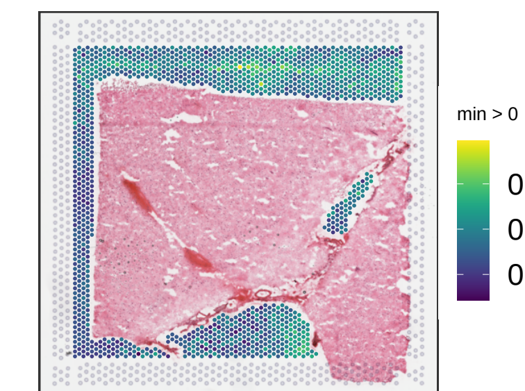
Br6321 expr_chrM_ratio
