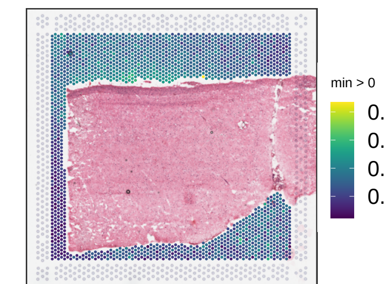
Br6263 expr_chrM_ratio
