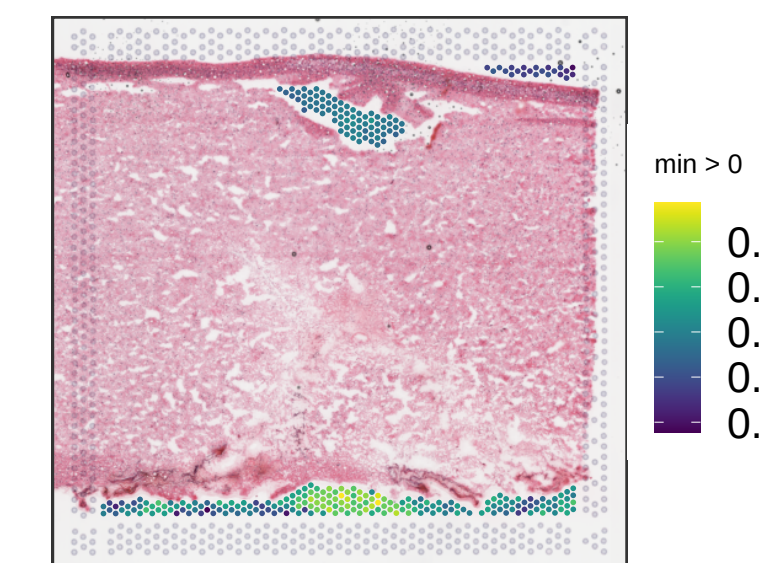
Br5161 expr_chrM_ratio
