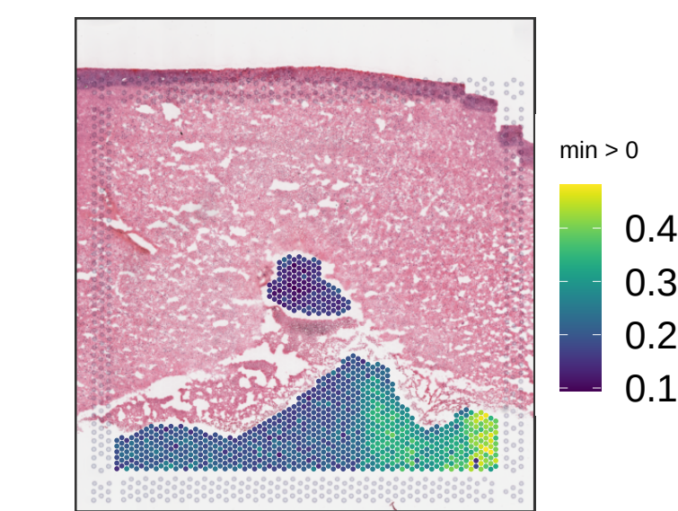
Br6085 expr_chrM_ratio
