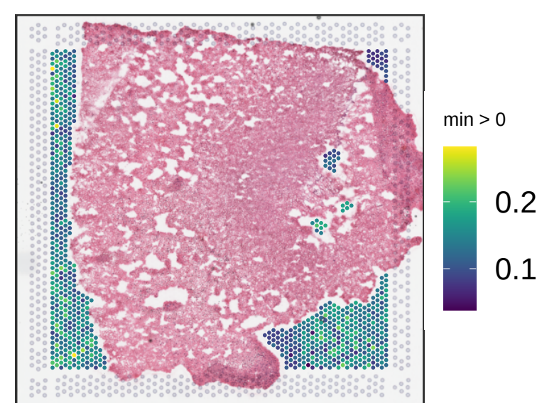
Br6538 expr_chrM_ratio
