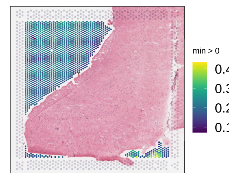
Br1289 expr_chrM_ratio
