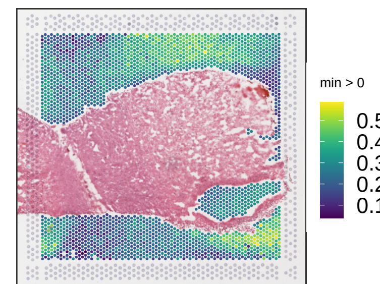
Br3974 expr_chrM_ratio
