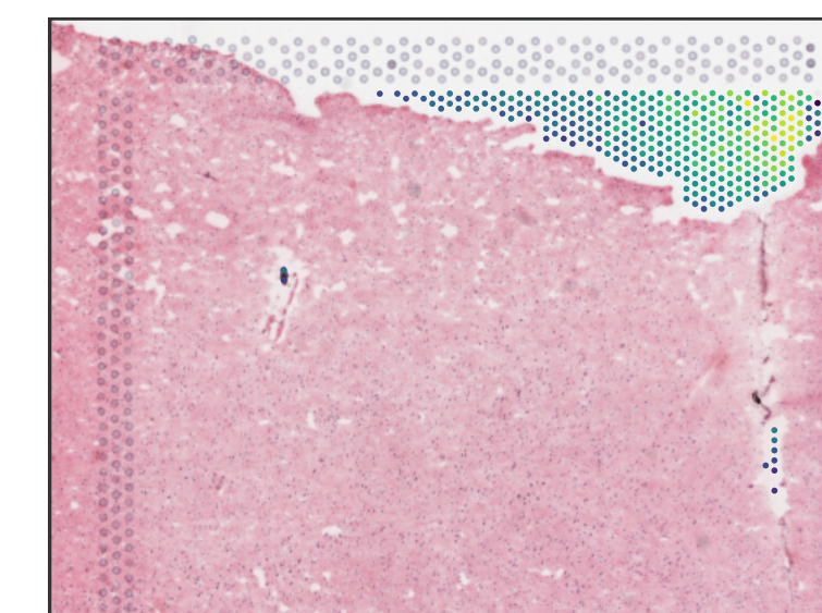
Br5212 expr_chrM_ratio
