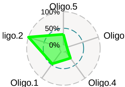
Oligo-M5
