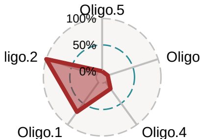
Oligo-M1
