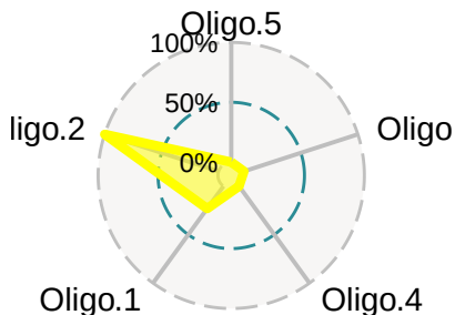
Oligo-M4
