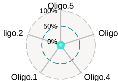
Oligo-M3
