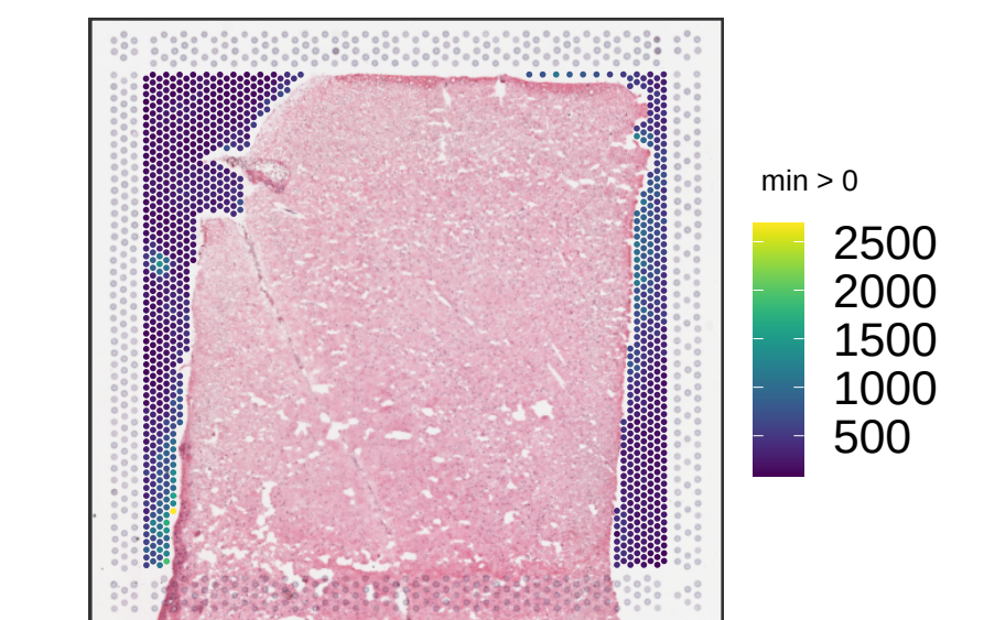
V13Y24-342_D1 sum_gene
