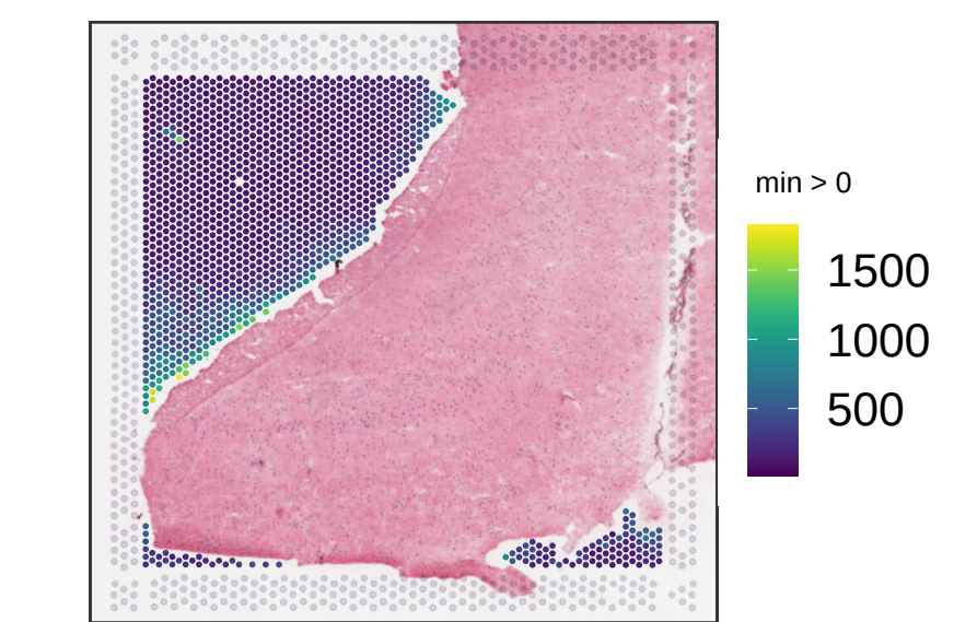
V13B23-364_D1 sum_gene
