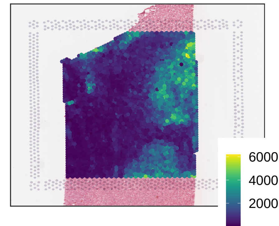
V13M06-387_D1 sum_gene
