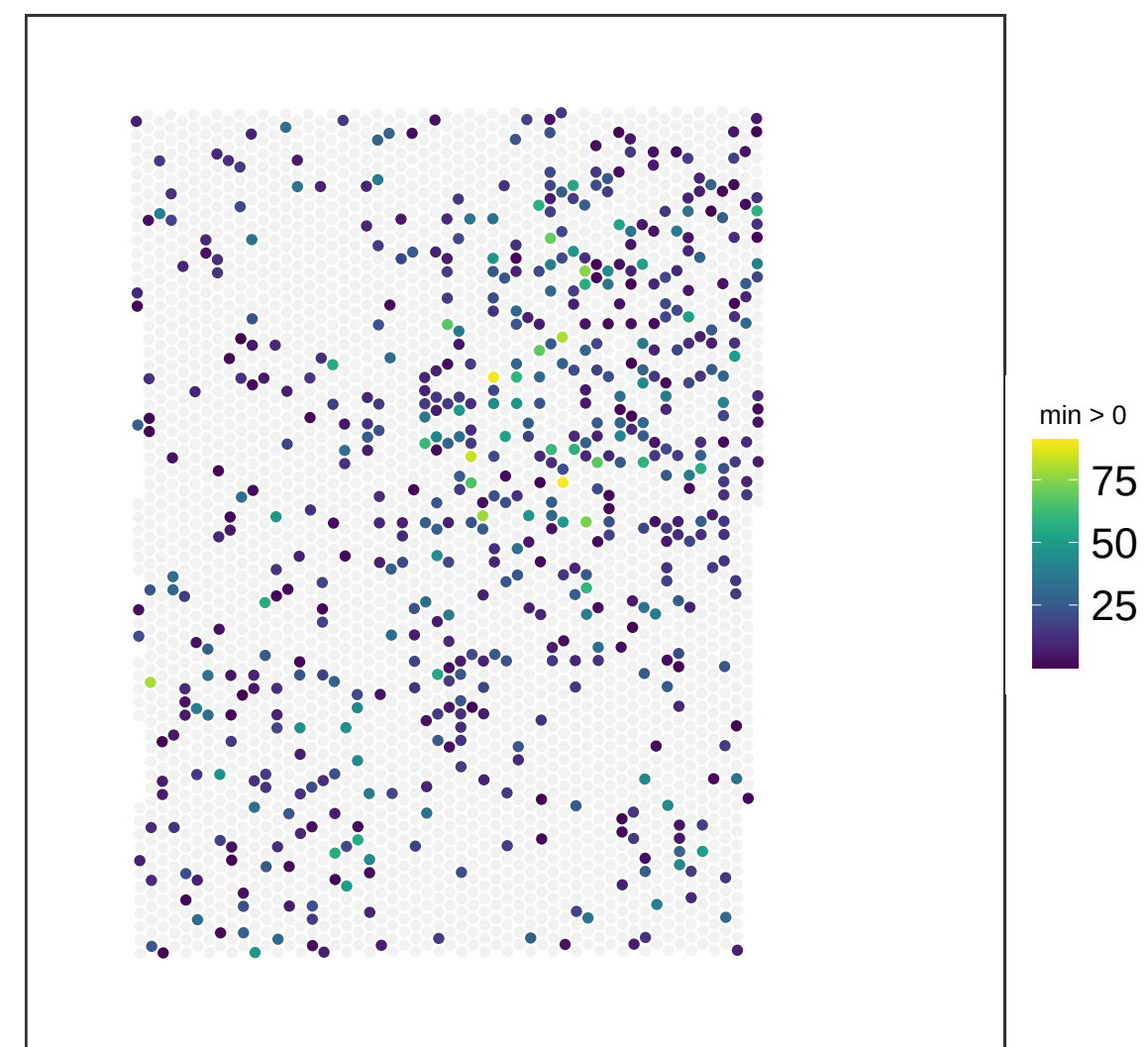
V13M06-387_C1 NMF_47
