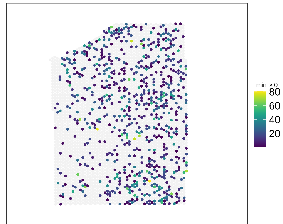
V13M06-387_D1 NMF_47
