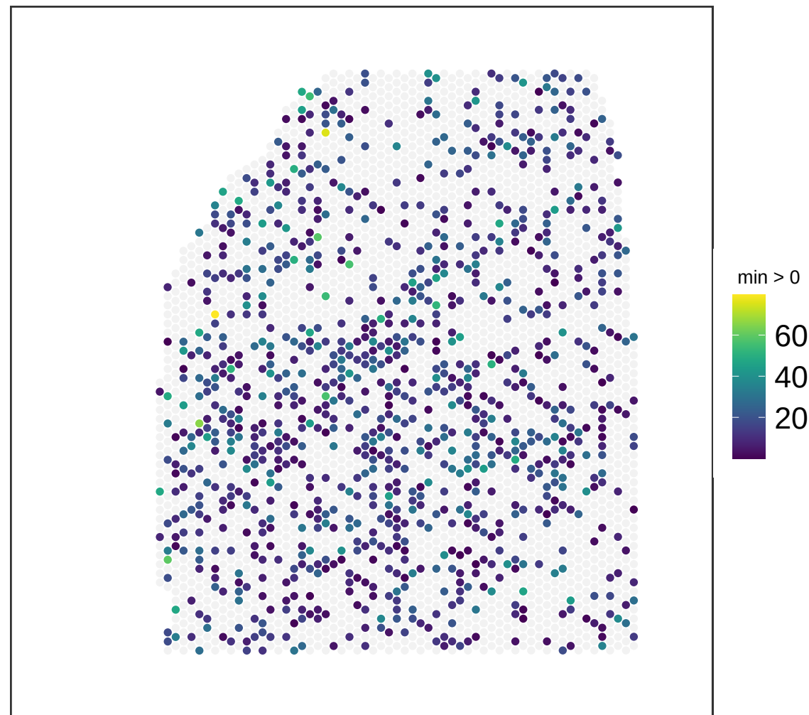
V13M06-388_B1 NMF_47
