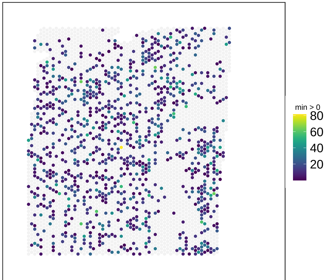
V13M06-388_A1 NMF_47
