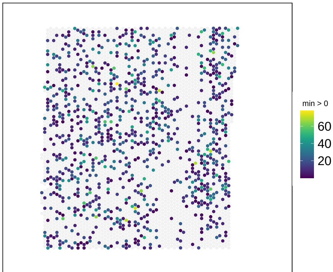
V13M06-388_C1 NMF_47
