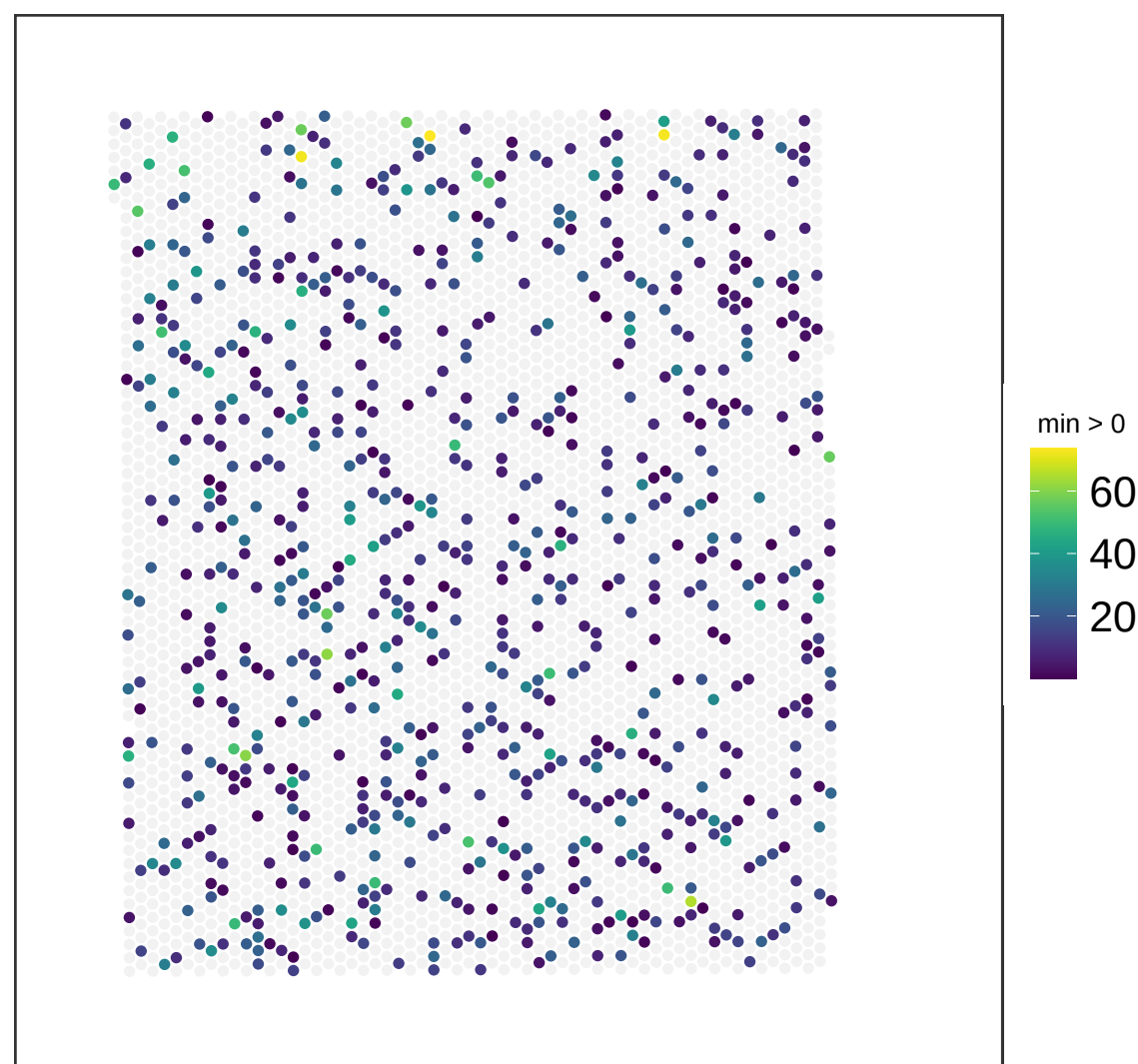
V13M06-387_B1 NMF_47
