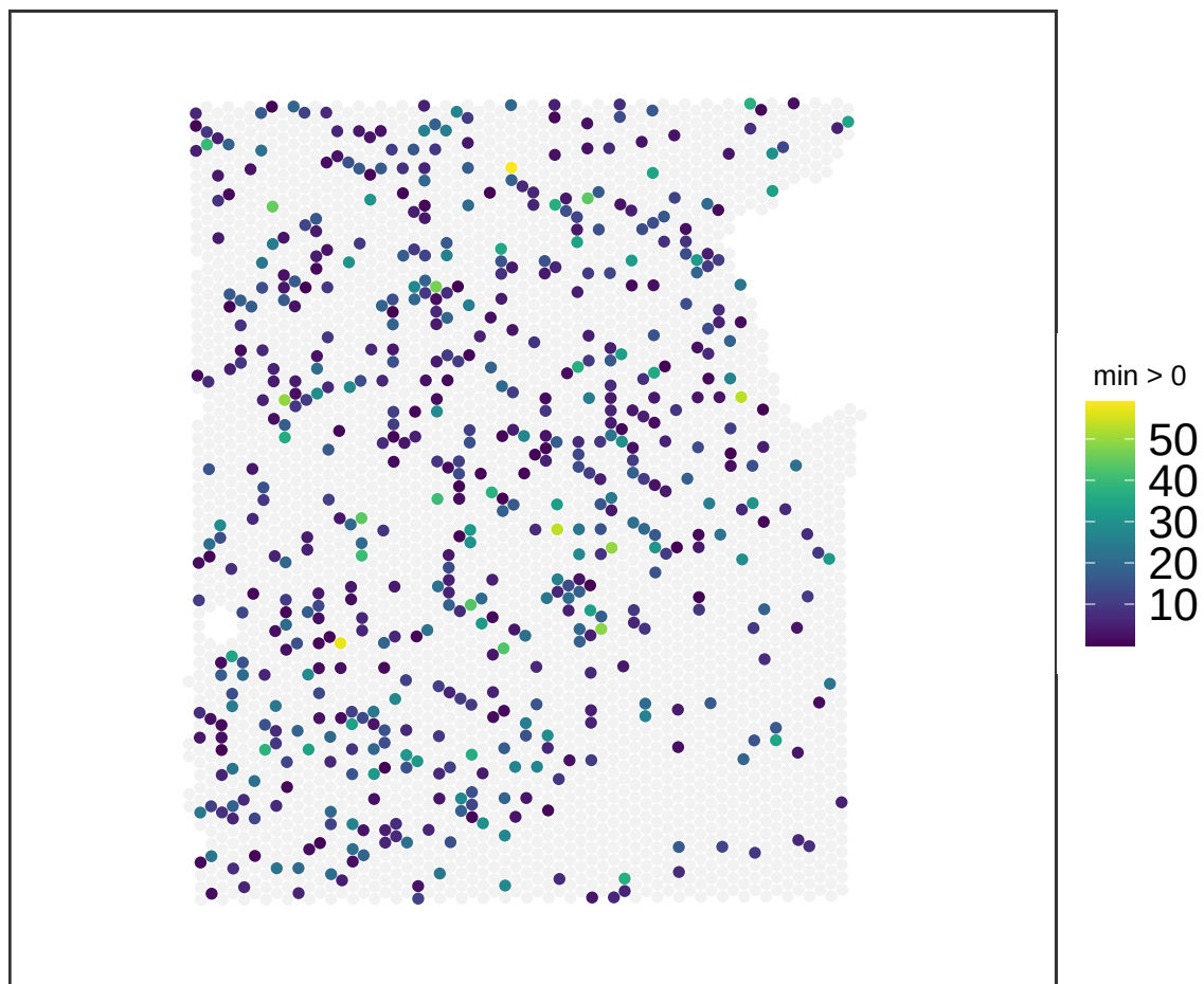
V13M06-387_A1 NMF_47
