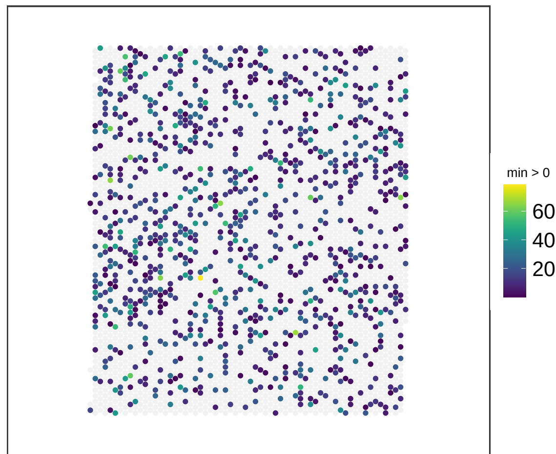
V13M06-388_D1 NMF_47
