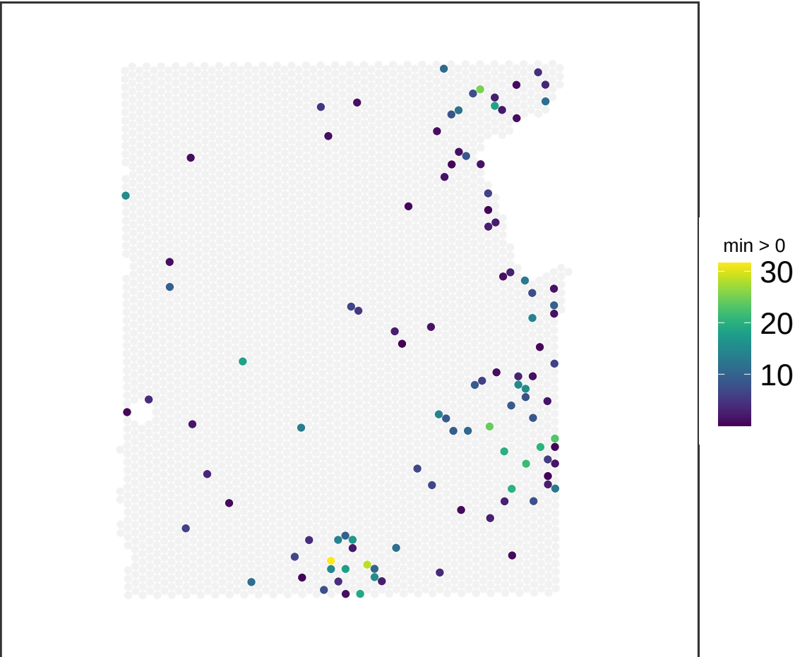
V13M06-387_A1 NMF_50
