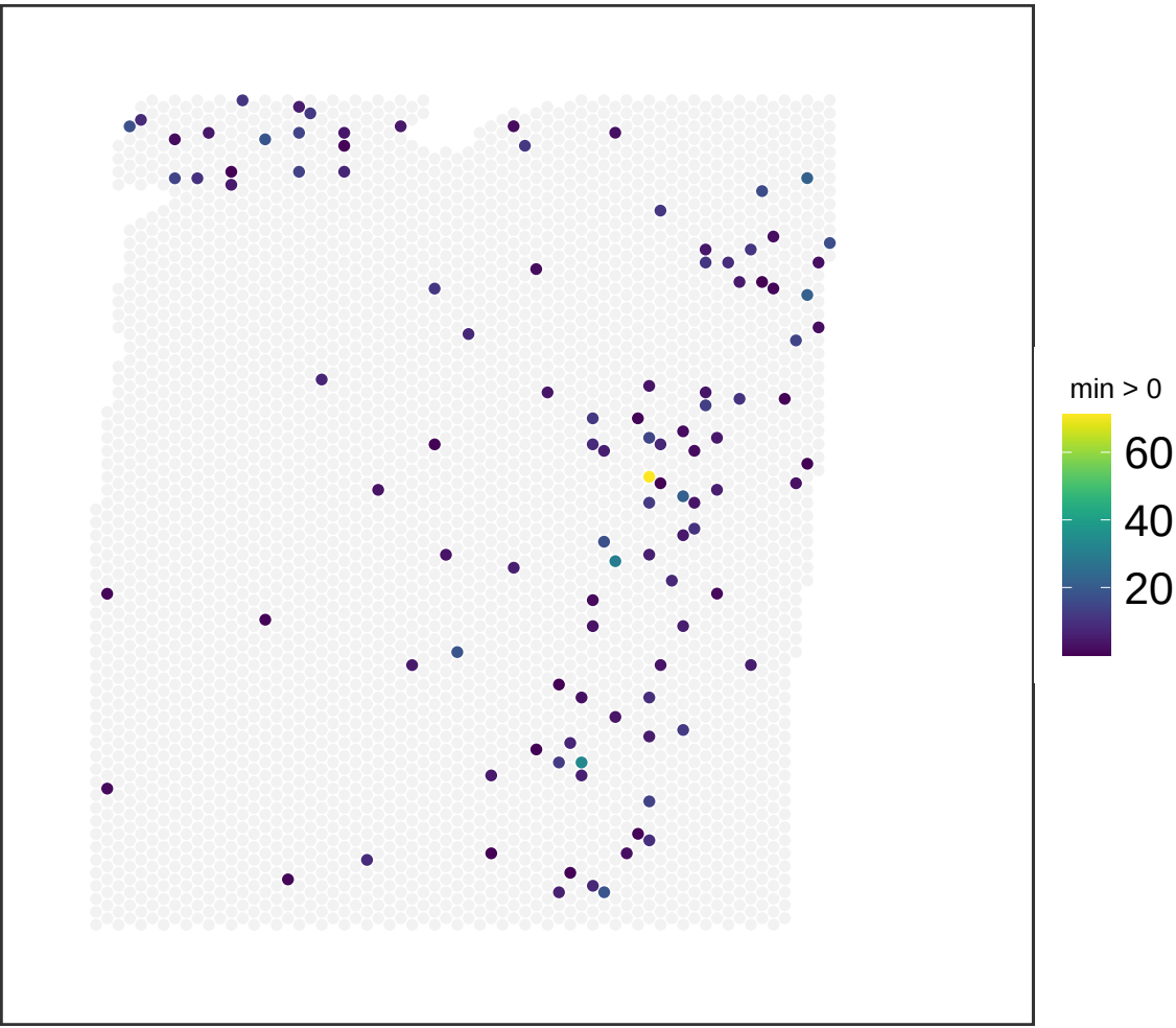
V13M06-388_A1 NMF_50
