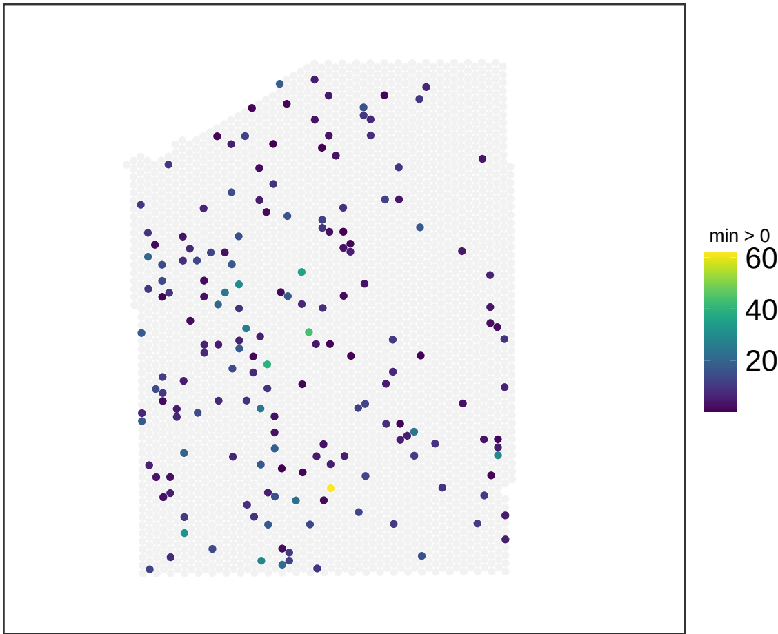
V13M06-387_D1 NMF_50
