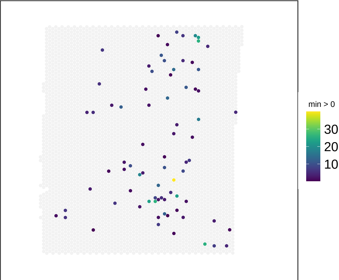
V13M06-388_C1 NMF_50
