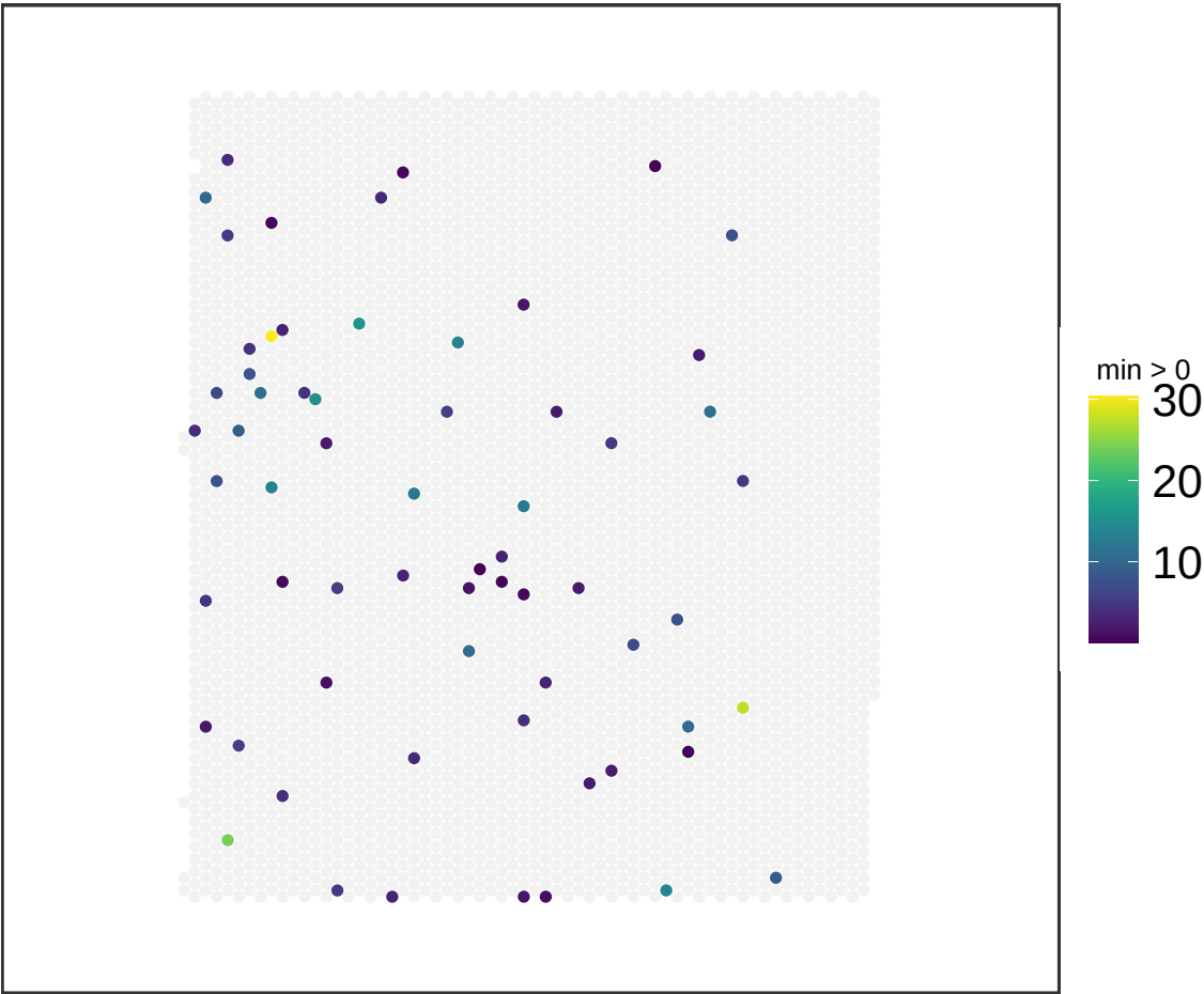
V13M06-388_D1 NMF_50
