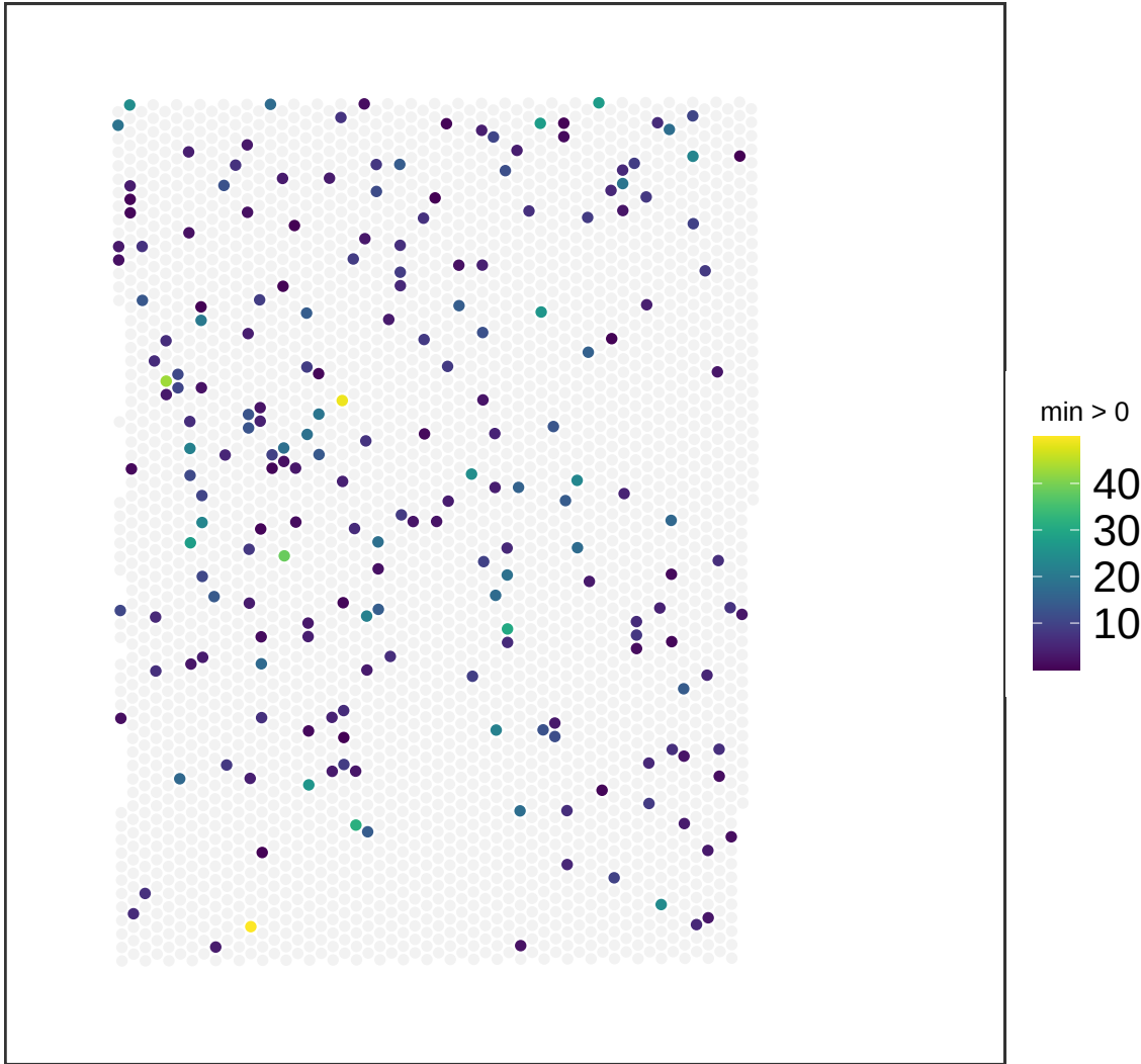
V13M06-387_C1 NMF_50
