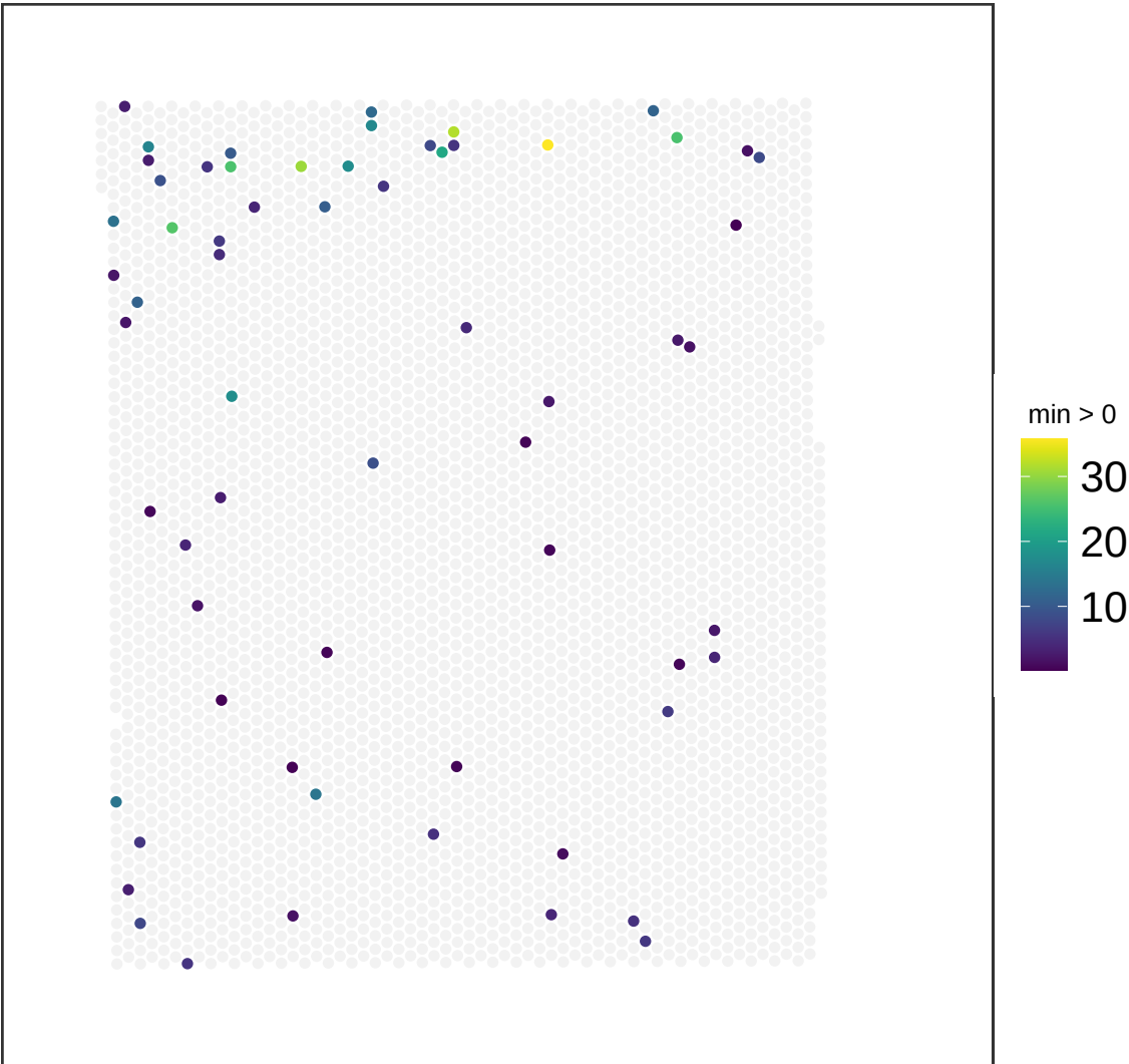
V13M06-387_B1 NMF_50
