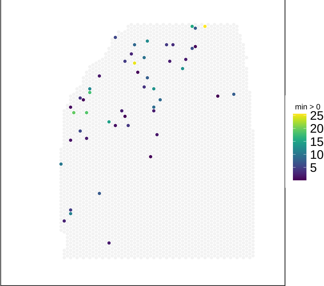
V13M06-388_B1 NMF_50
