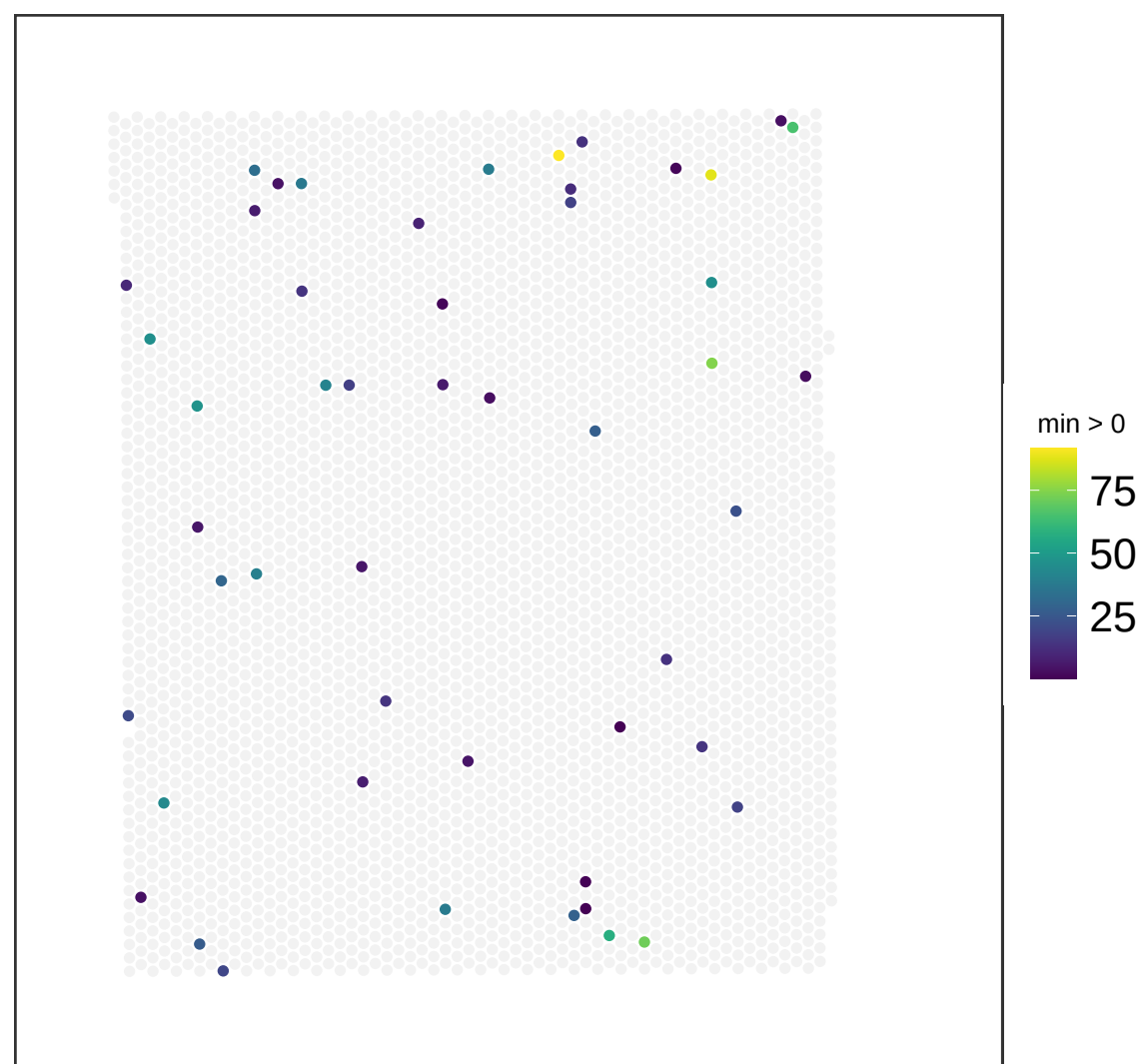
V13M06-387_B1 NMF_54
