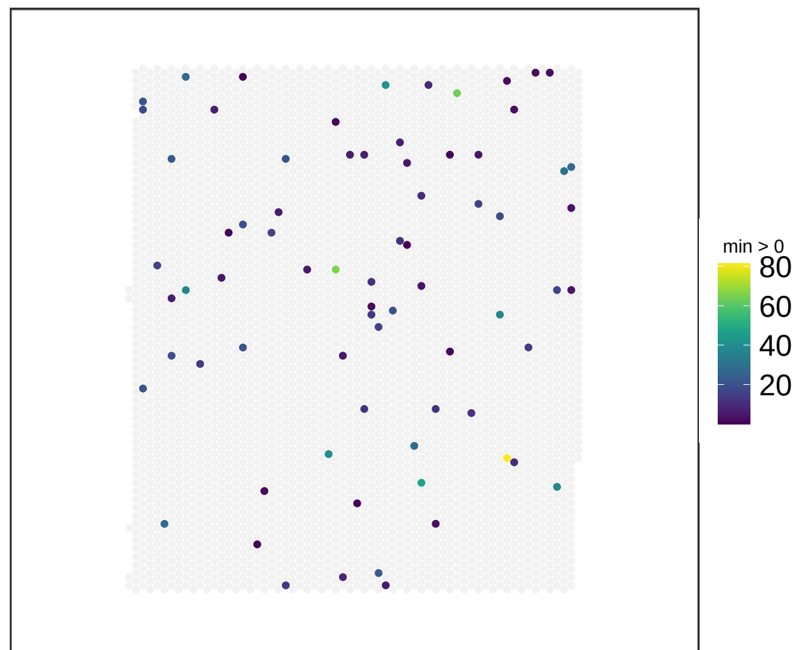
V13M06-388_D1 NMF_54
