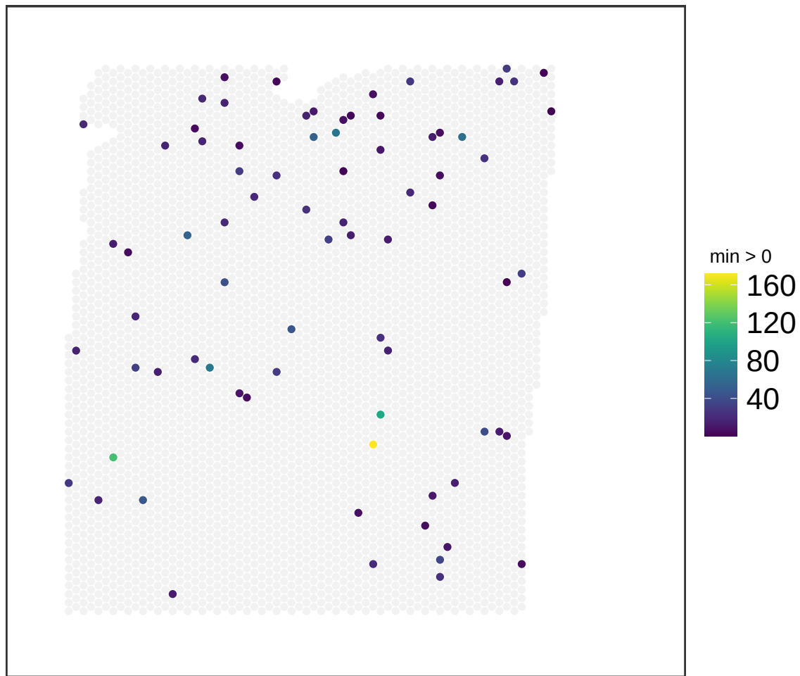
V13M06-388_A1 NMF_54
