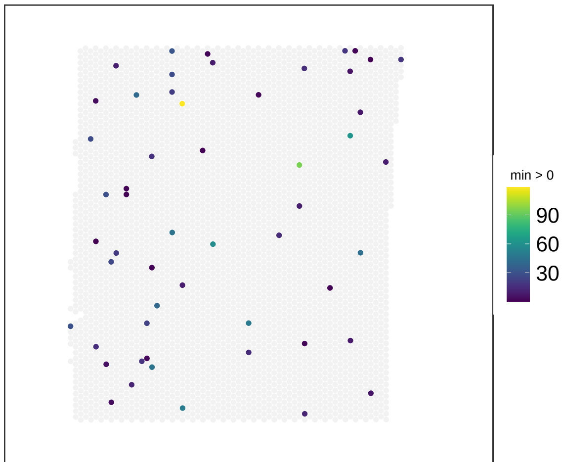
V13M06-388_C1 NMF_54
