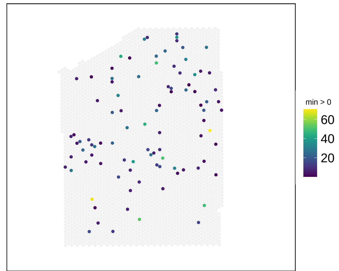
V13M06-387_D1 NMF_54
