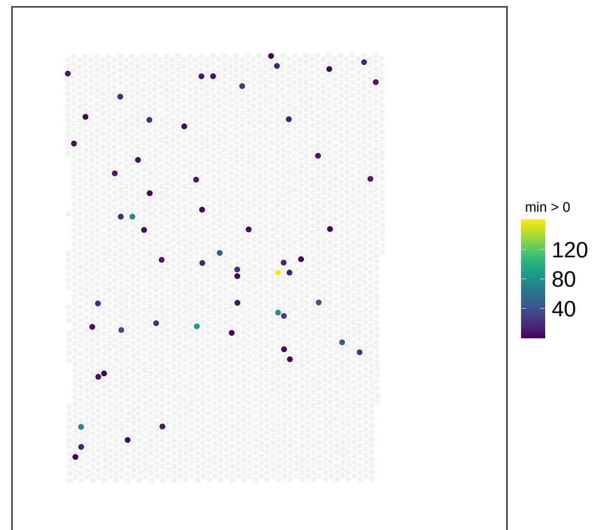
V13M06-387_C1 NMF_54
