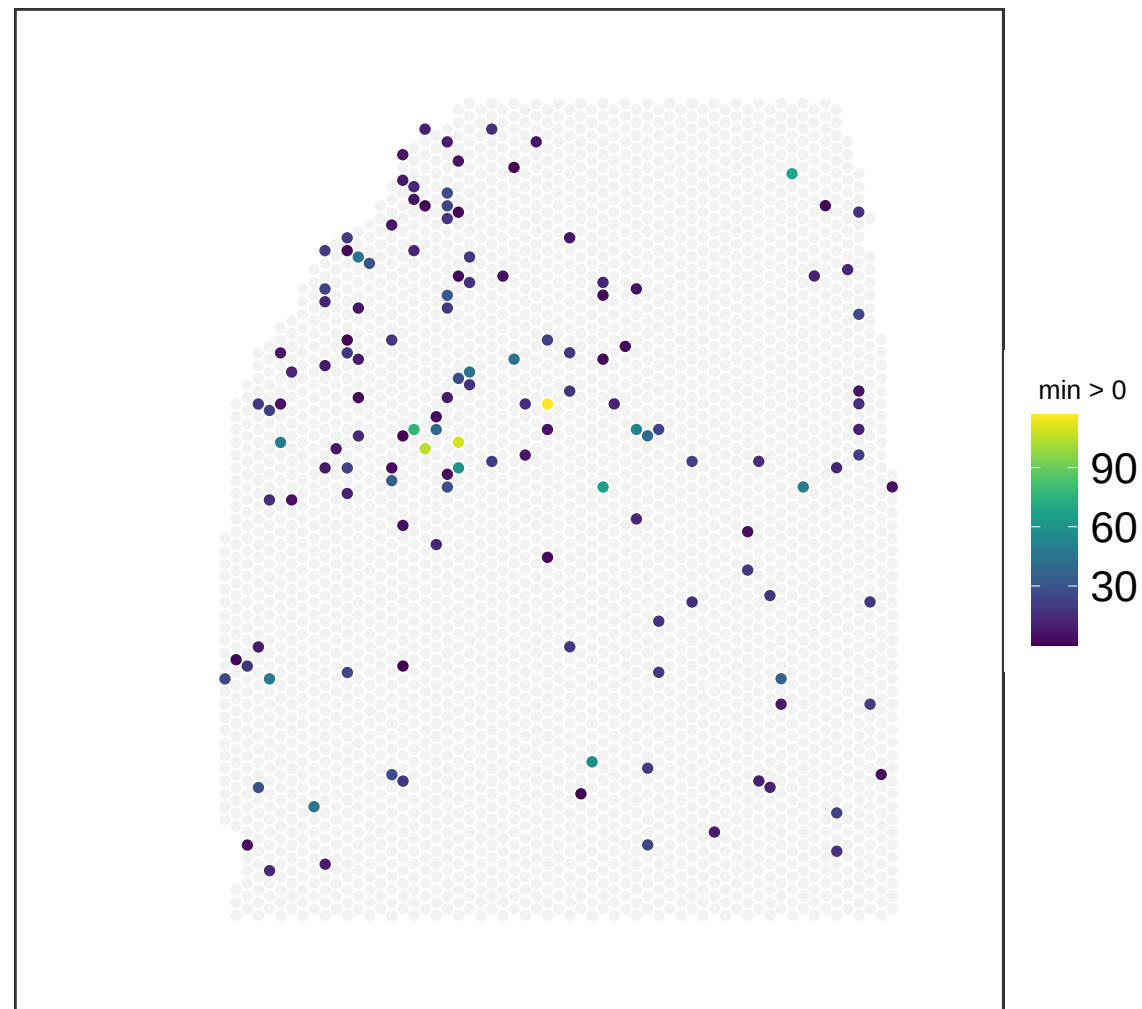
V13M06-388_B1 NMF_54
