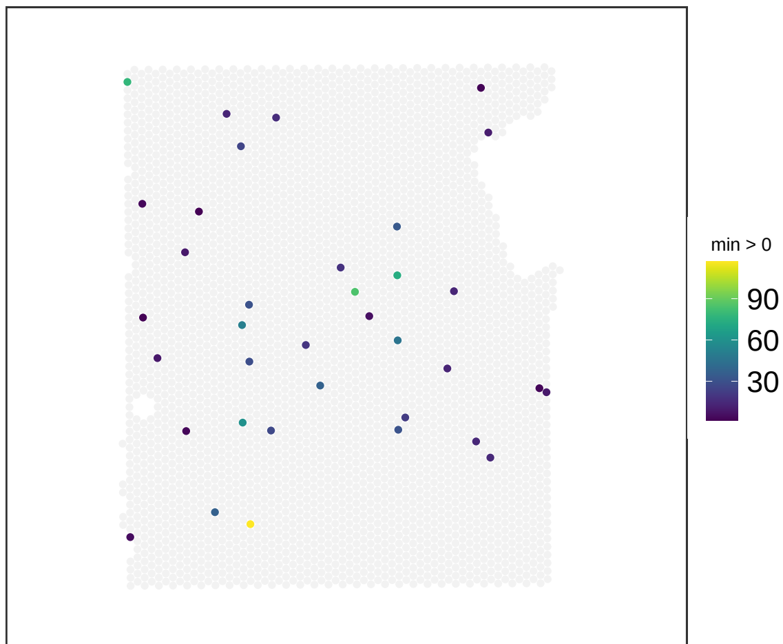
V13M06-387_A1 NMF_54
