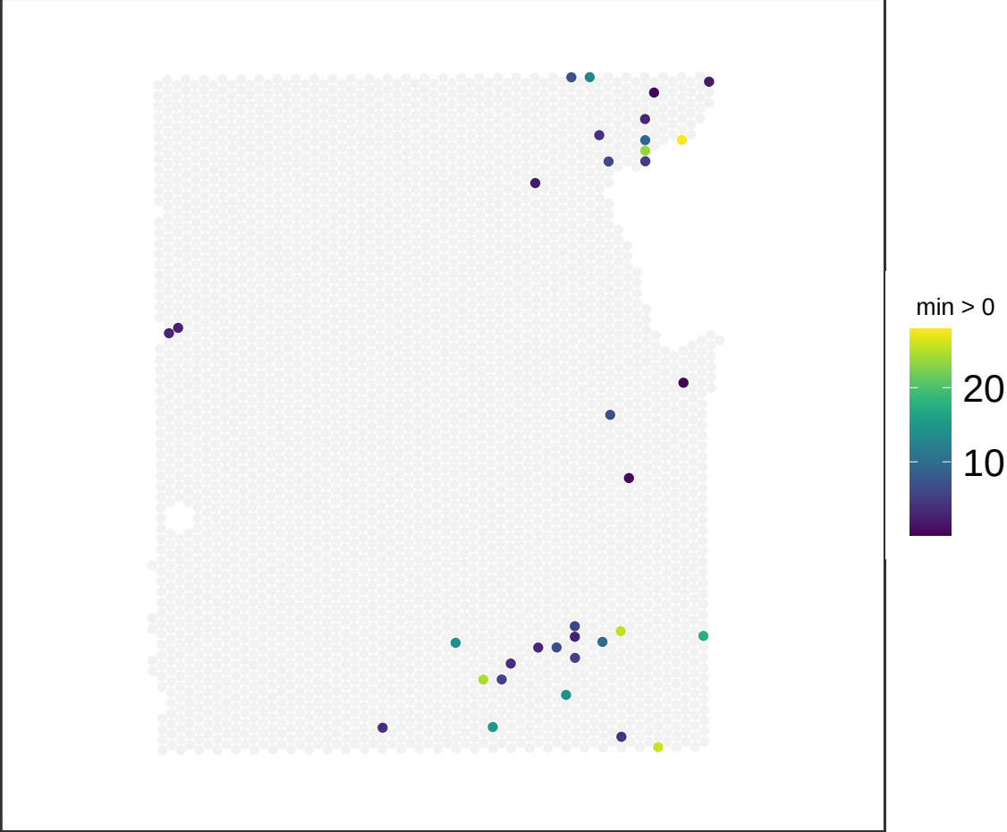
V13M06-387_A1 NMF_61
