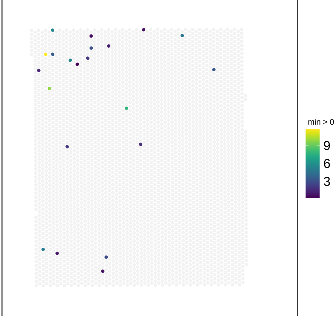
V13M06-387_B1 NMF_61
