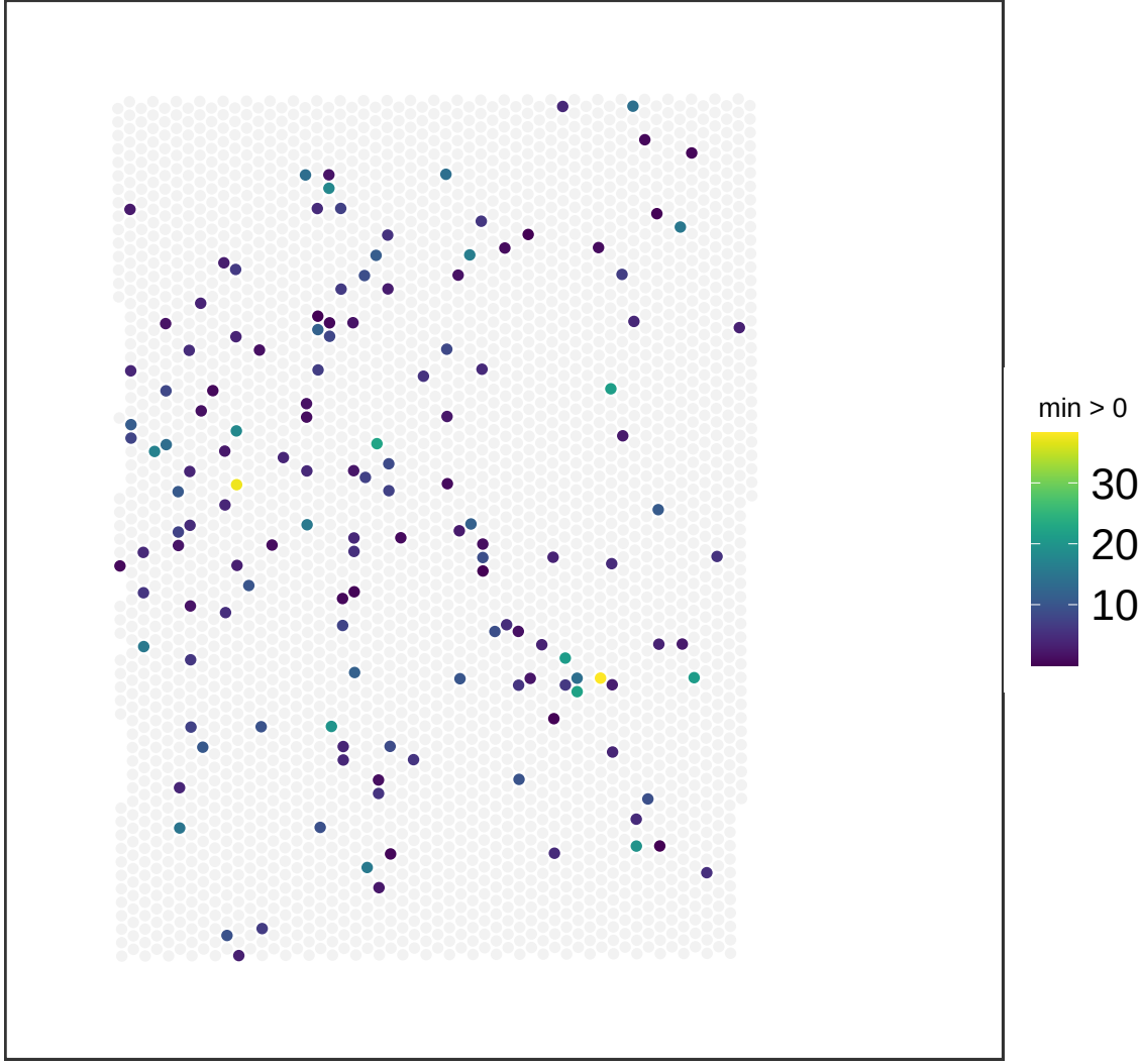
V13M06-387_C1 NMF_61
