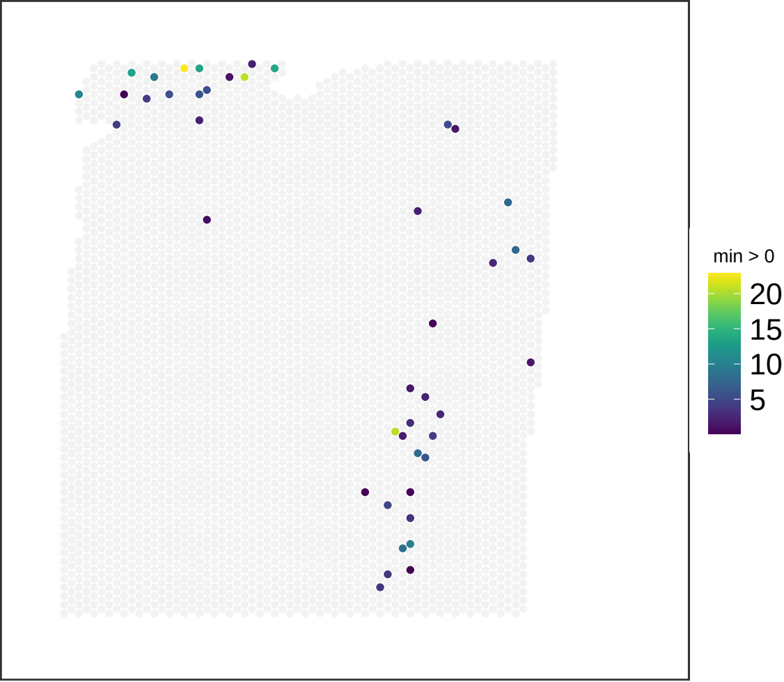
V13M06-388_A1 NMF_61
