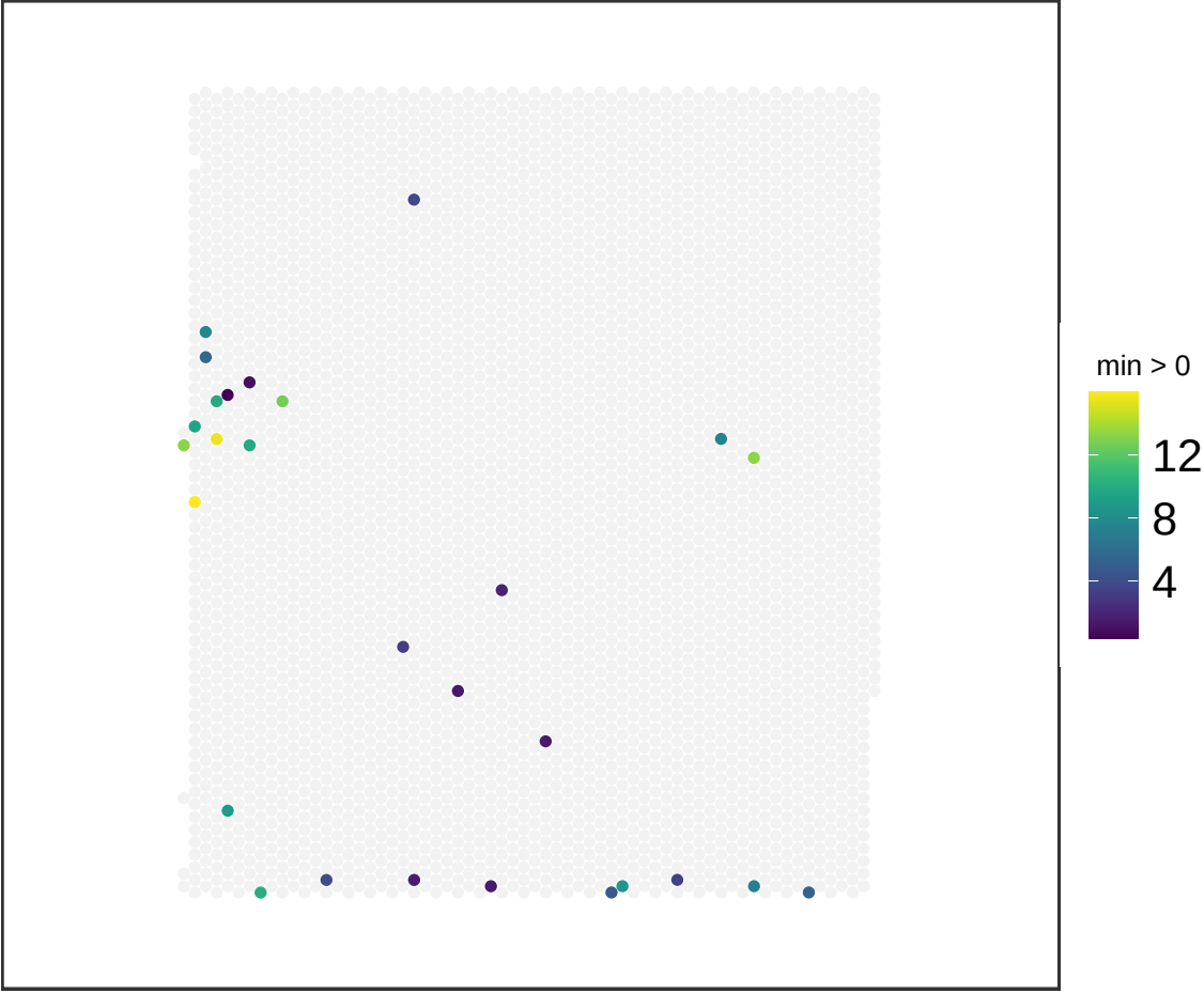
V13M06-388_D1 NMF_61
