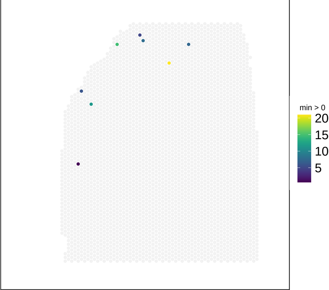
V13M06-388_B1 NMF_61
