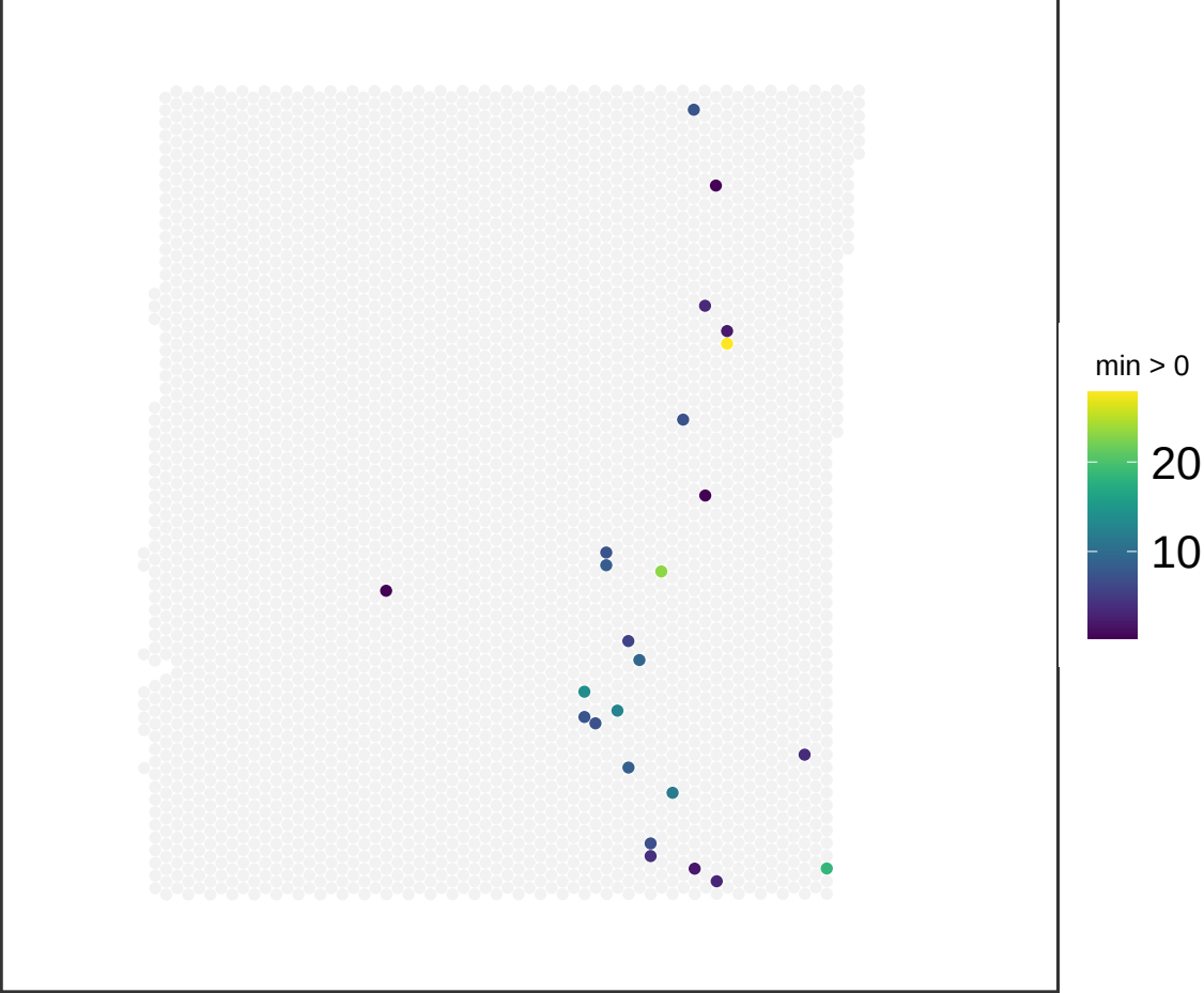
V13M06-388_C1 NMF_61
