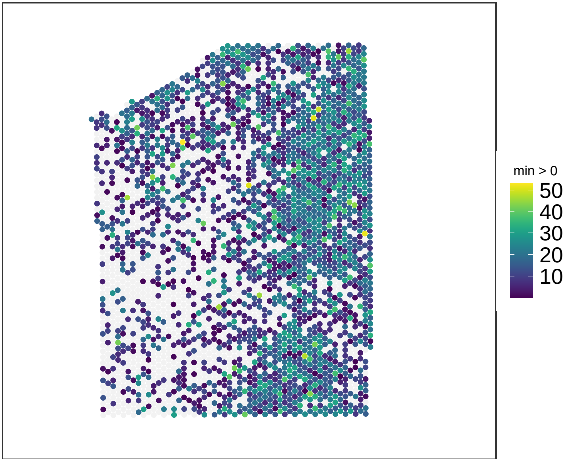
V13M06-387_D1 NMF_70
