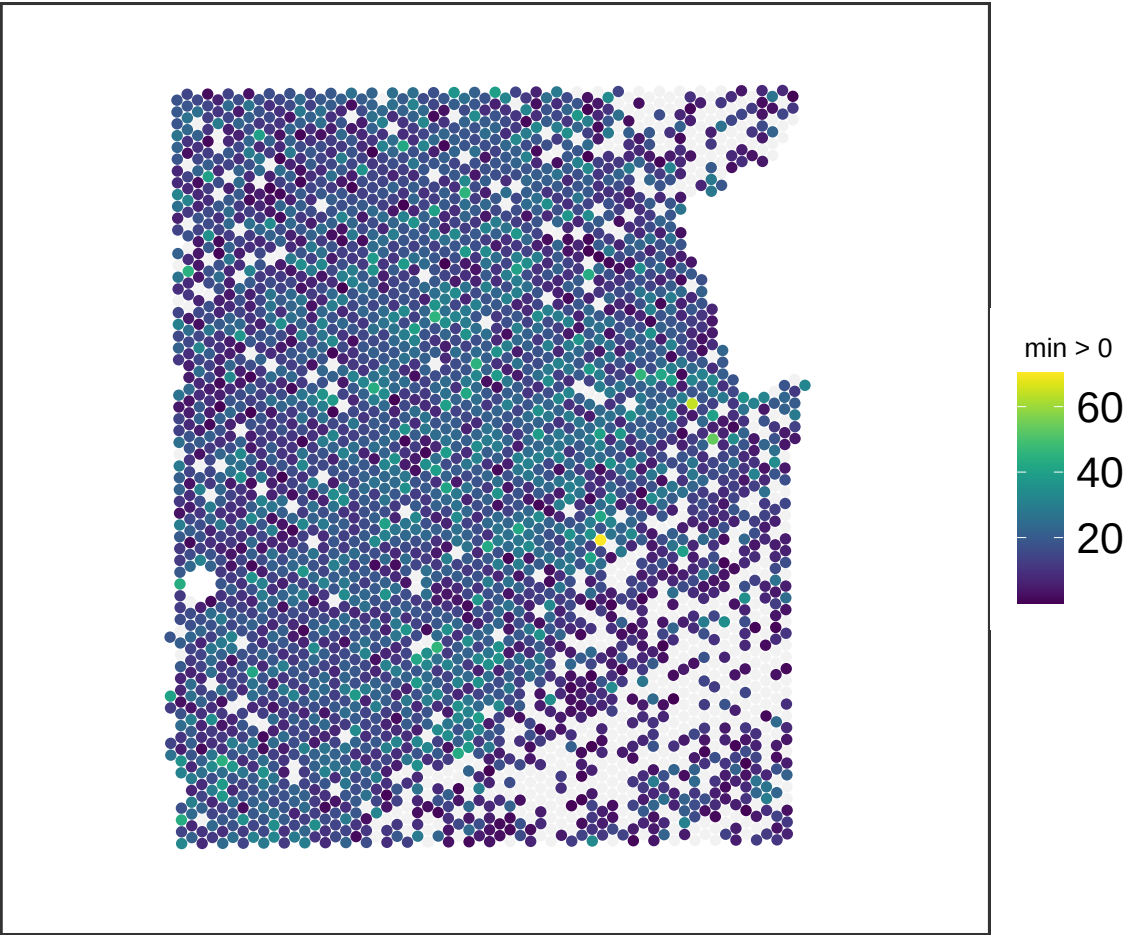
V13M06-387_A1 NMF_70
