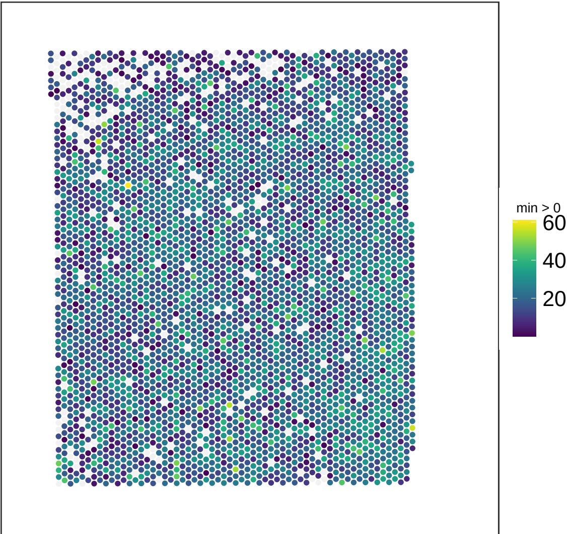
V13M06-387_B1 NMF_70
