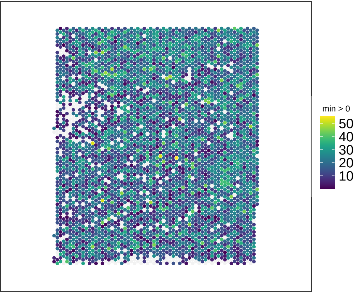
V13M06-388_D1 NMF_70
