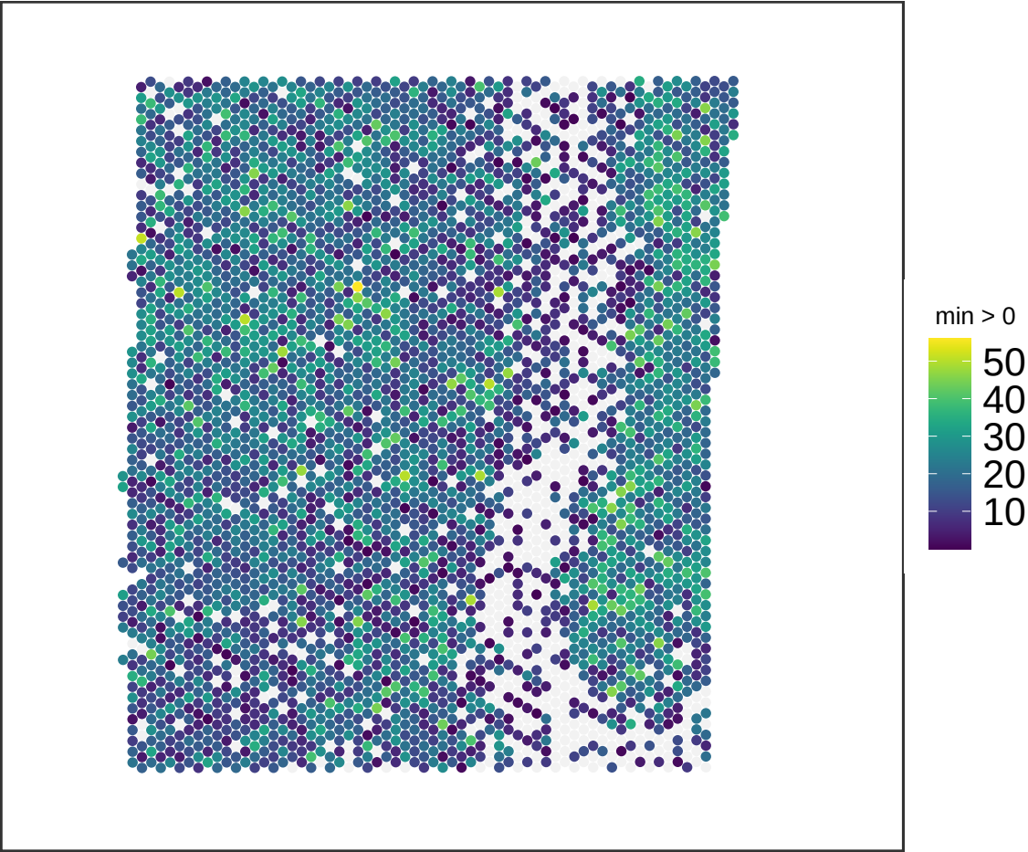
V13M06-388_C1 NMF_70
