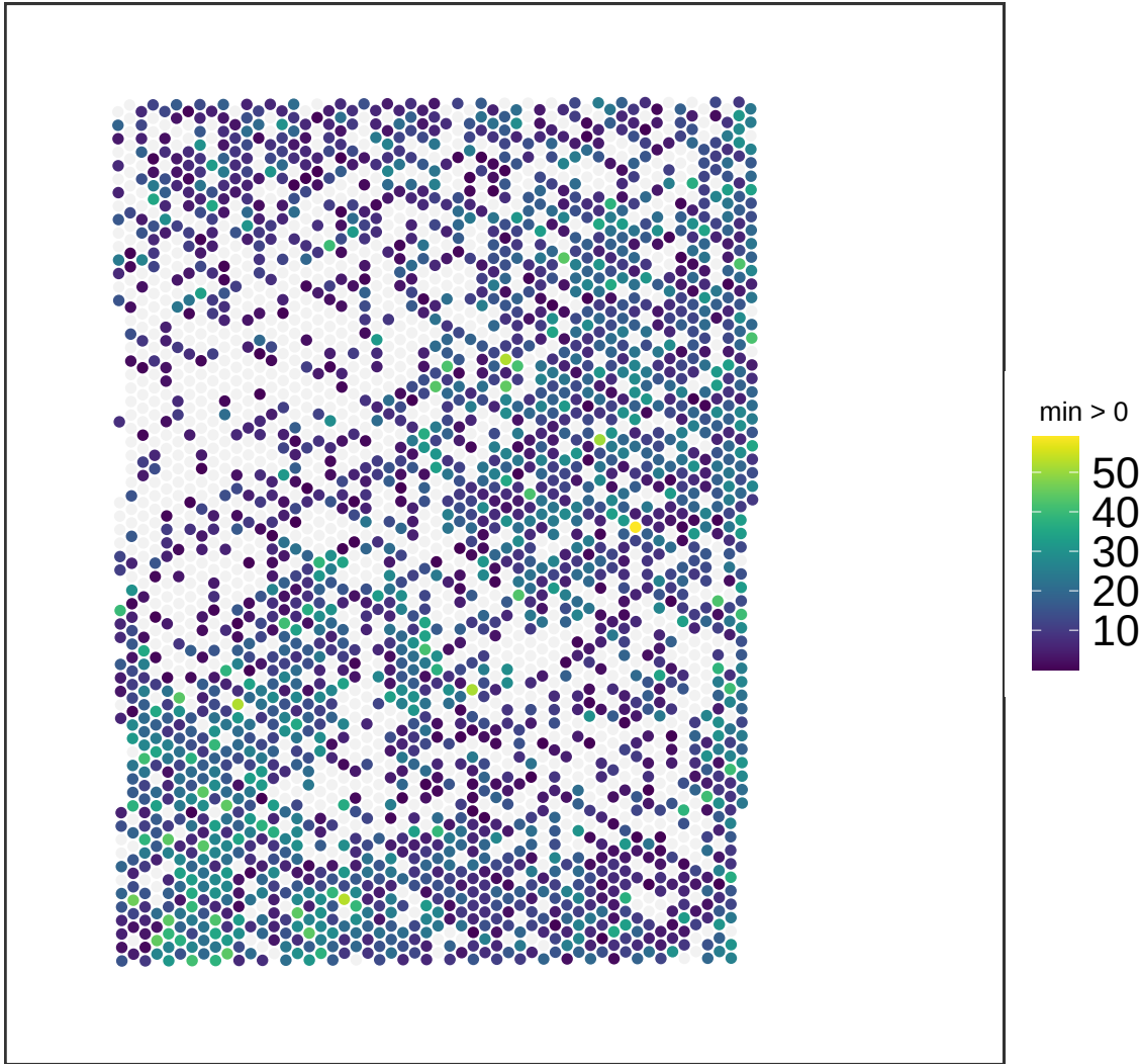
V13M06-387_C1 NMF_70
