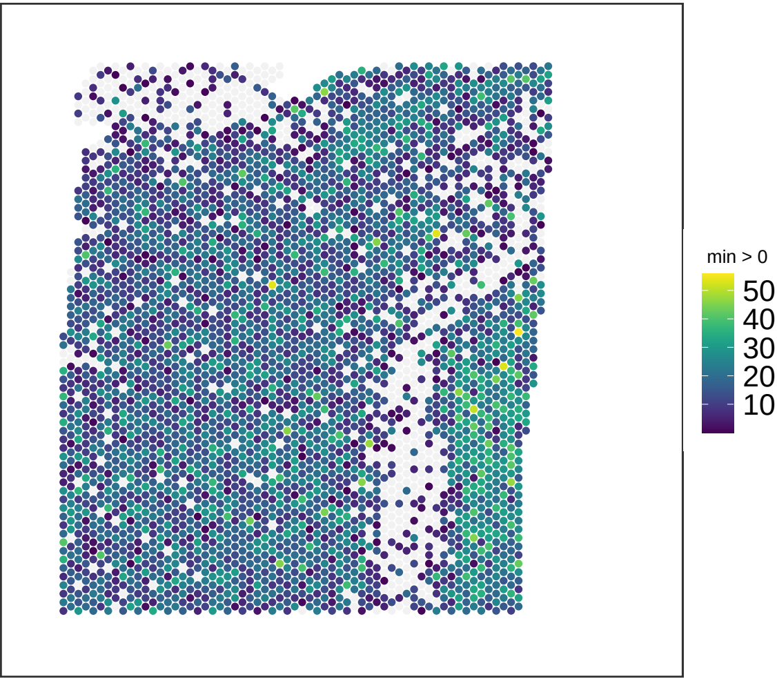
V13M06-388_A1 NMF_70
