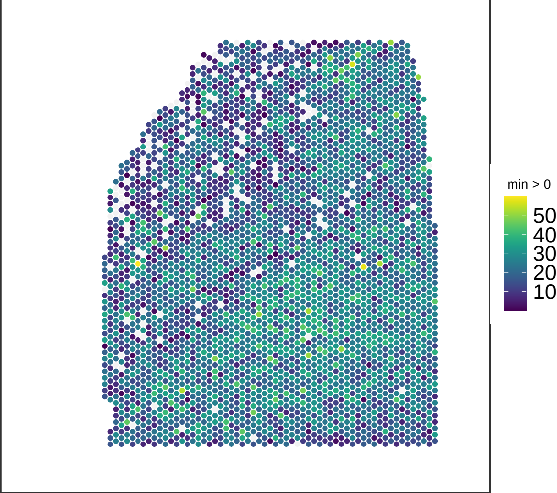
V13M06-388_B1 NMF_70
