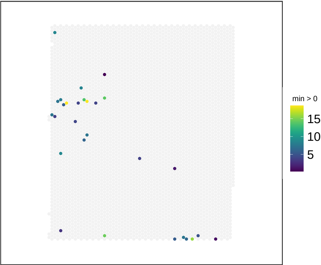
V13M06-388_D1 NMF_9
