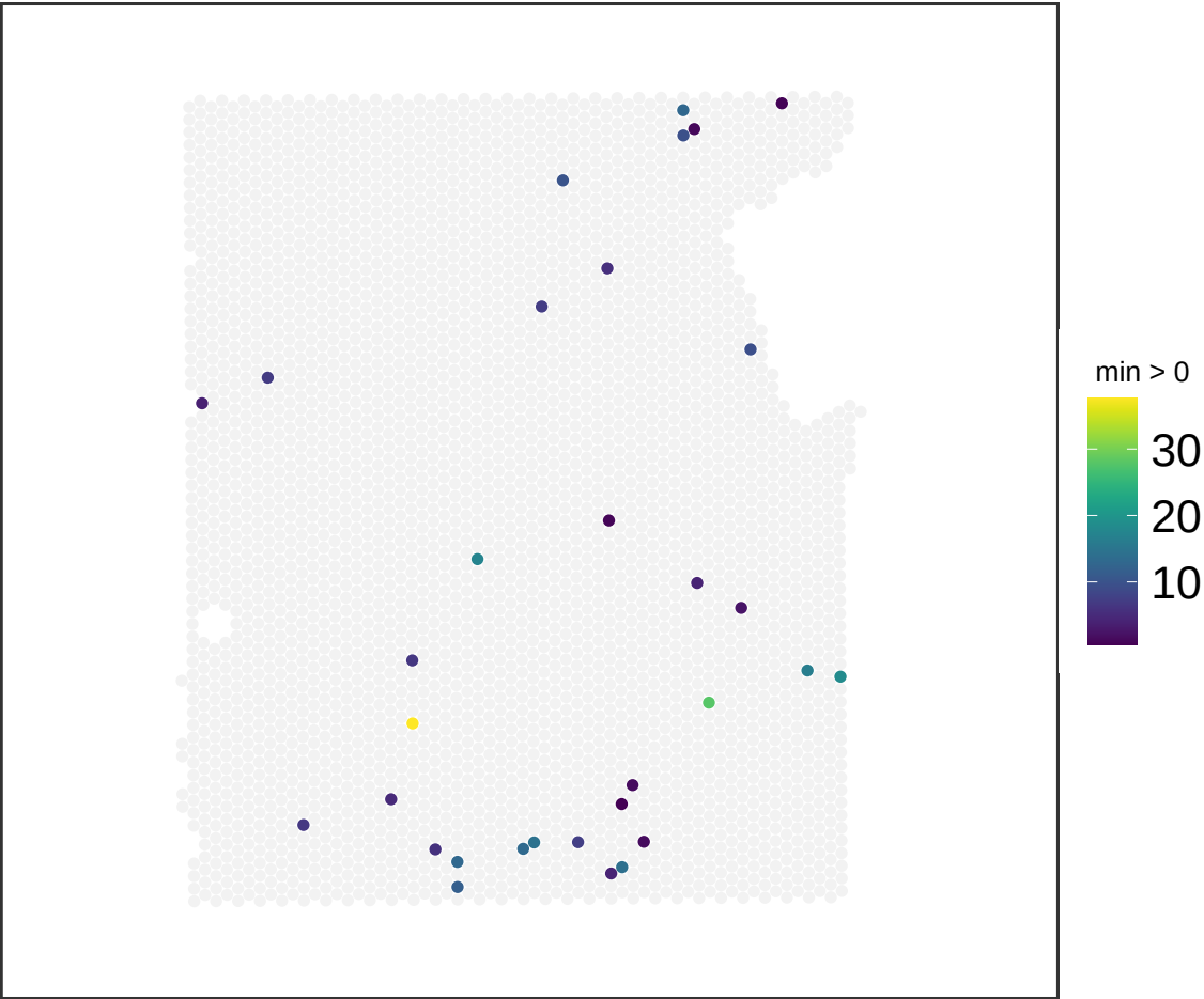
V13M06-387_A1 NMF_9
