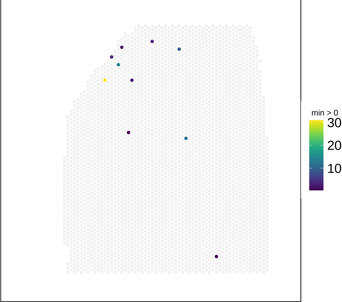
V13M06-388_B1 NMF_9
