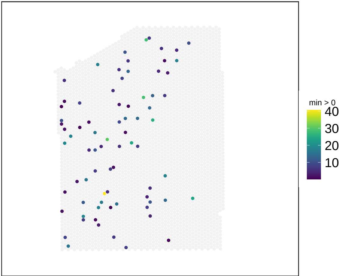
V13M06-387_D1 NMF_9
