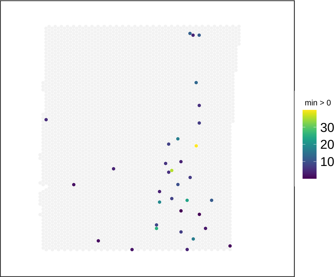
V13M06-388_C1 NMF_9
