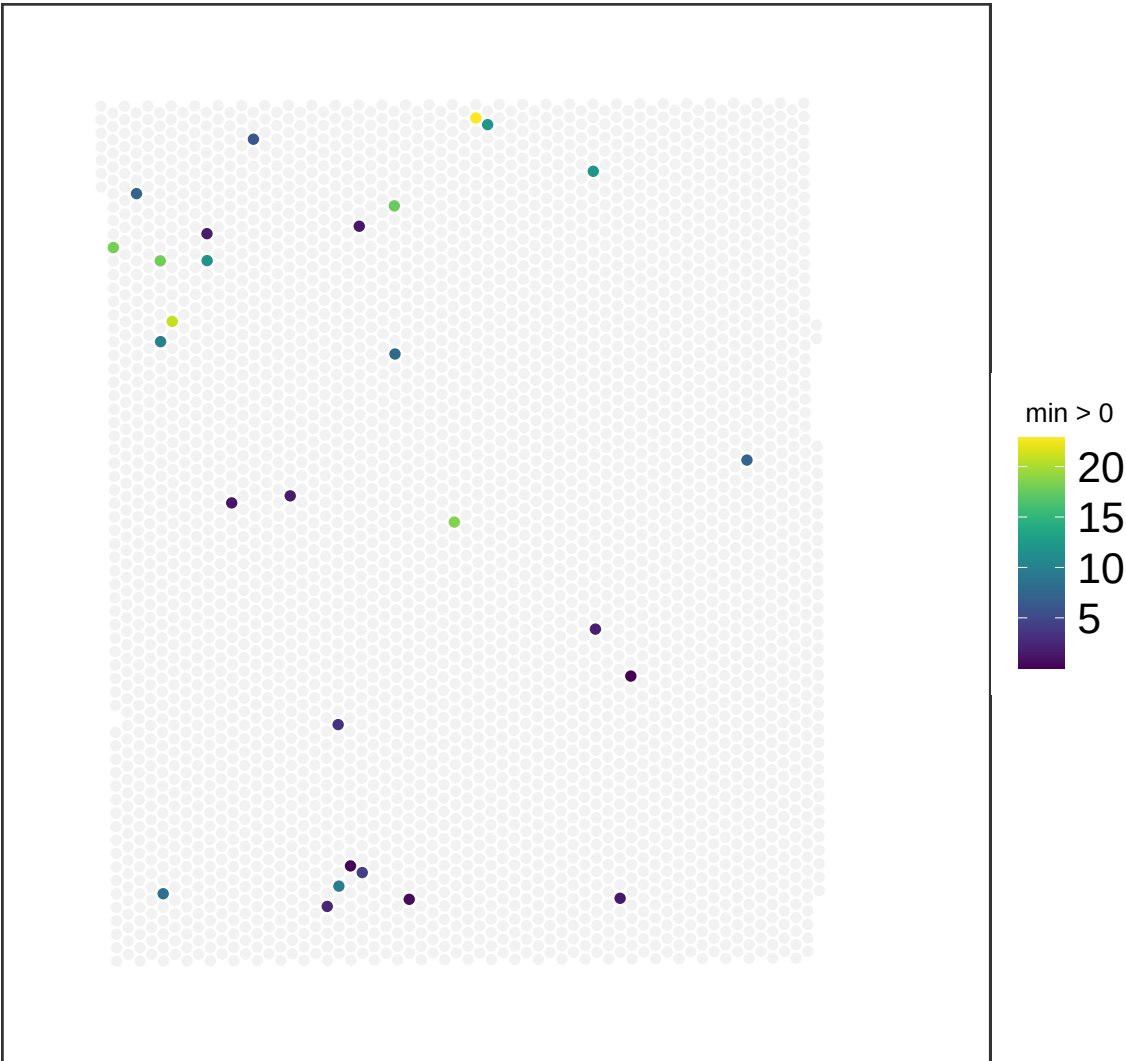
V13M06-387_B1 NMF_9
