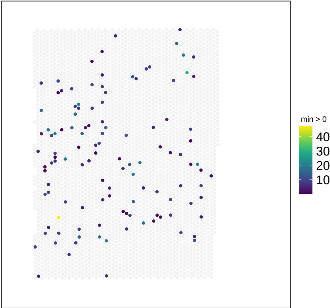
V13M06-387_C1 NMF_9
