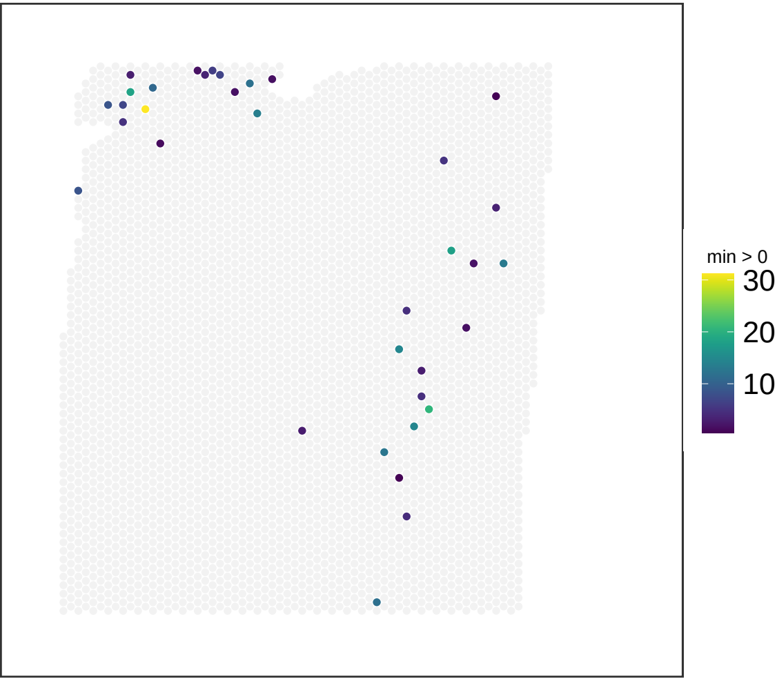
V13M06-388_A1 NMF_9
