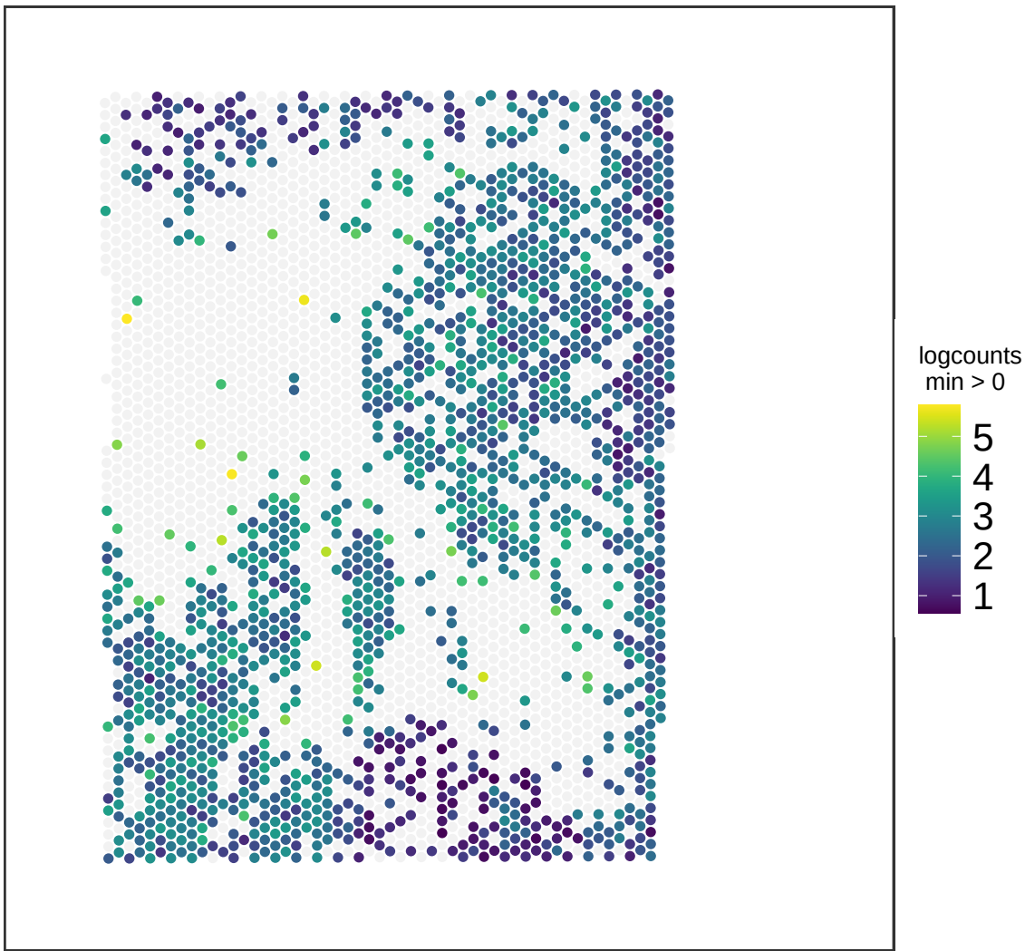
V13M06-387_C1 BASP1
