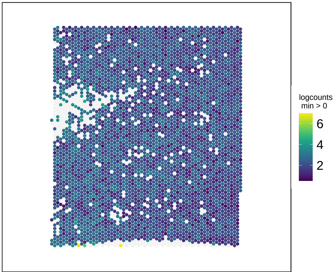
V13M06-388_D1 BASP1
