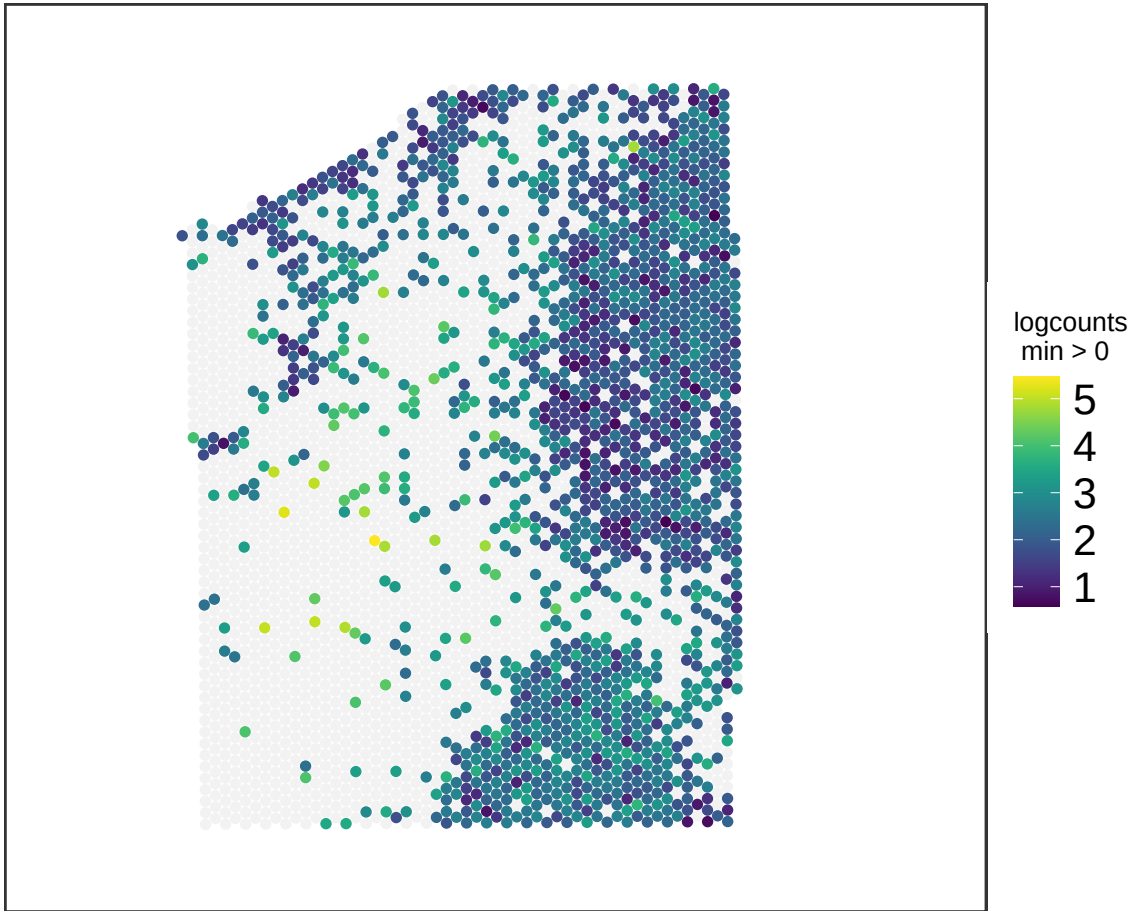
V13M06-387_D1 BASP1
