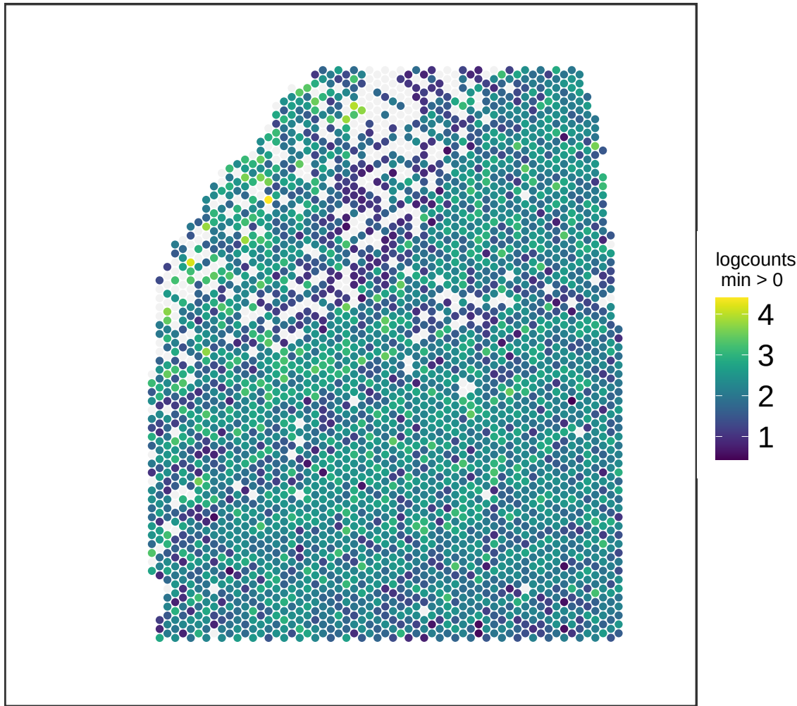
V13M06-388_B1 BASP1
