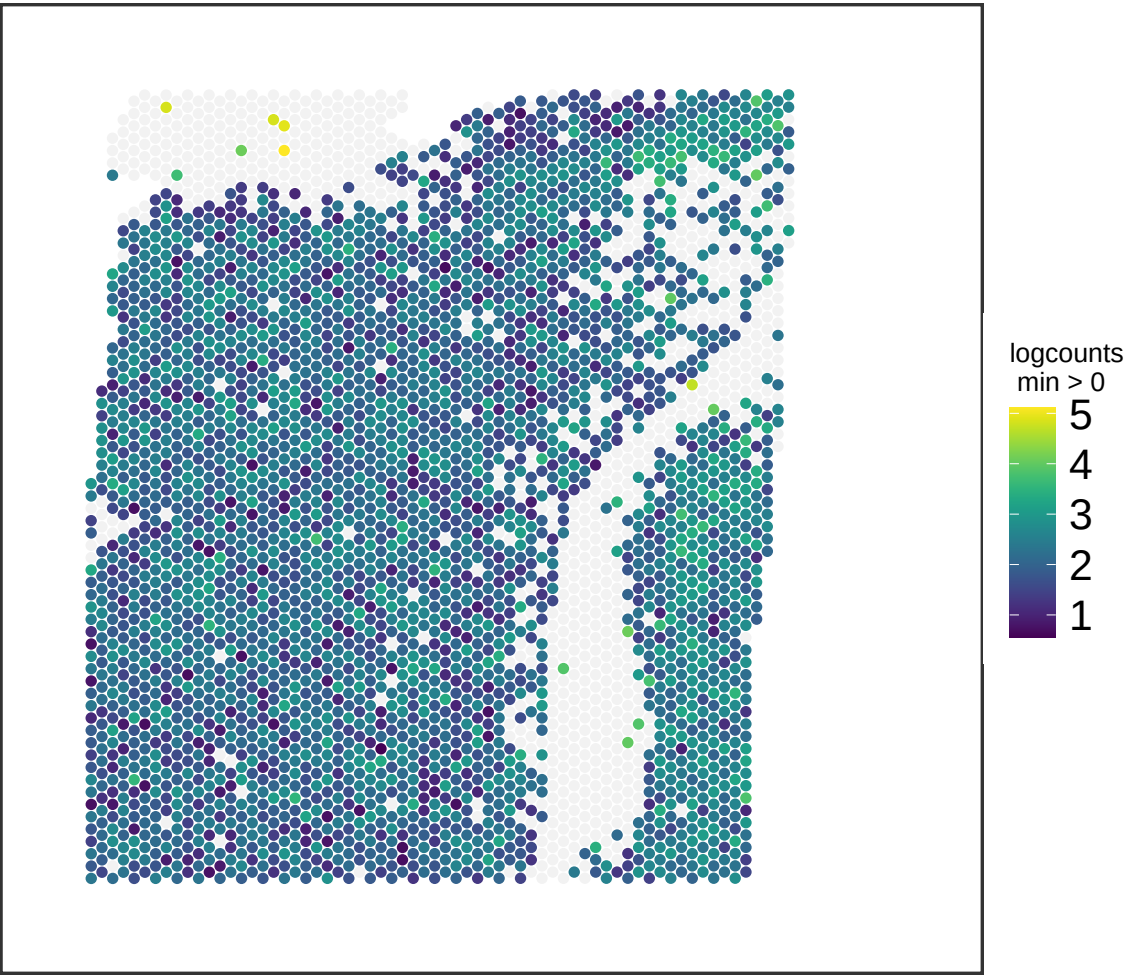
V13M06-388_A1 BASP1
