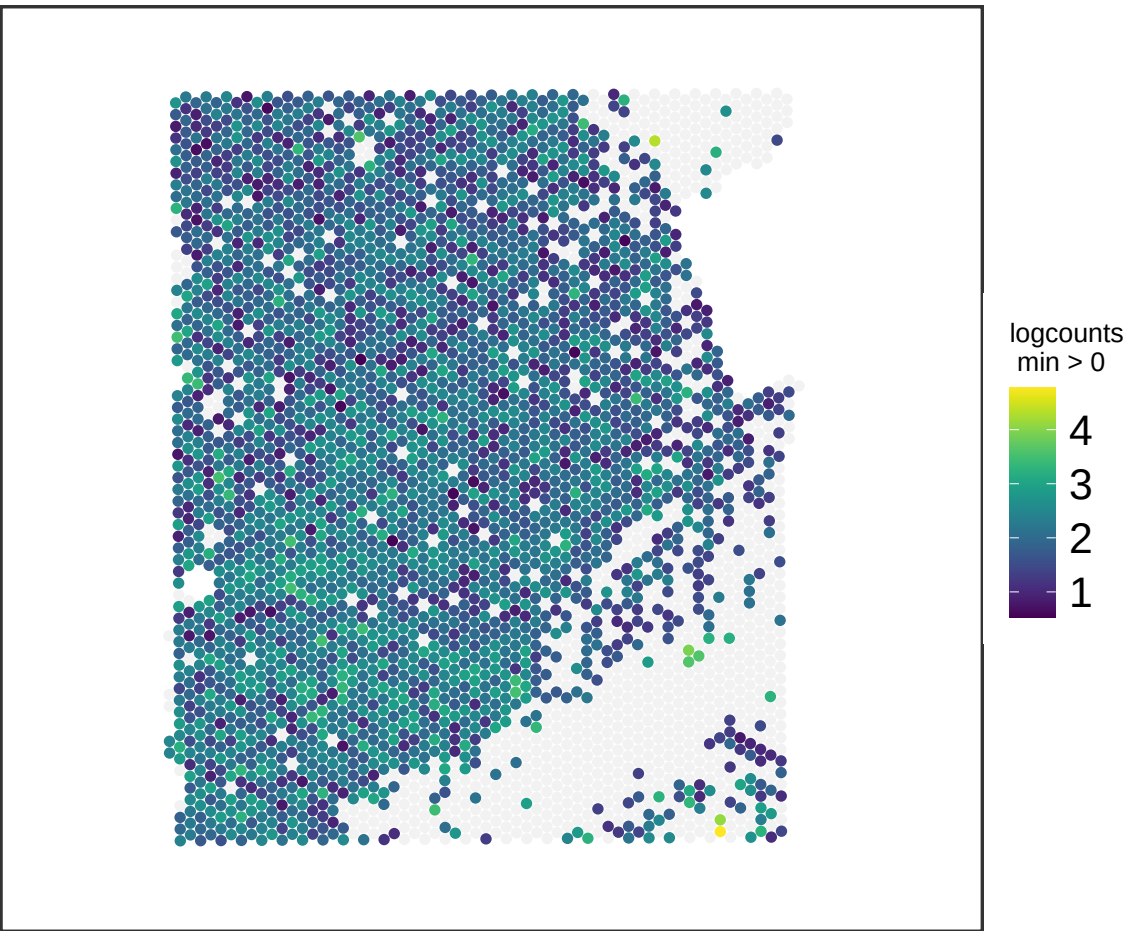
V13M06-387_A1 BASP1
