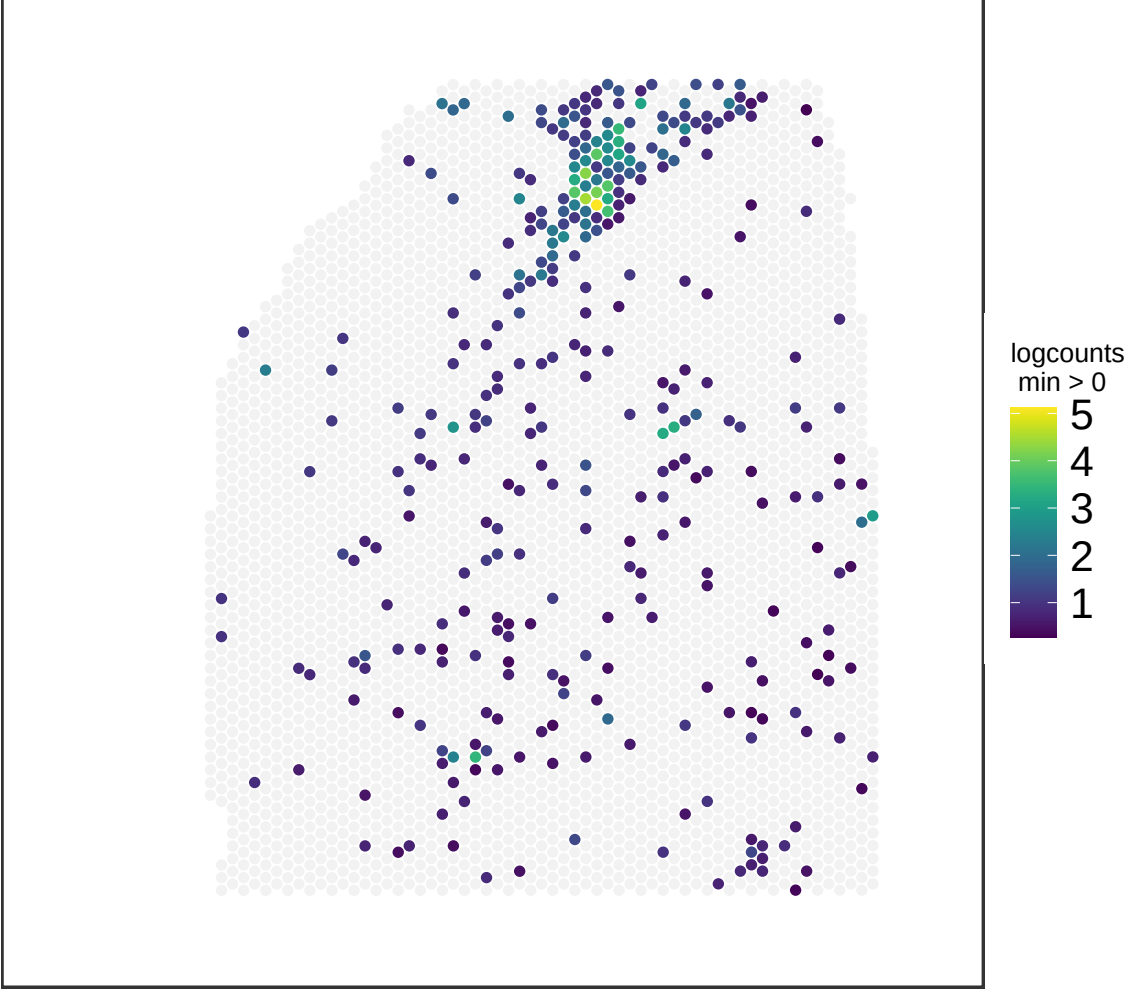
V13M06-388_B1 ACTA2
