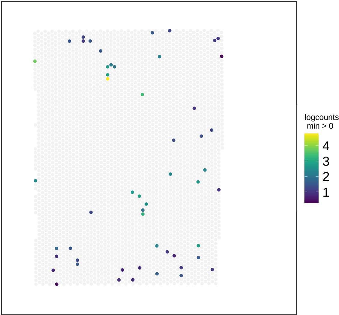
V13M06-387_C1 ACTA2
