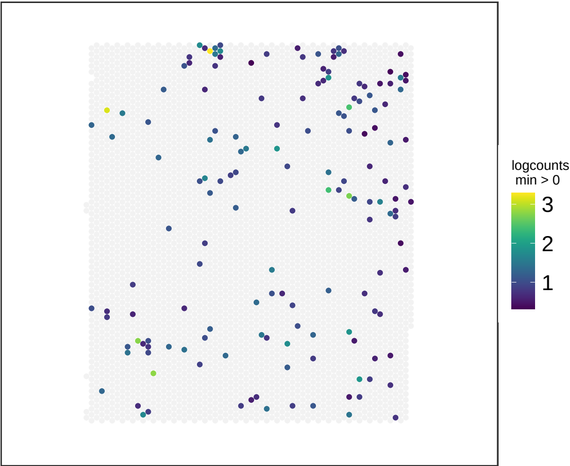
V13M06-388_D1 ACTA2
