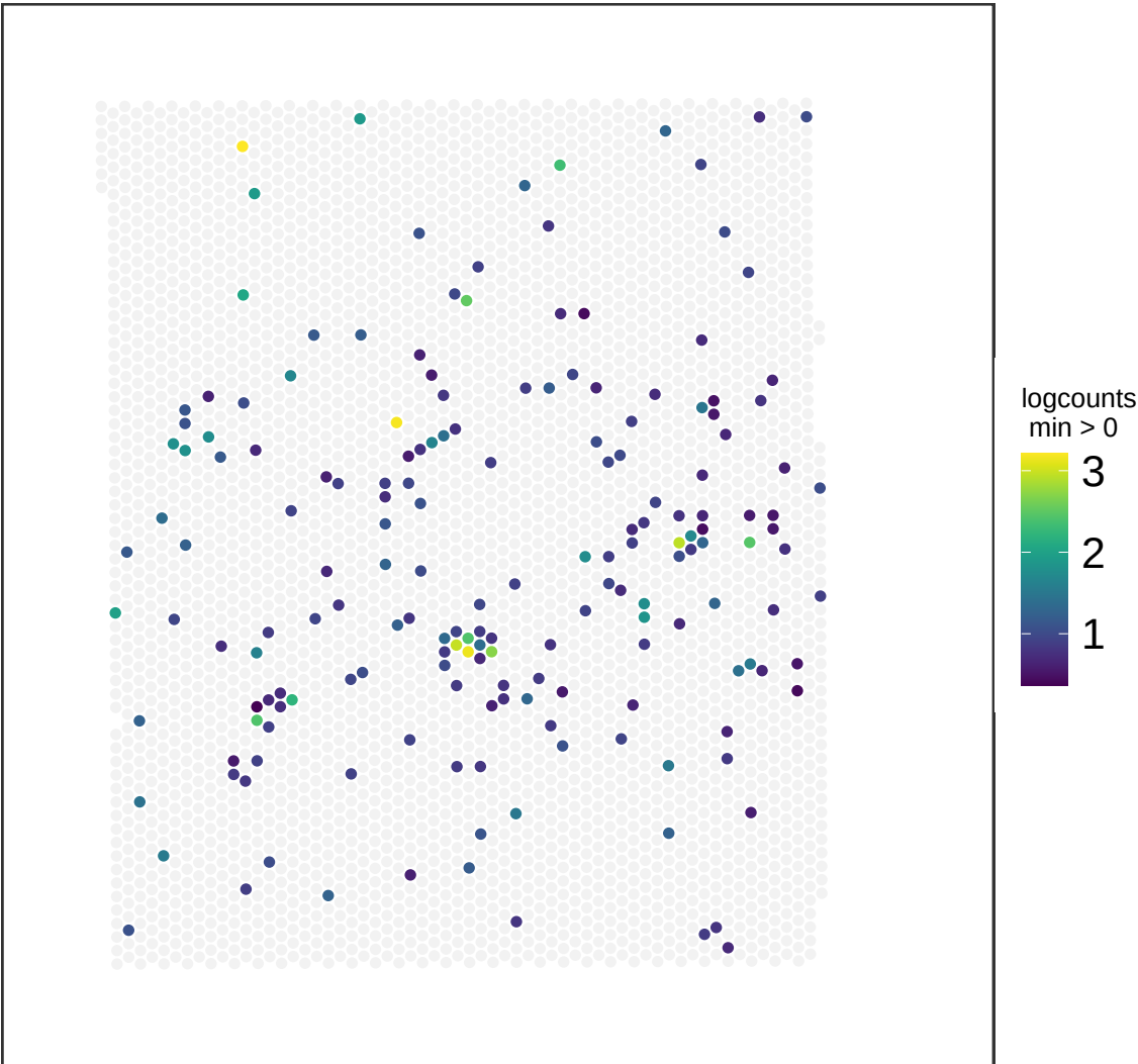
V13M06-387_B1 ACTA2
