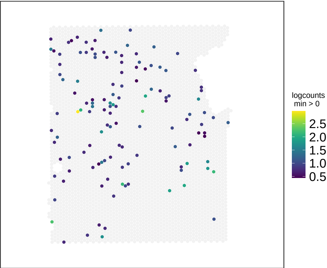
V13M06-387_A1 ACTA2
