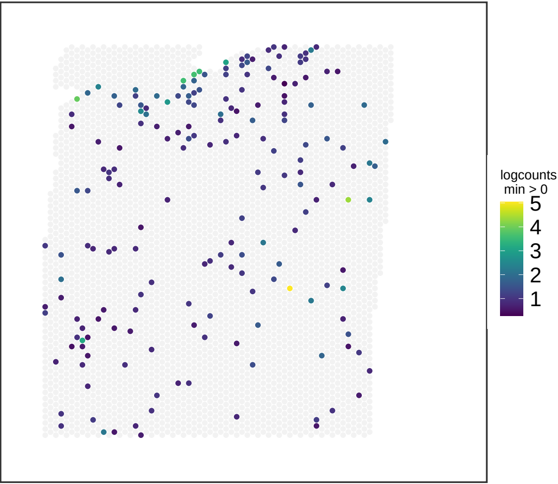
V13M06-388_A1 ACTA2
