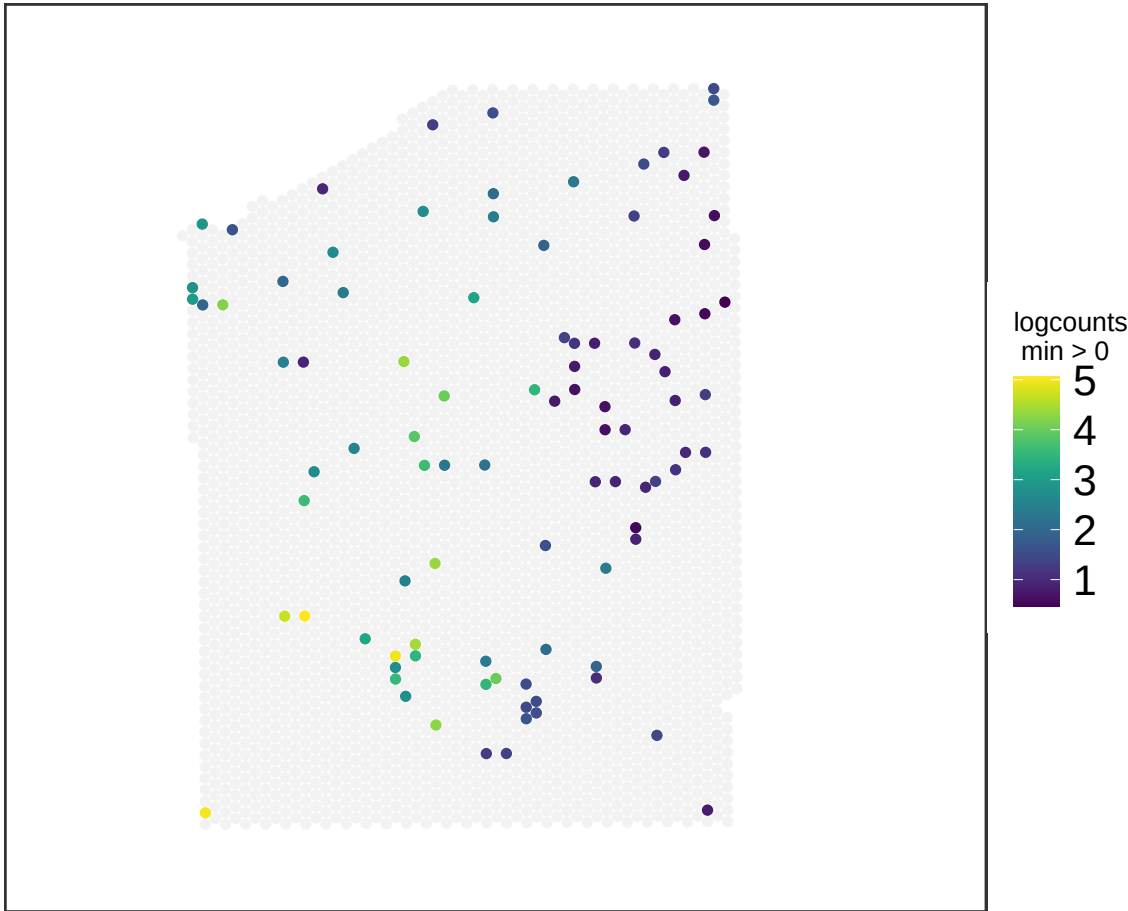
V13M06-387_D1 ACTA2
