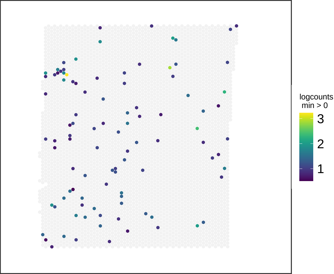
V13M06-388_C1 ACTA2
