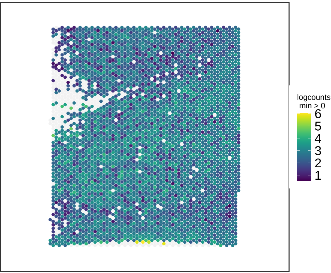
V13M06-388_D1 SLC17A7
