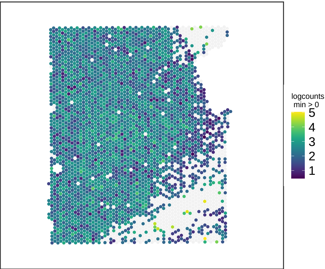
V13M06-387_A1 SLC17A7
