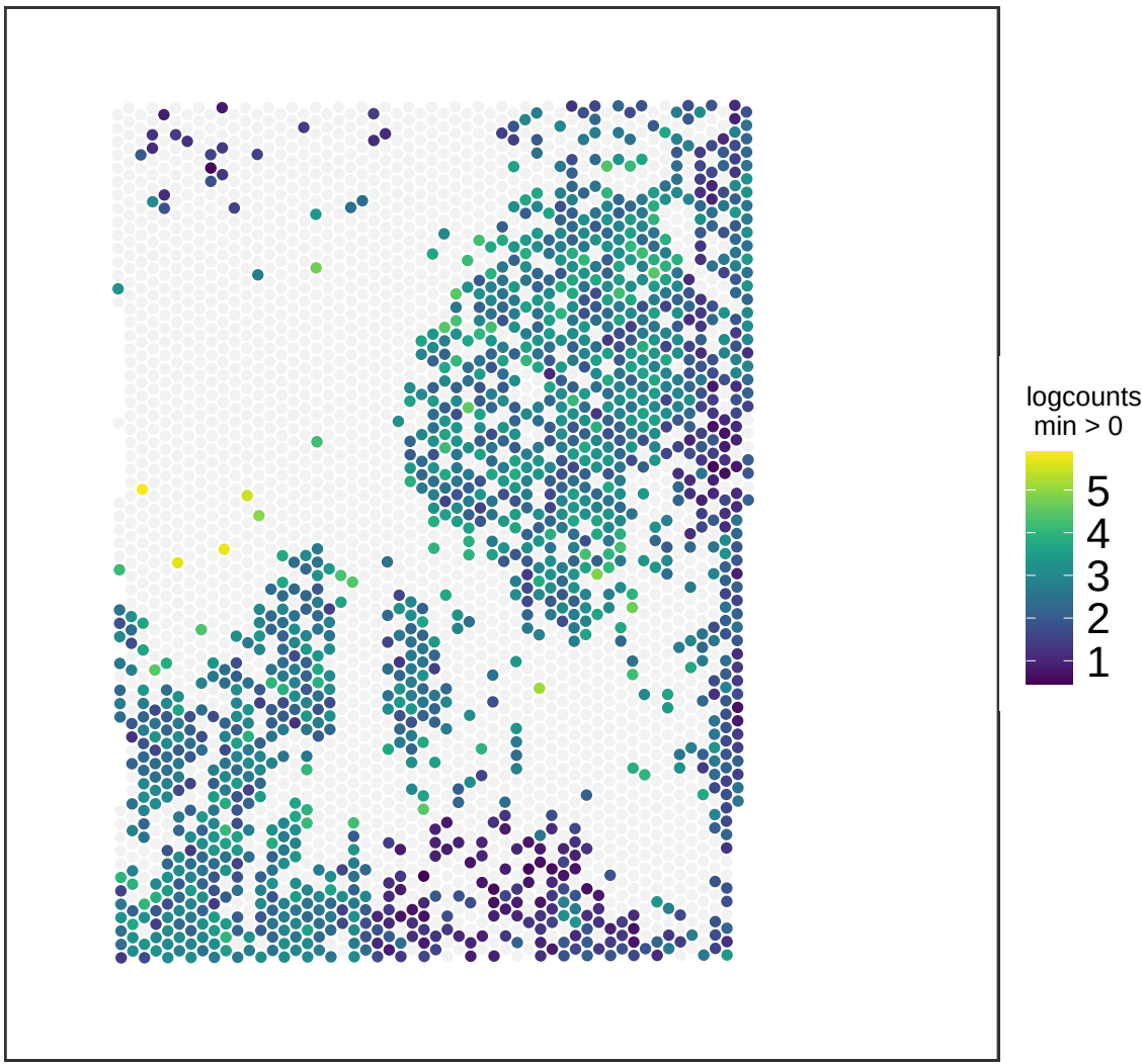
V13M06-387_C1 SLC17A7
