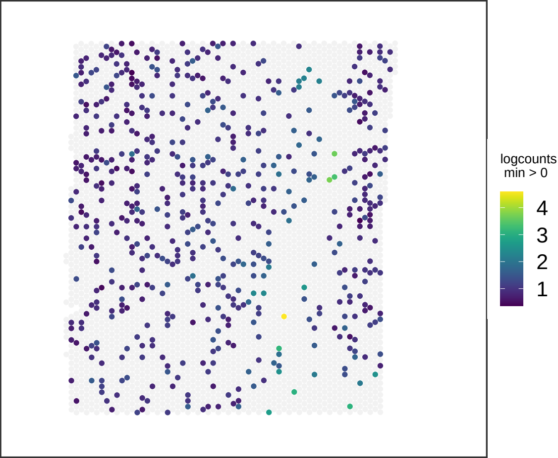
V13M06-388_C1 PLXDC2
