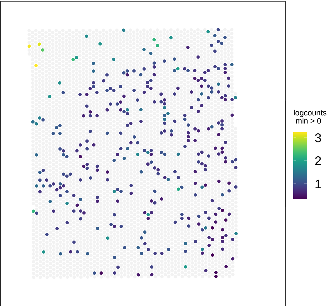
V13M06-387_B1 PLXDC2
