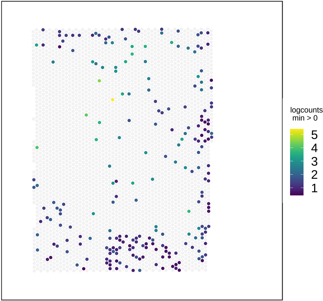
V13M06-387_C1 PLXDC2
