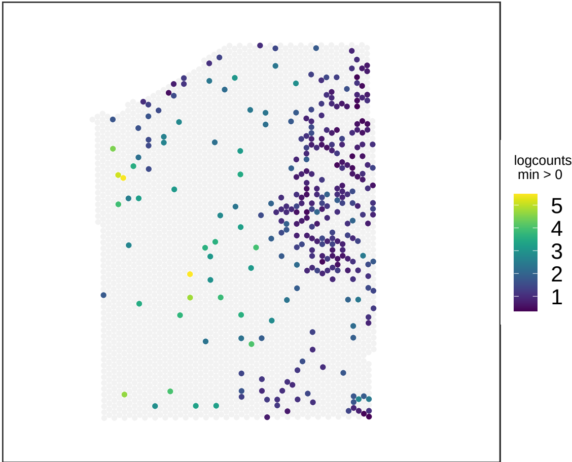
V13M06-387_D1 PLXDC2
