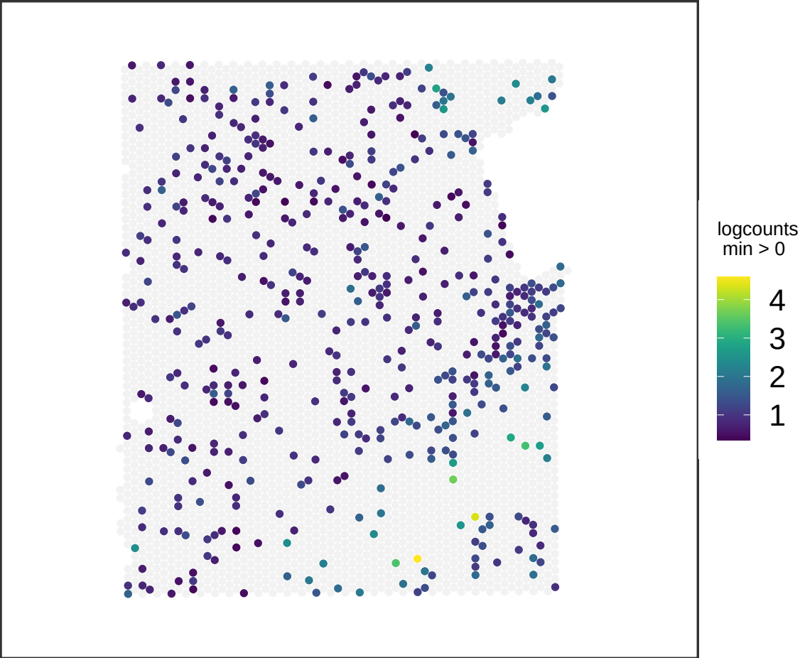
V13M06-387_A1 PLXDC2
