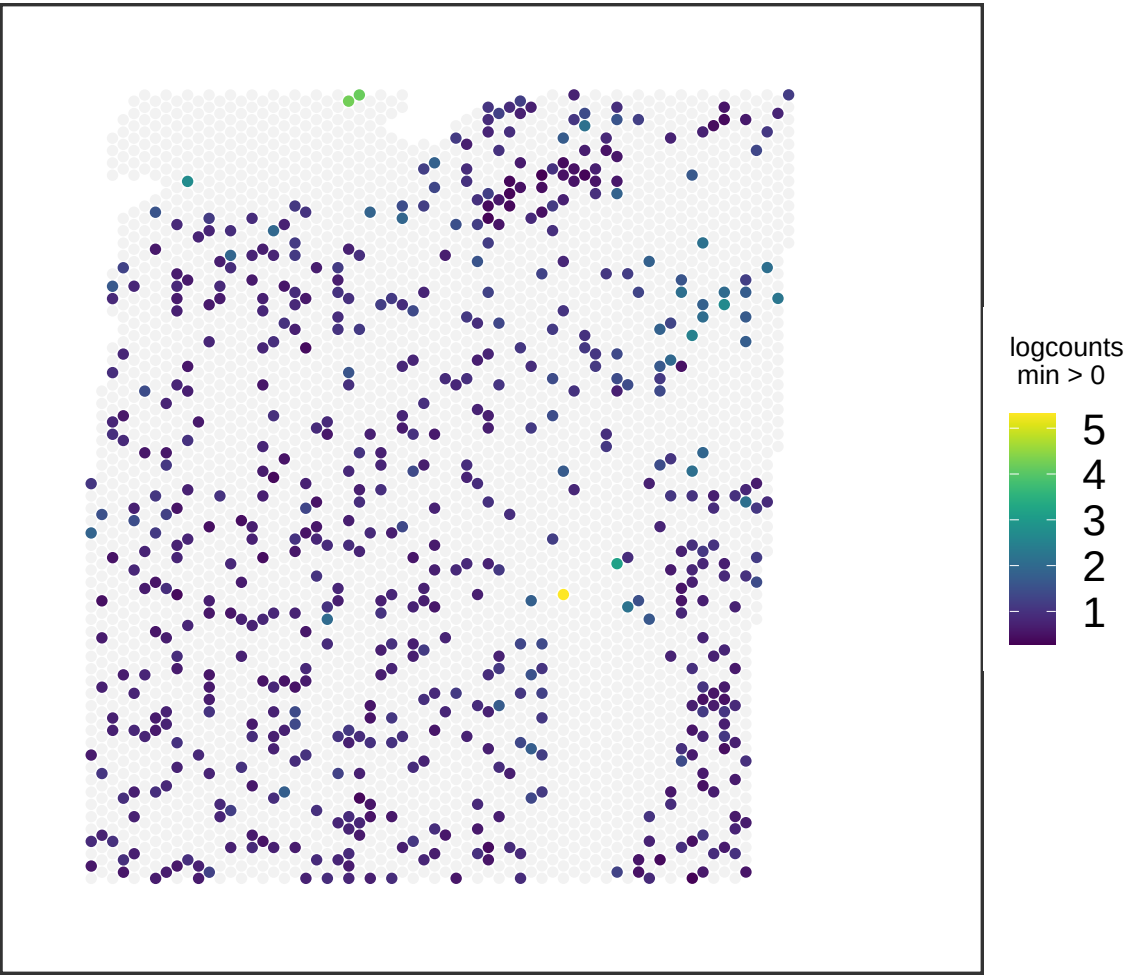
V13M06-388_A1 PLXDC2
