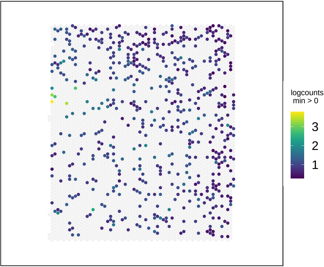
V13M06-388_D1 PLXDC2
