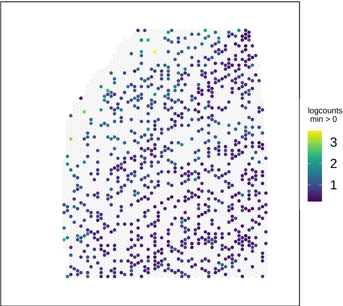
V13M06-388_B1 PLXDC2
