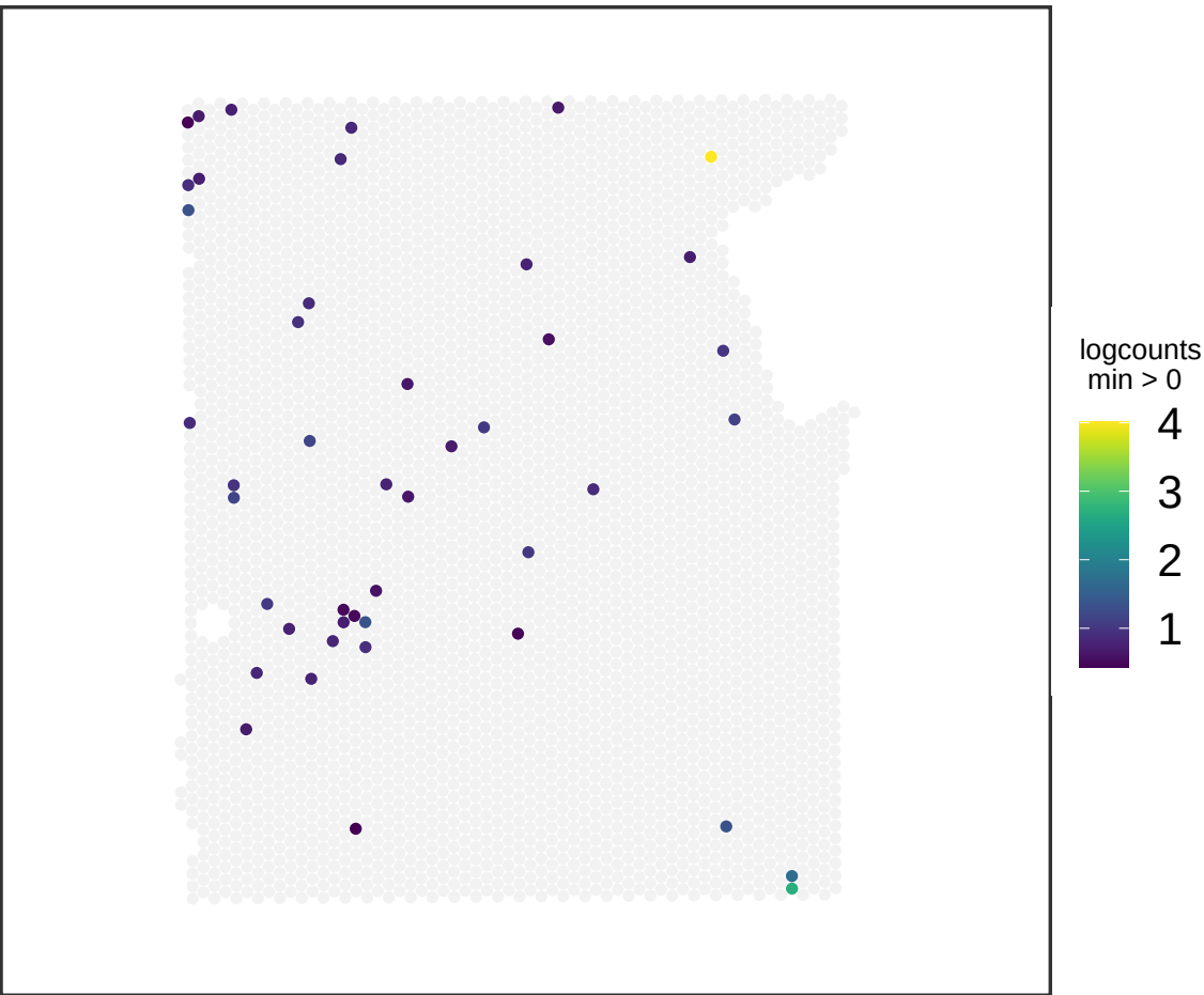
V13M06-387_A1 ZNF385B
