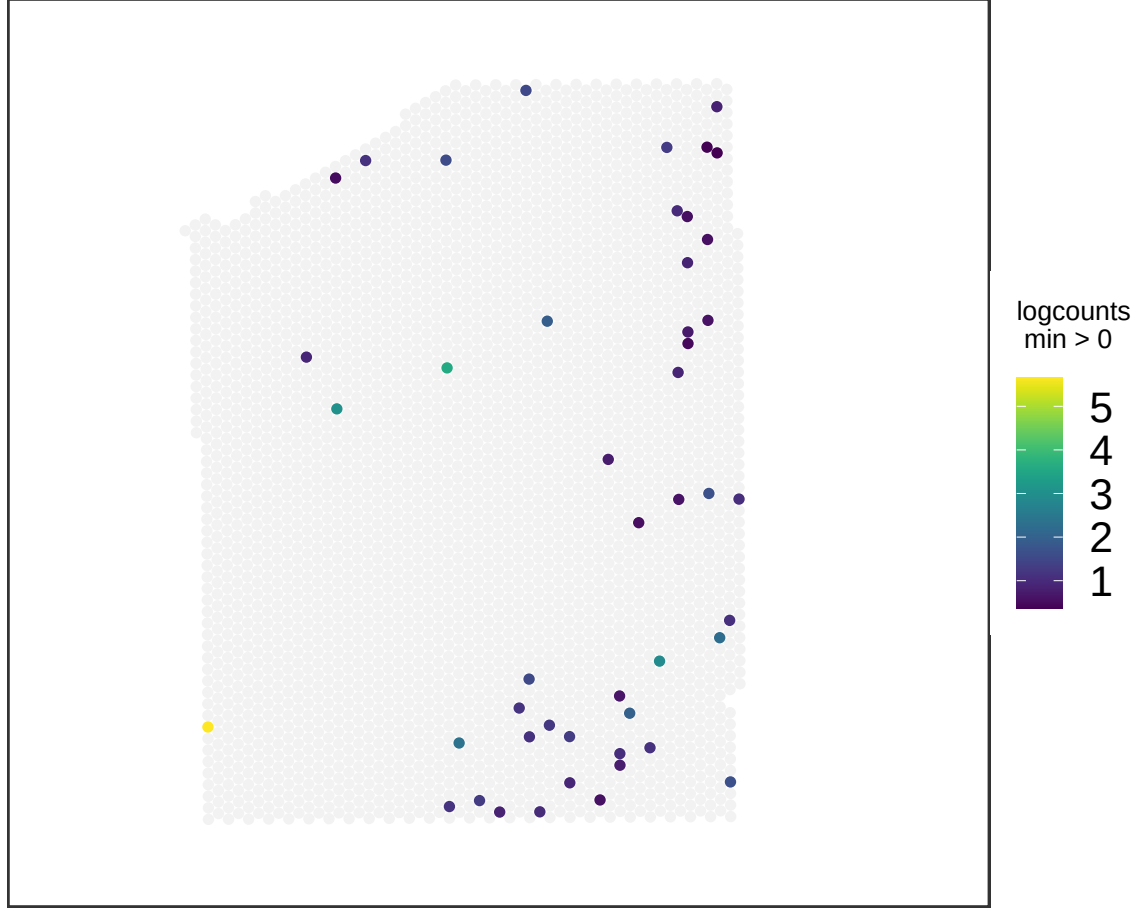
V13M06-387_D1 ZNF385B
