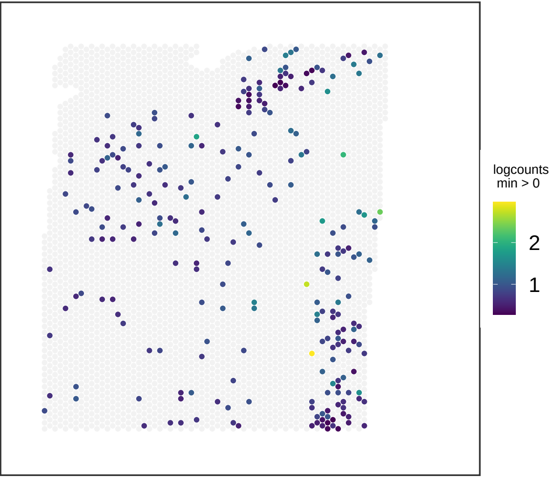
V13M06-388_A1 ZNF385B
