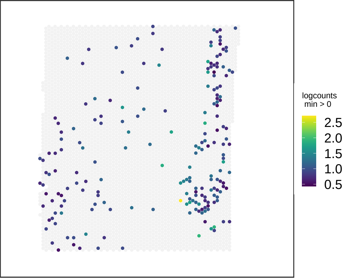
V13M06-388_C1 ZNF385B
