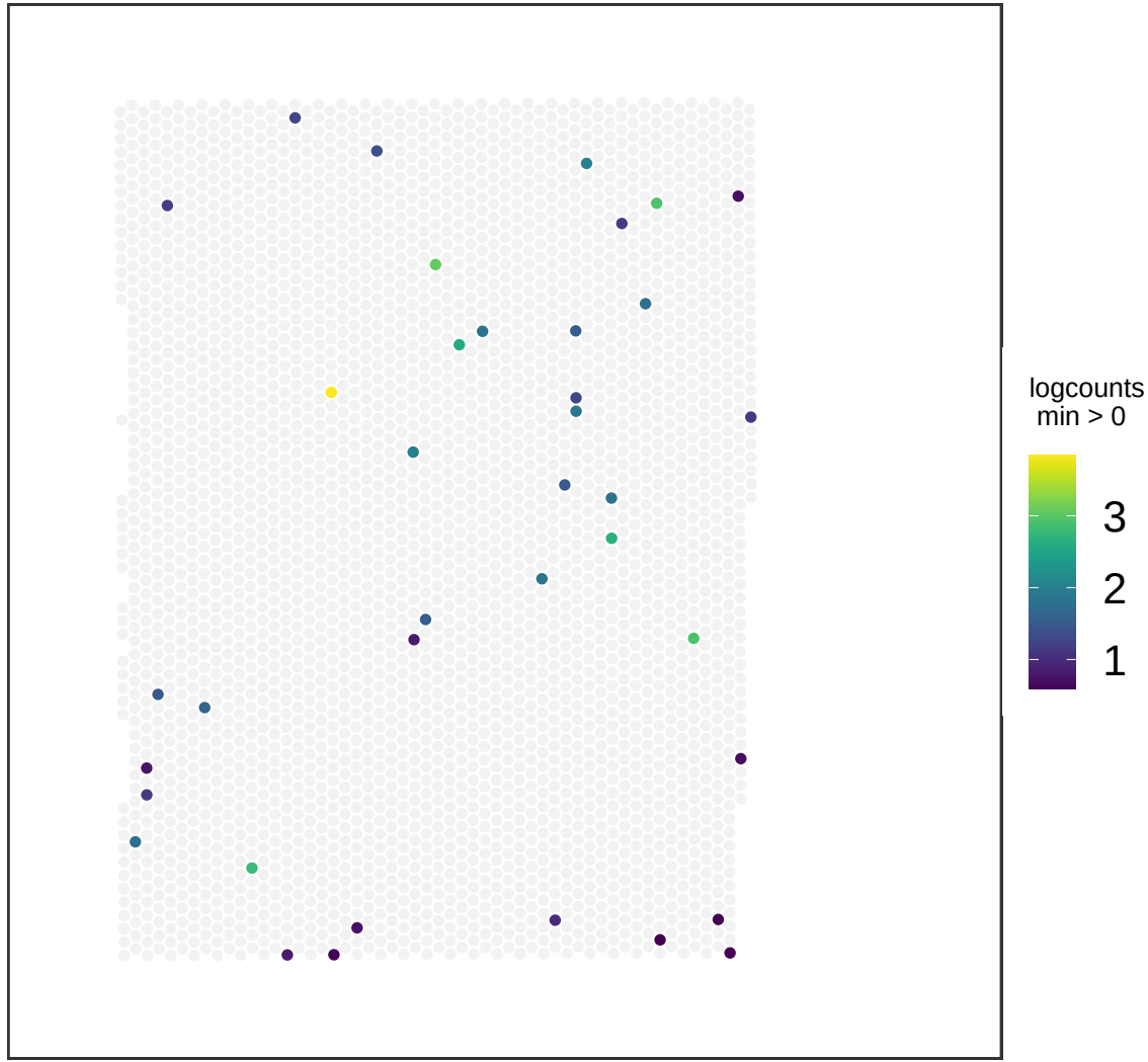
V13M06-387_C1 ZNF385B
