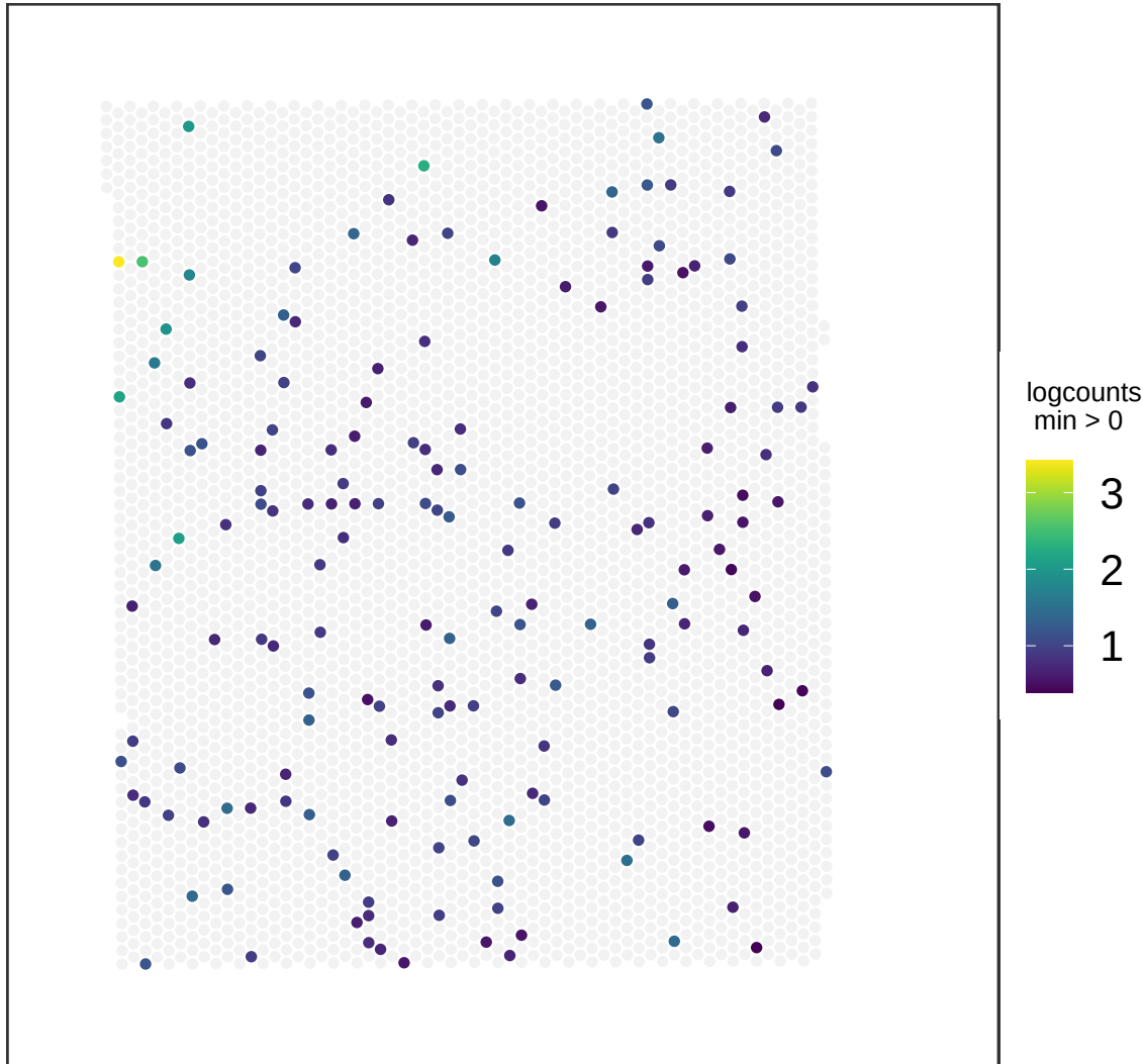
V13M06-387_B1 ZNF385B
