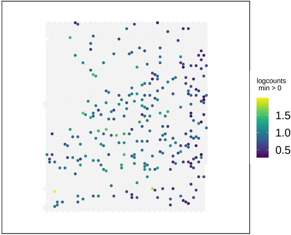
V13M06-388_D1 ZNF385B
