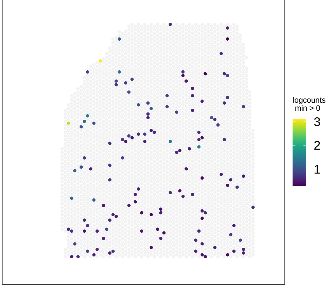
V13M06-388_B1 ZNF385B
