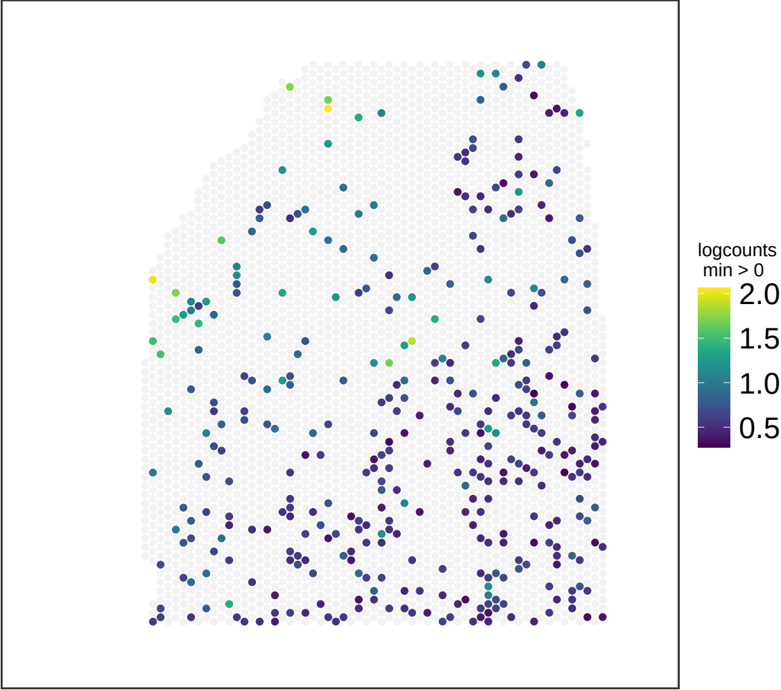
V13M06-388_B1 TMEM132C
