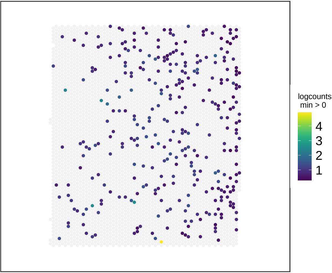
V13M06-388_D1 TMEM132C
