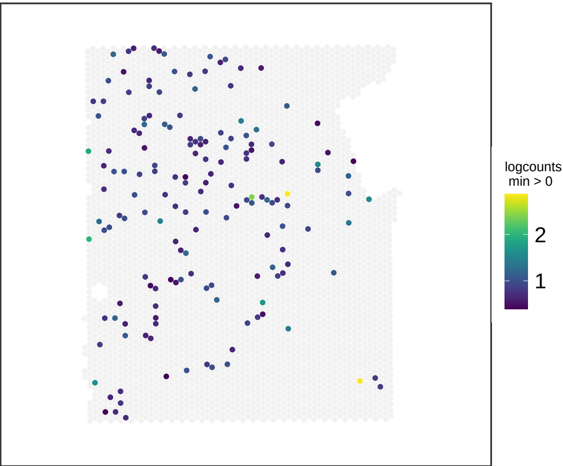
V13M06-387_A1 TMEM132C
