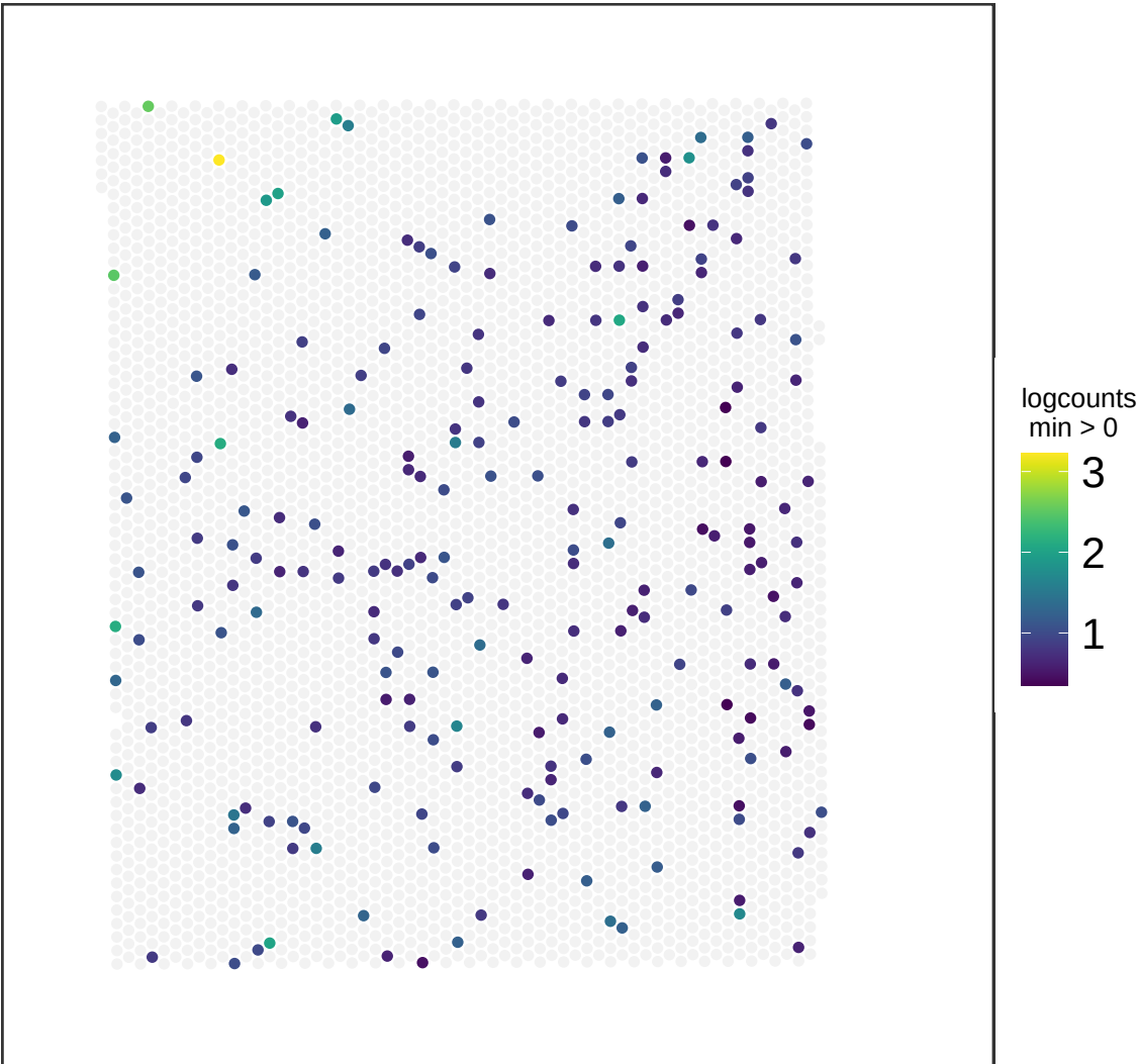
V13M06-387_B1 TMEM132C
