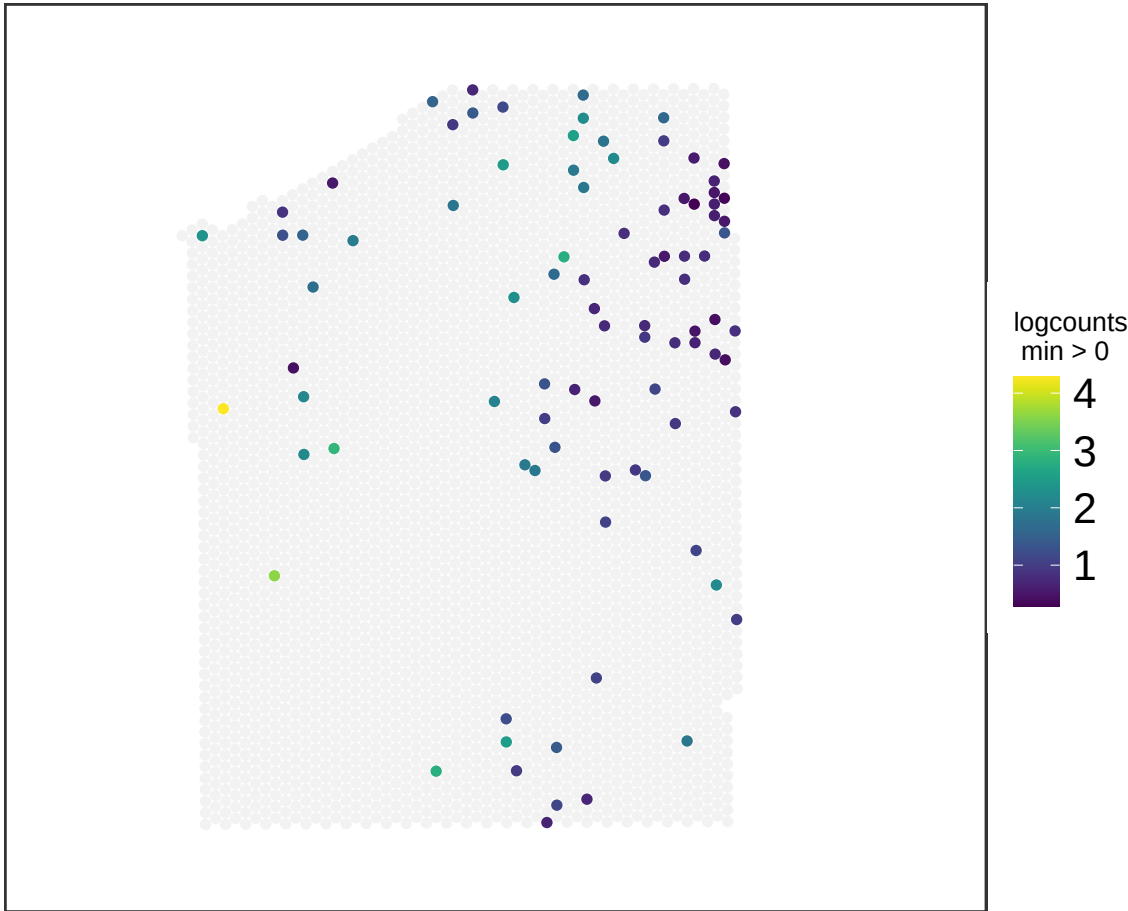
V13M06-387_D1 TMEM132C
