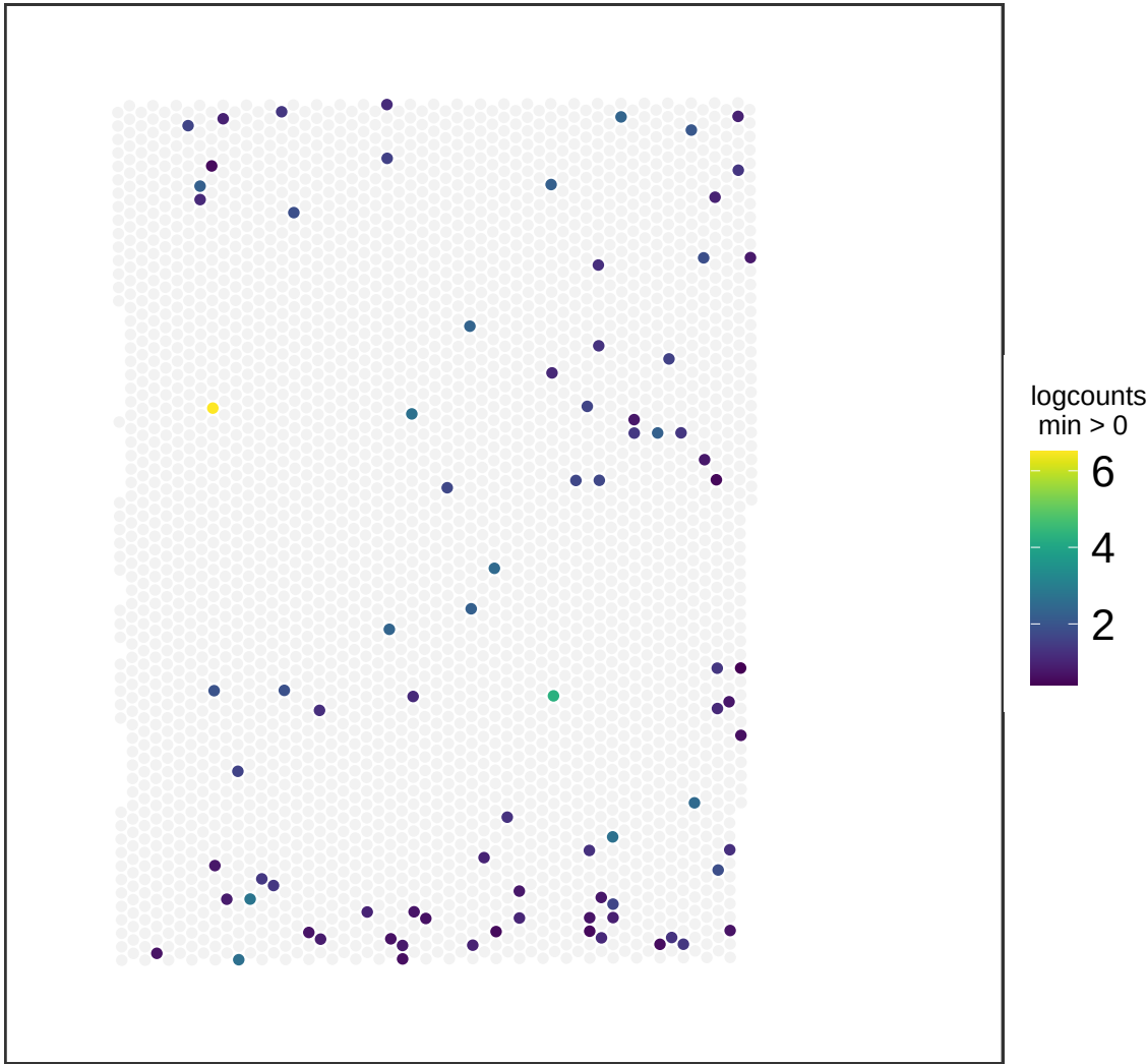
V13M06-387_C1 TMEM132C
