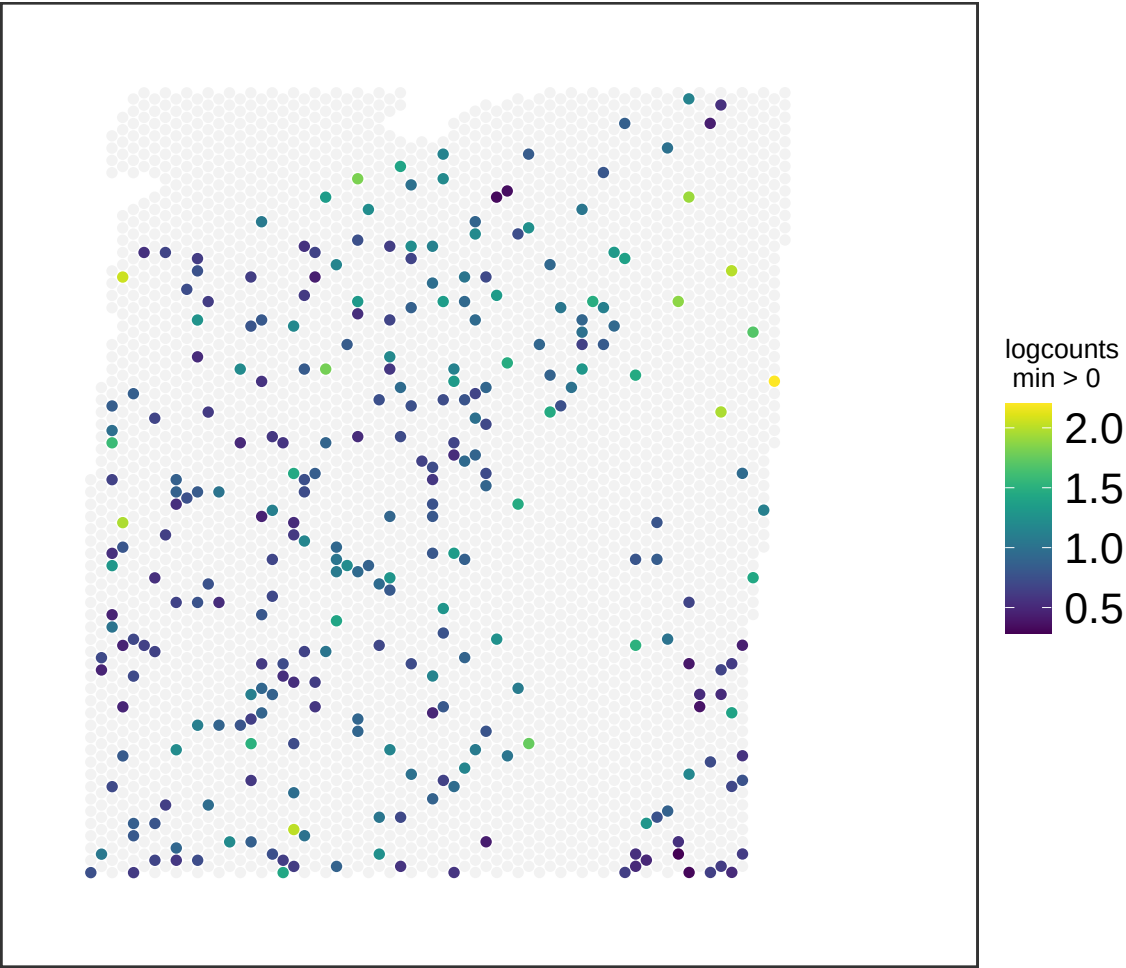
V13M06-388_A1 TMEM132C
