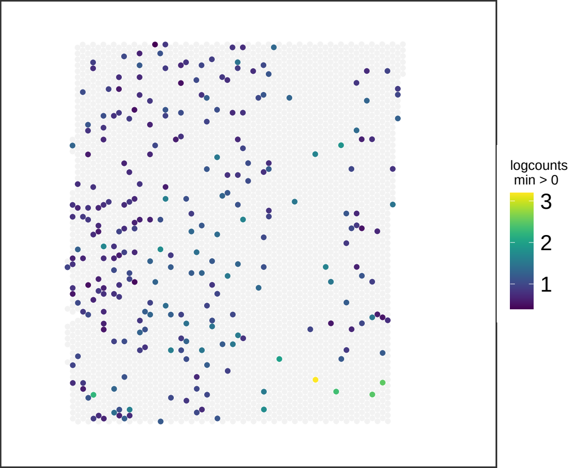
V13M06-388_C1 TMEM132C
