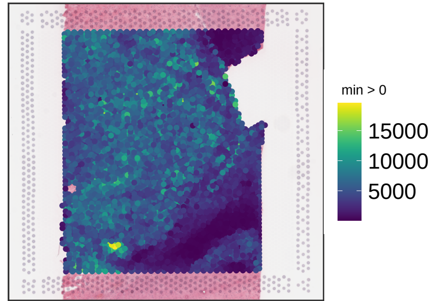
V13M06-387_A1 sum_umi
