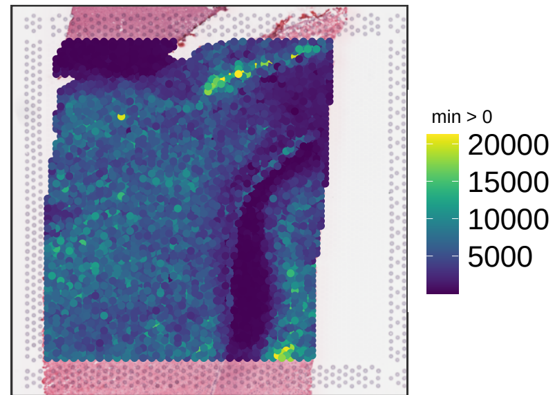
V13M06-388_A1 sum_umi
