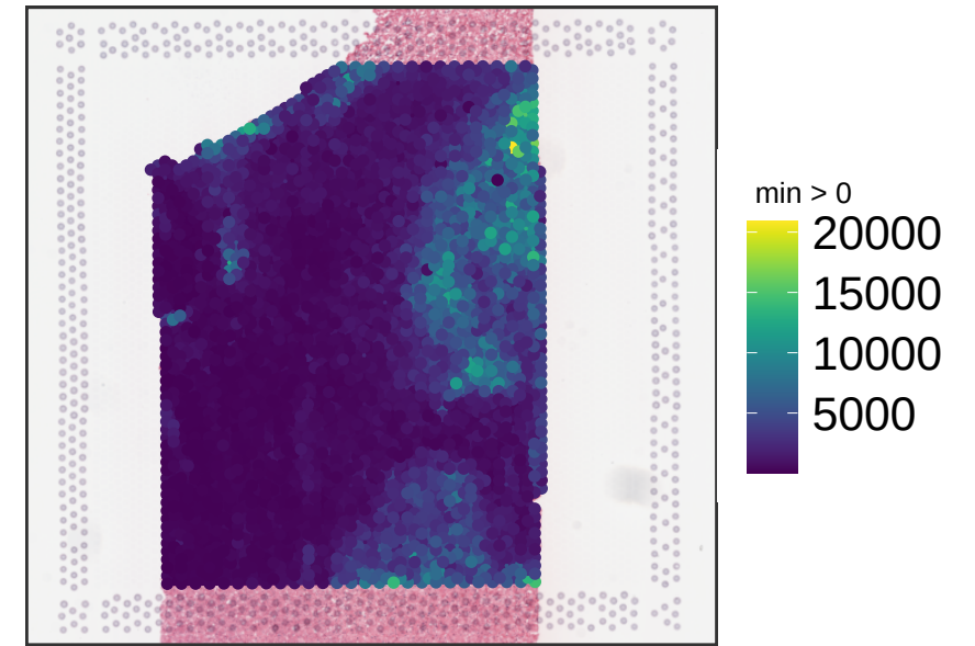
V13M06-387_D1 sum_umi
