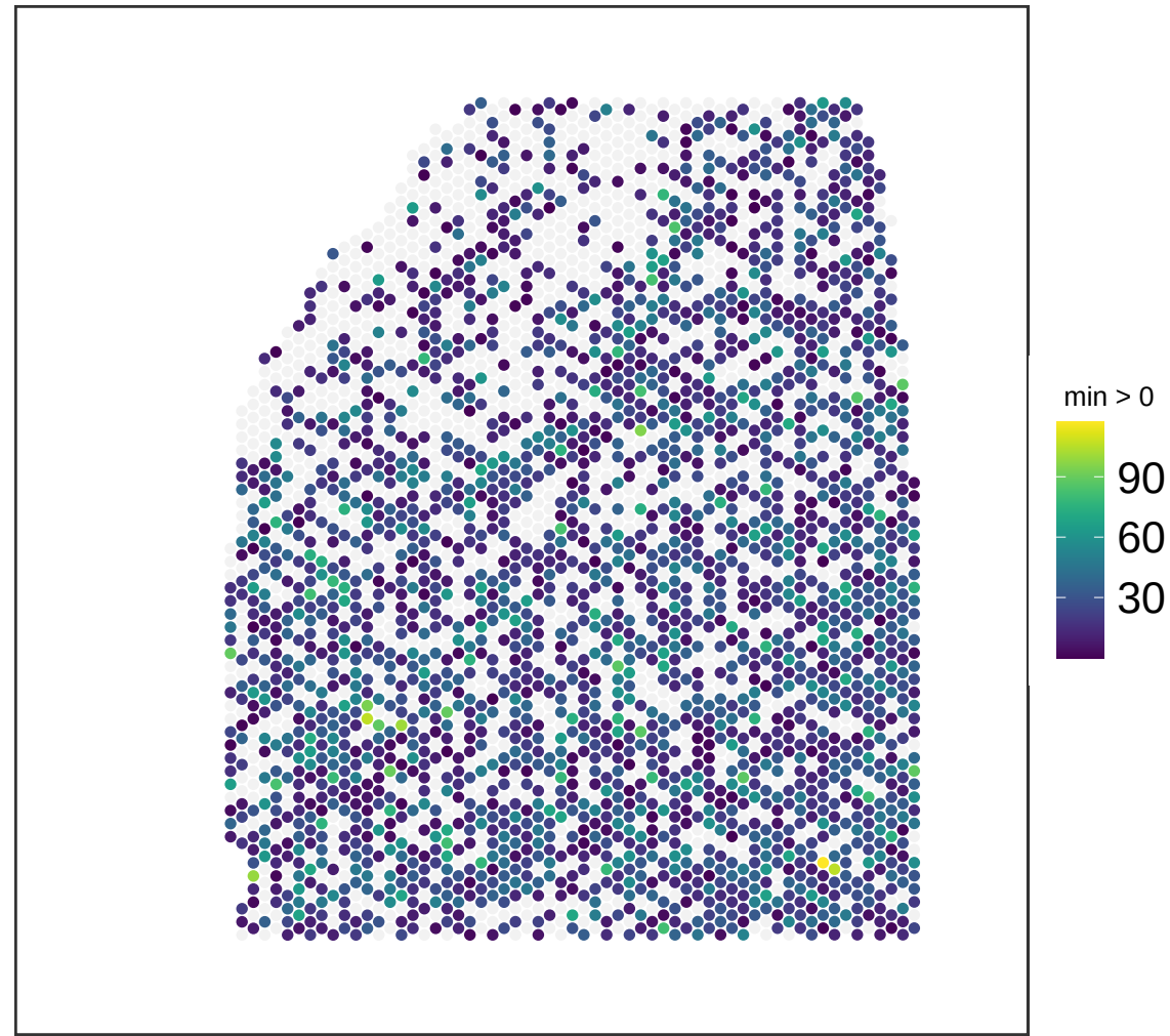
V13M06-388_B1 NMF_14
