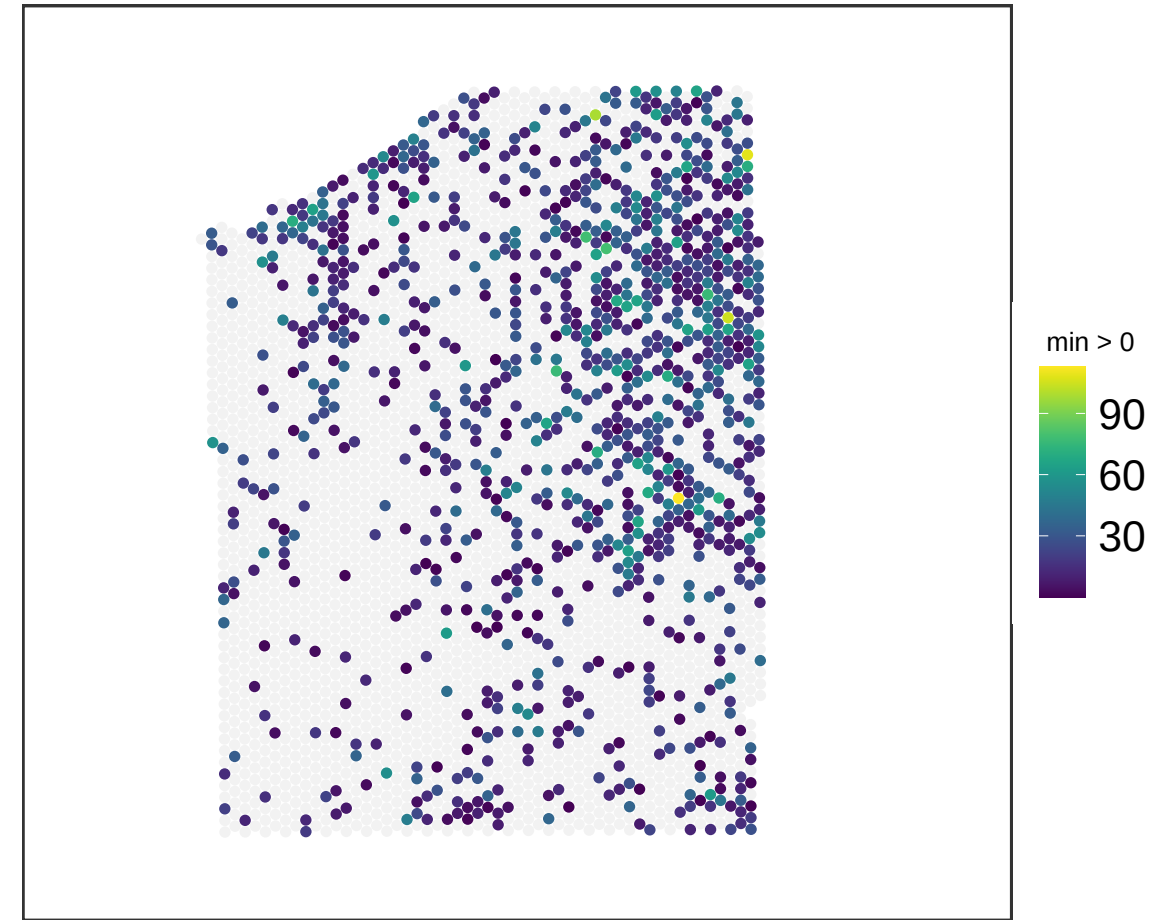
V13M06-387_D1 NMF_14
