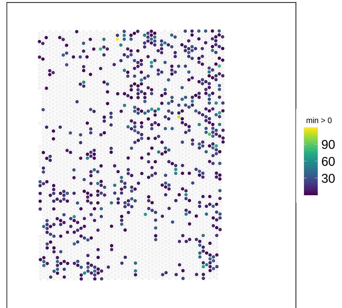
V13M06-387_C1 NMF_14
