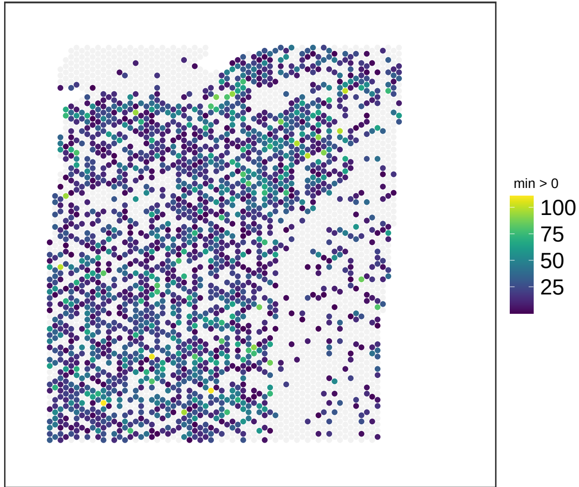
V13M06-388_A1 NMF_14
