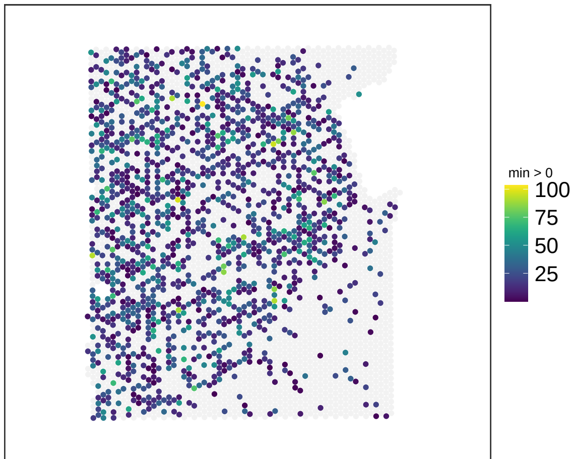
V13M06-387_A1 NMF_14
