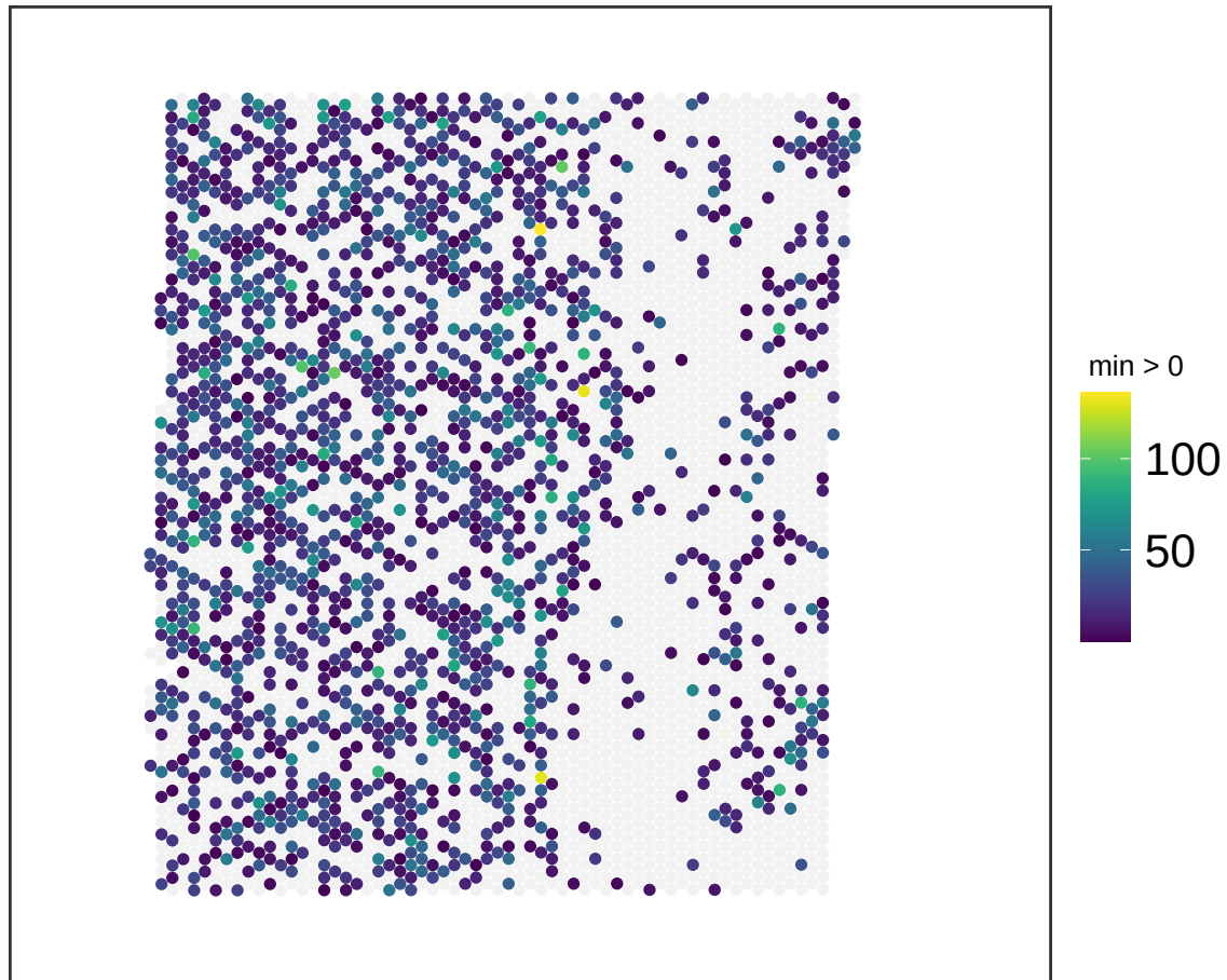
V13M06-388_C1 NMF_14
