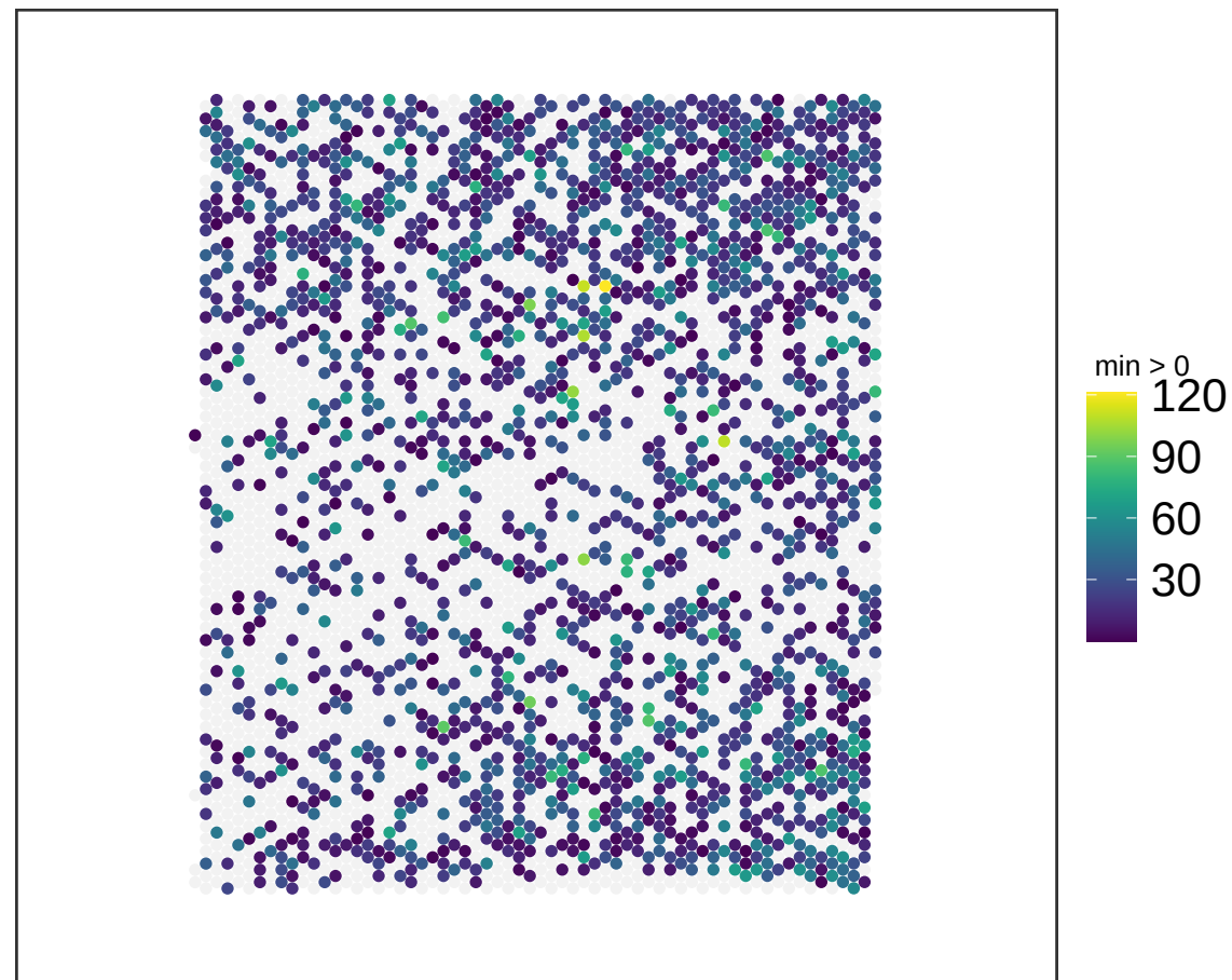
V13M06-388_D1 NMF_14
