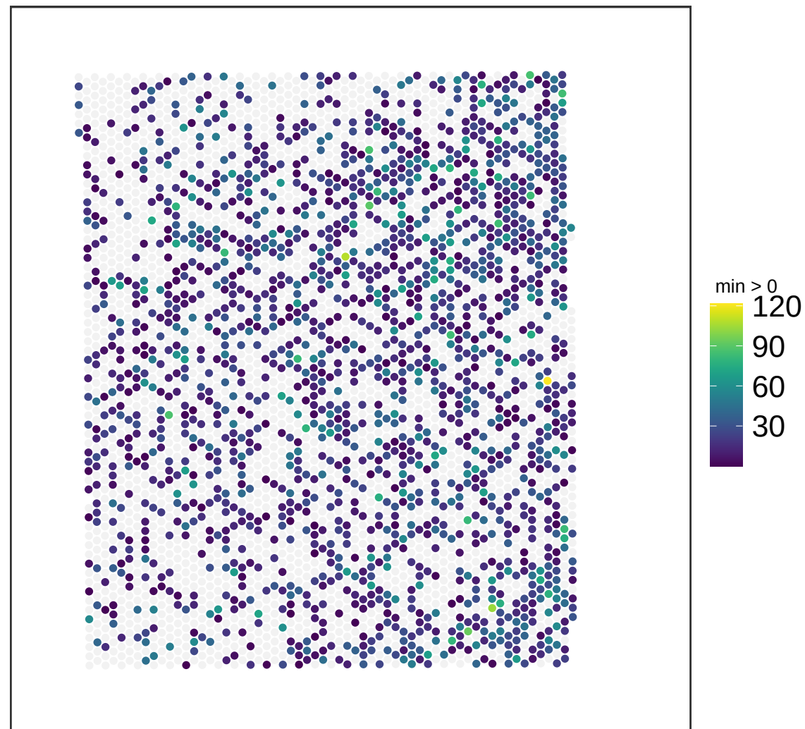
V13M06-387_B1 NMF_14
