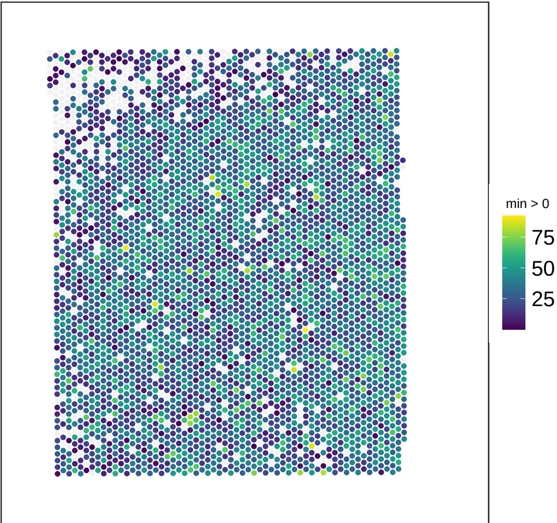
V13M06-387_B1 NMF_4
