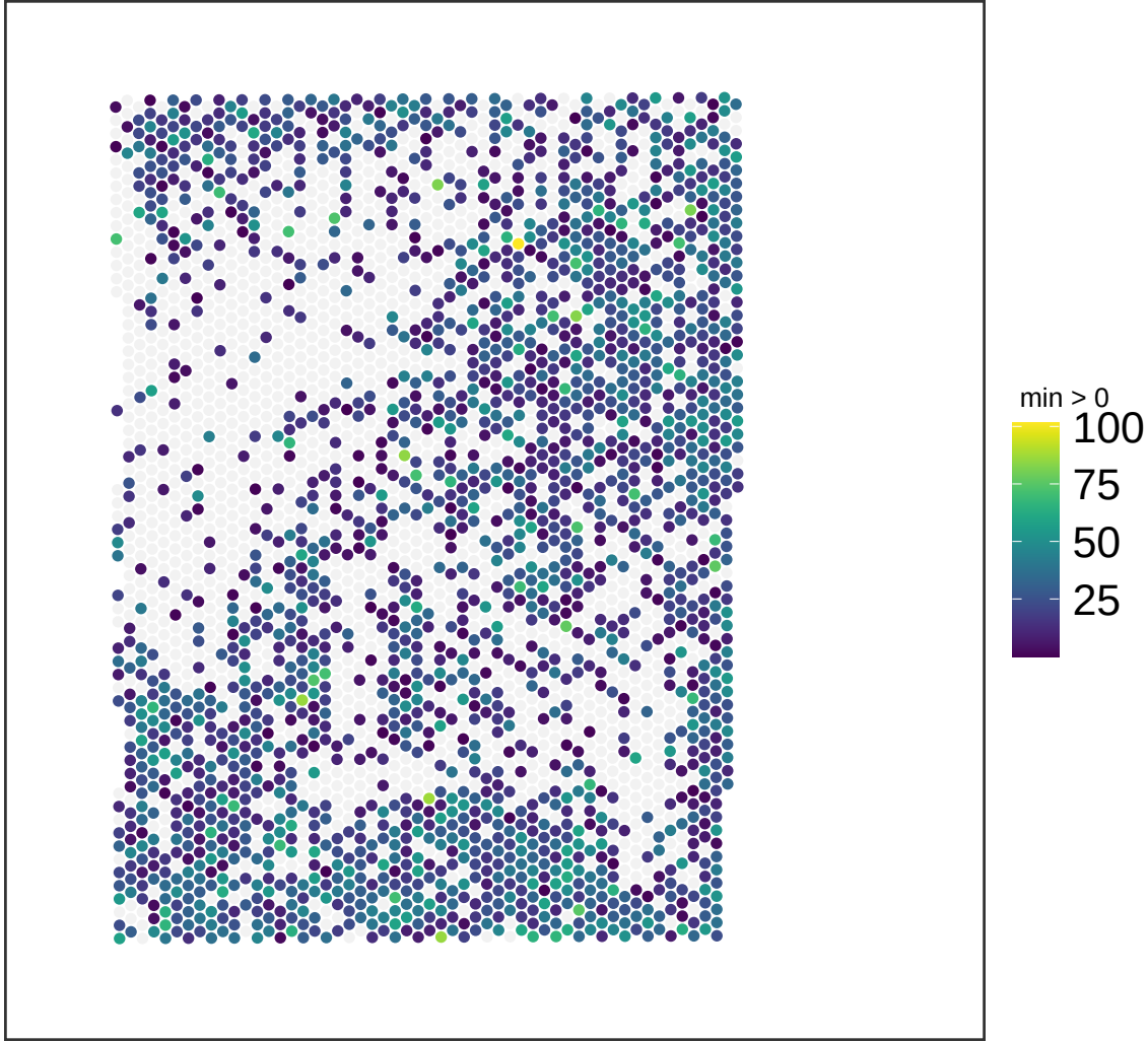
V13M06-387_C1 NMF_4
