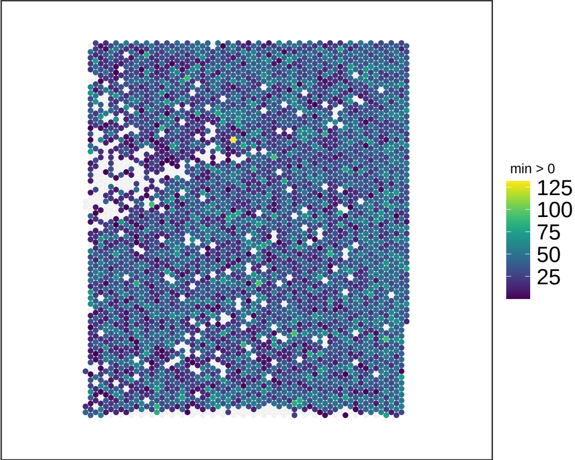
V13M06-388_D1 NMF_4
