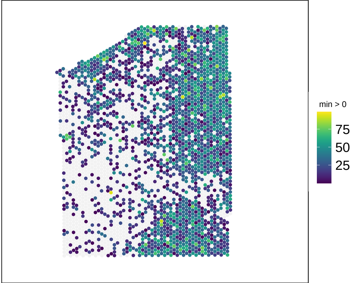
V13M06-387_D1 NMF_4
