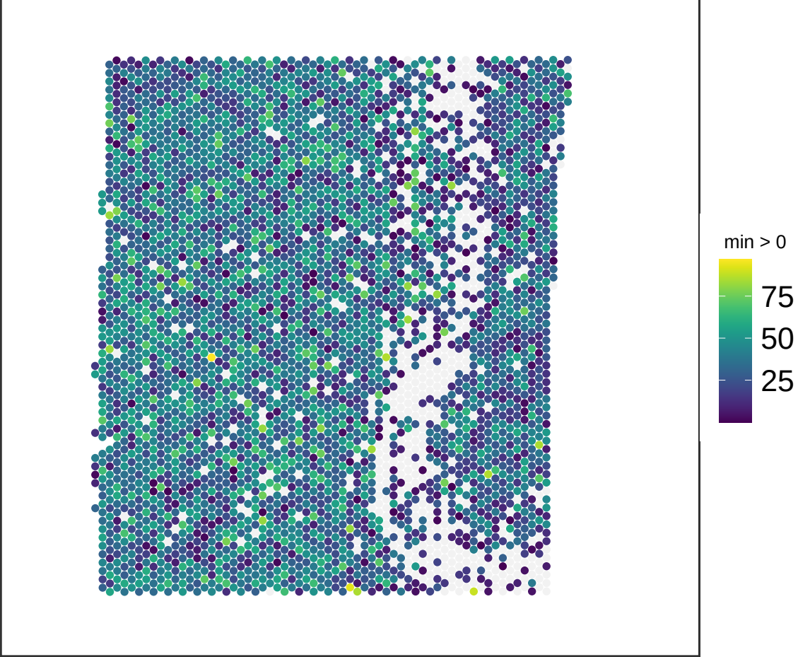
V13M06-388_C1 NMF_4
