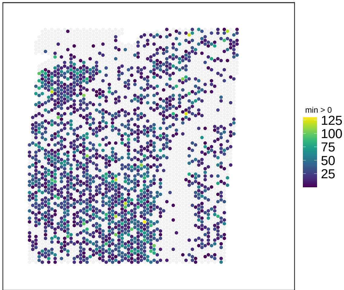
V13M06-388_A1 NMF_49
