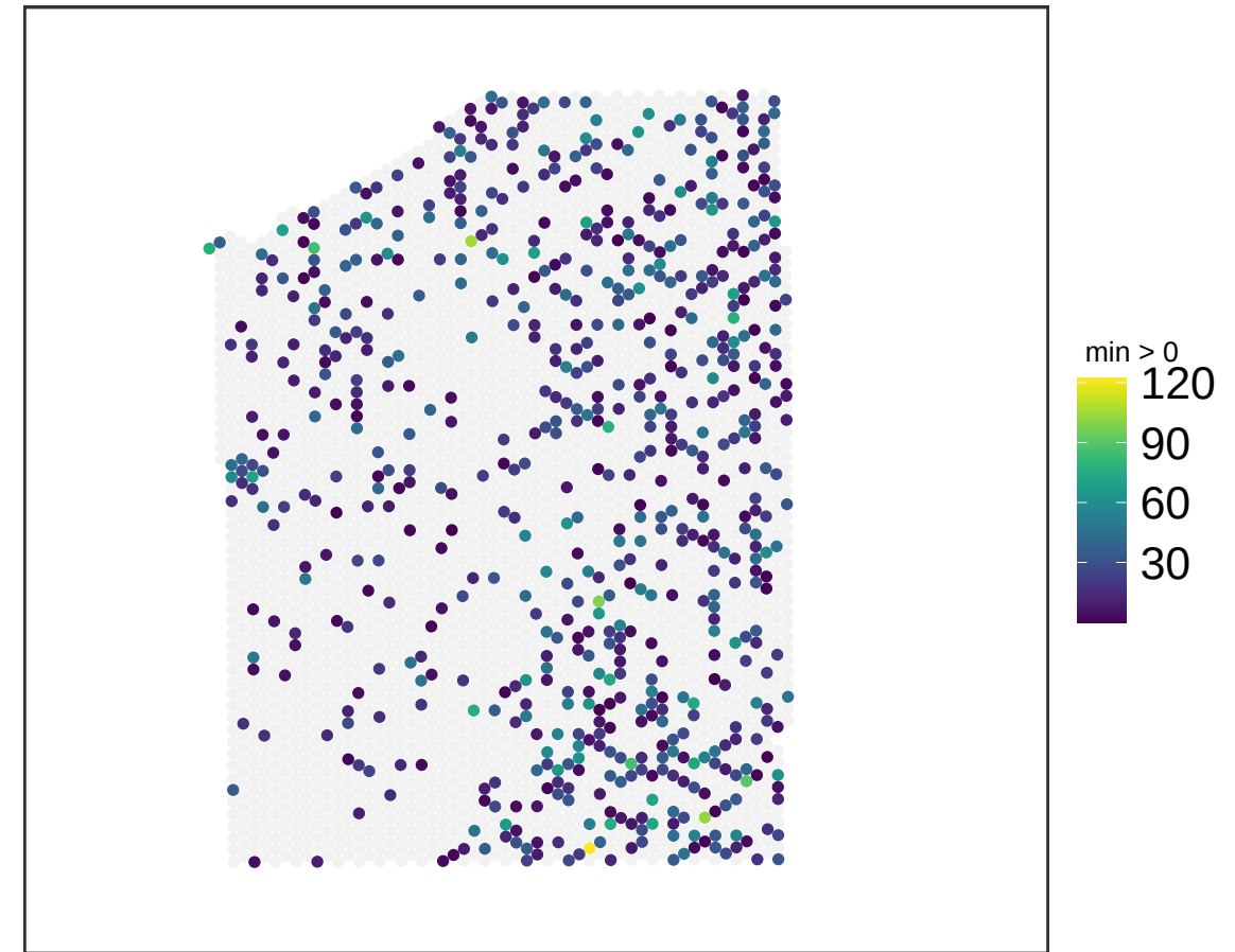
V13M06-387_D1 NMF_49
