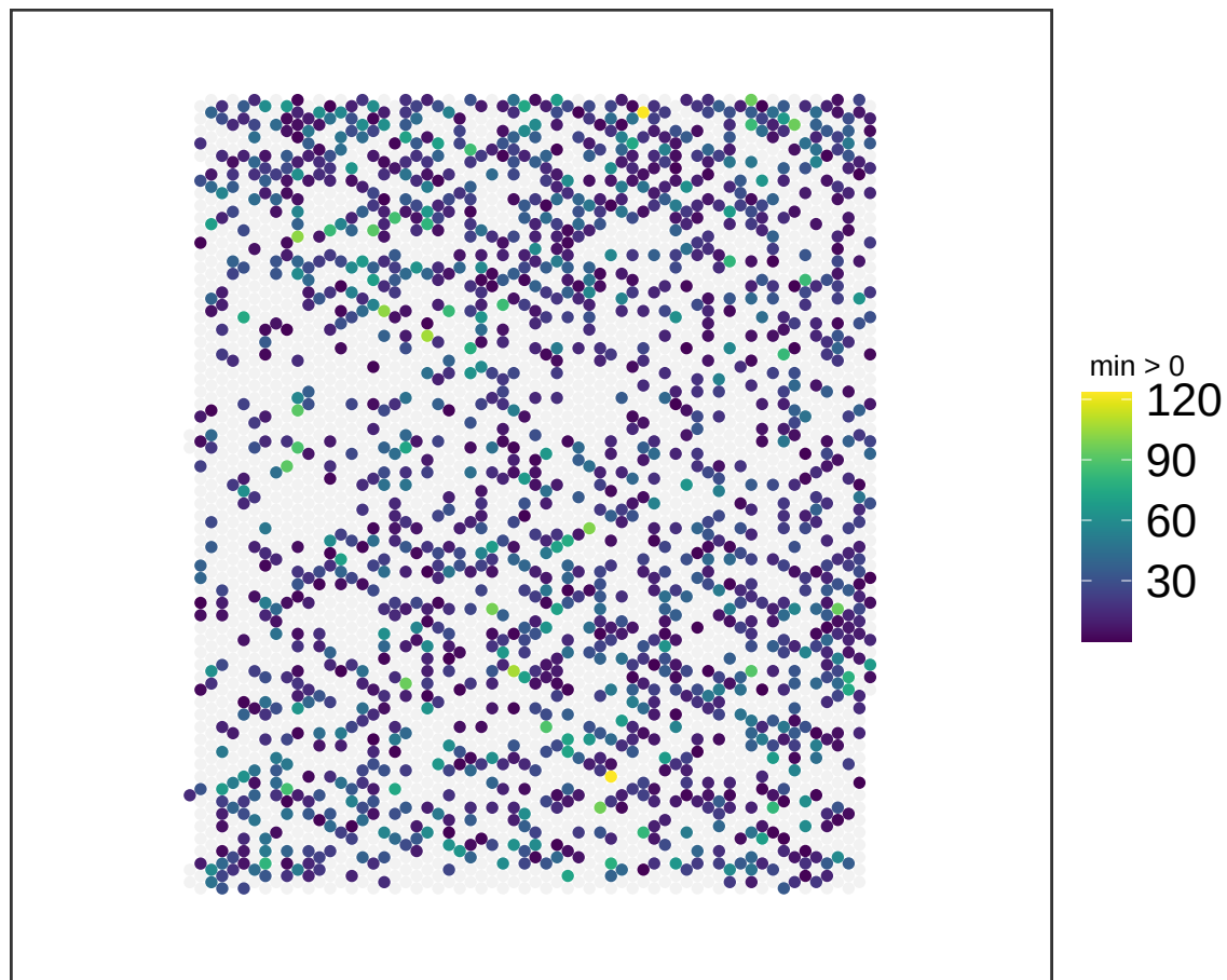
V13M06-388_D1 NMF_49
