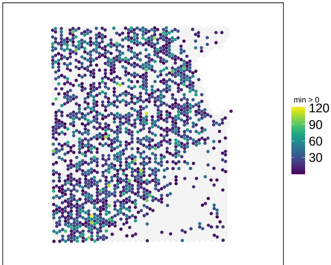
V13M06-387_A1 NMF_49
