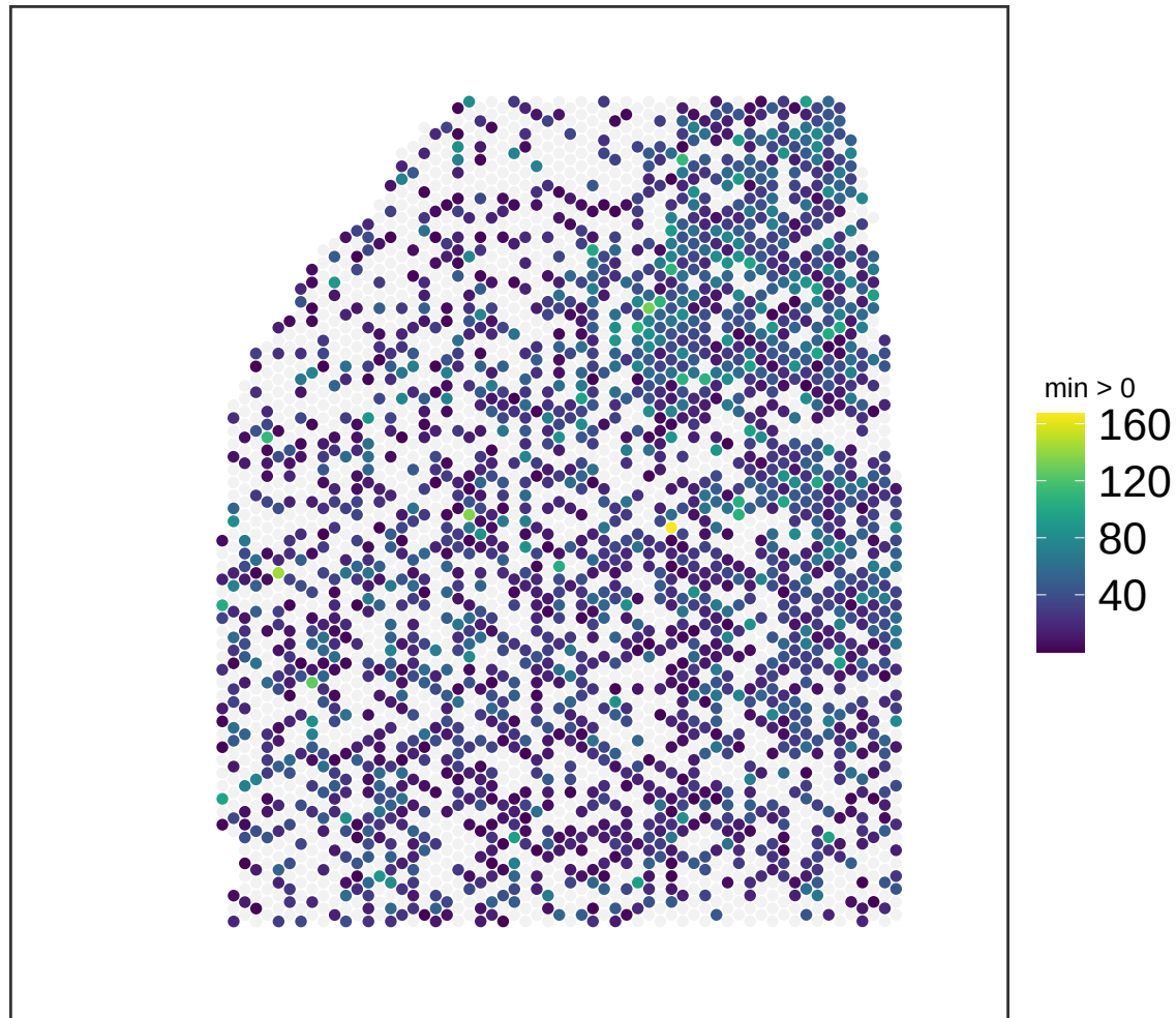
V13M06-388_B1 NMF_49
