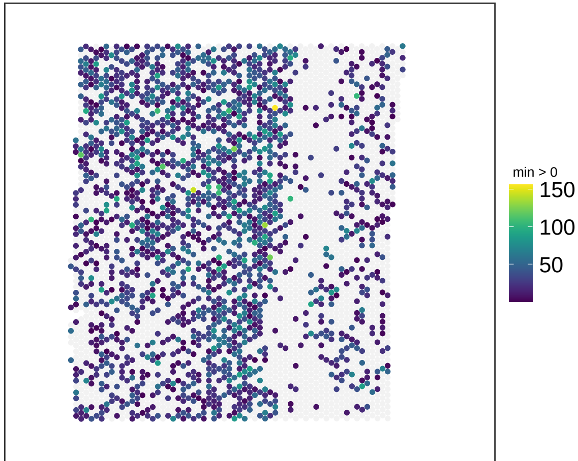
V13M06-388_C1 NMF_49
