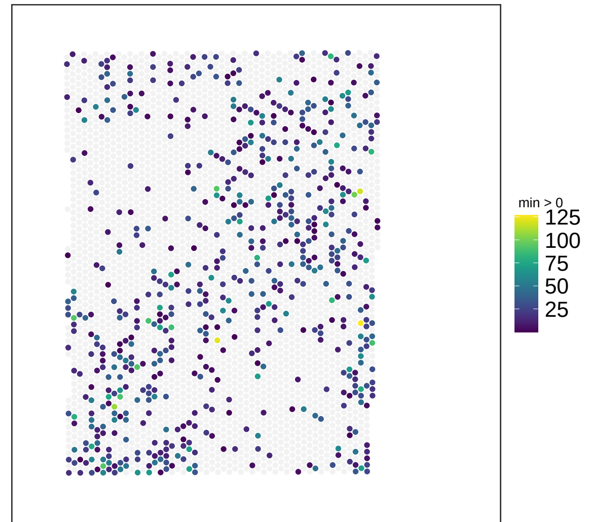
V13M06-387_C1 NMF_49
