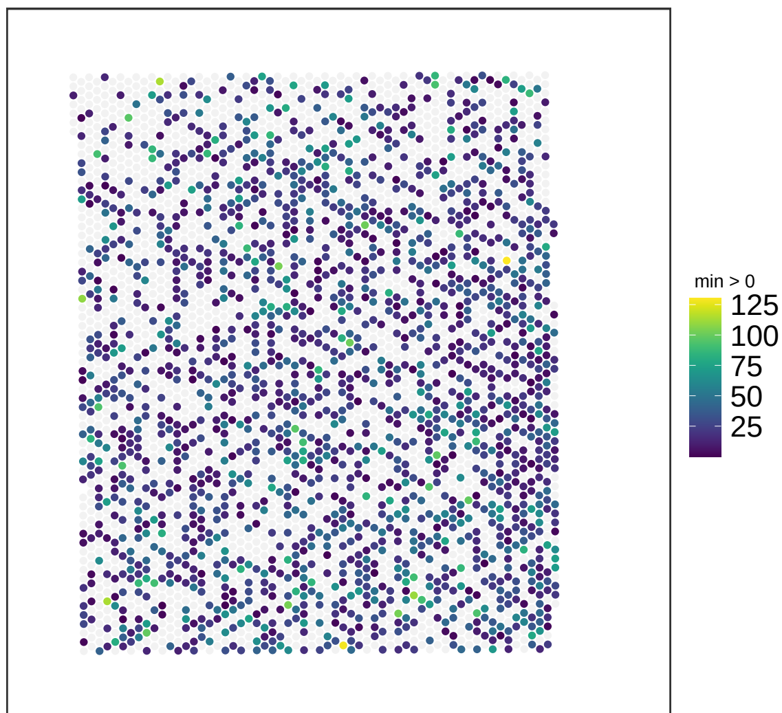
V13M06-387_B1 NMF_49
