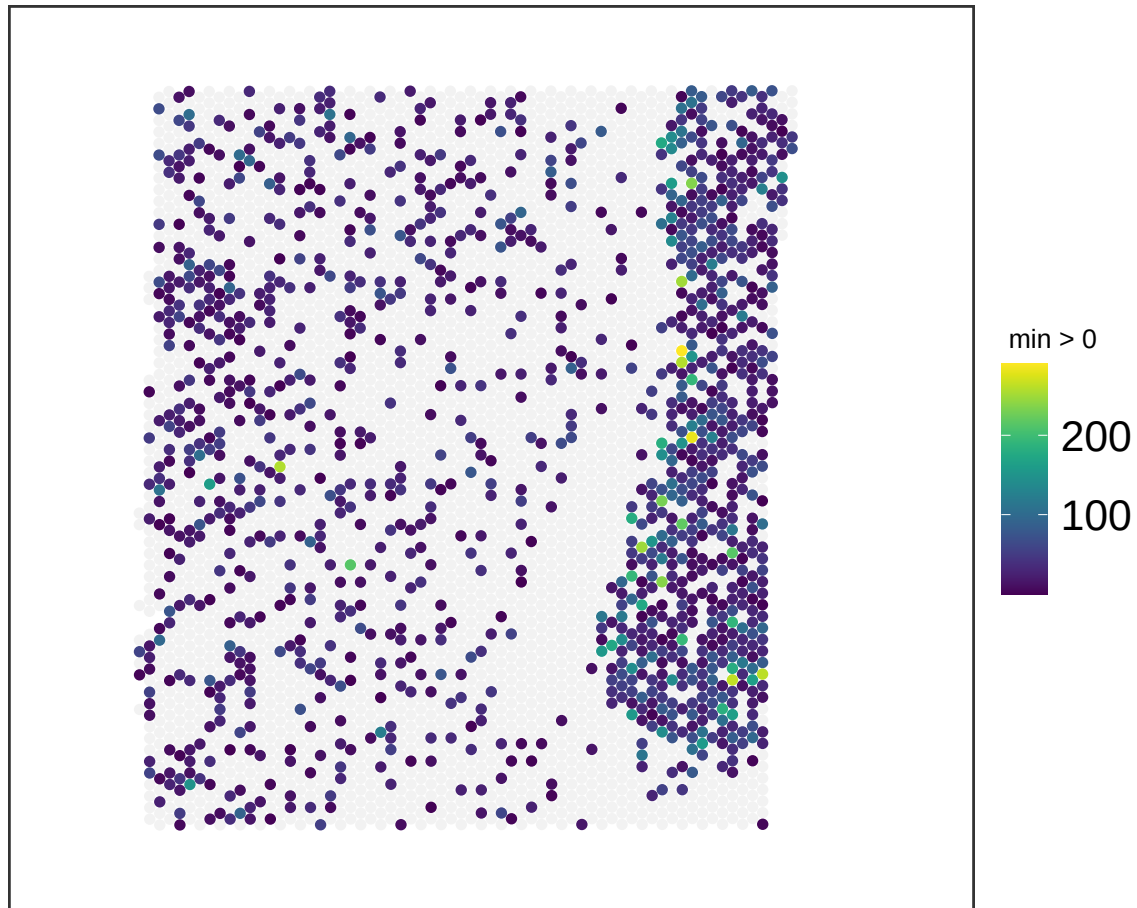
V13M06-388_C1 NMF_63
