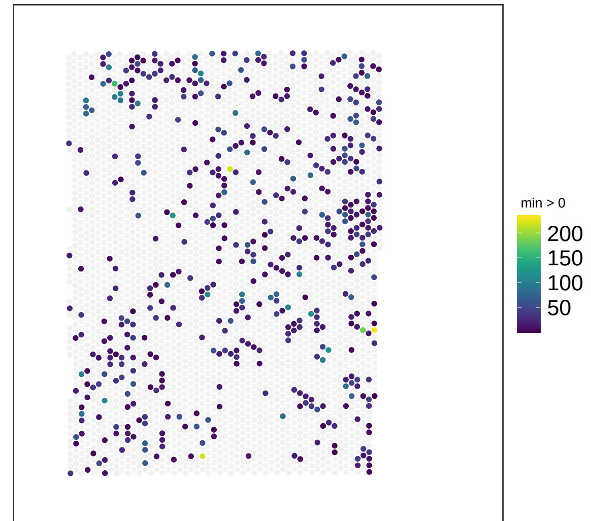
V13M06-387_C1 NMF_63
