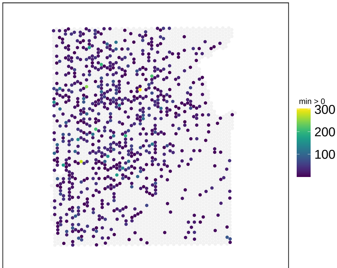
V13M06-387_A1 NMF_63
