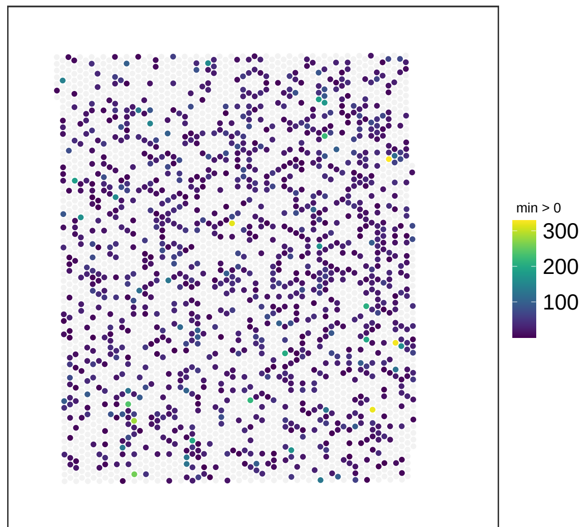
V13M06-387_B1 NMF_63
