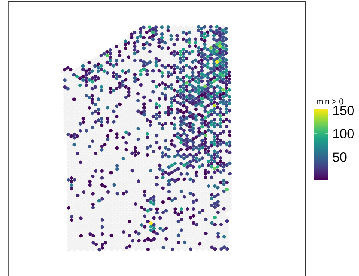
V13M06-387_D1 NMF_63
