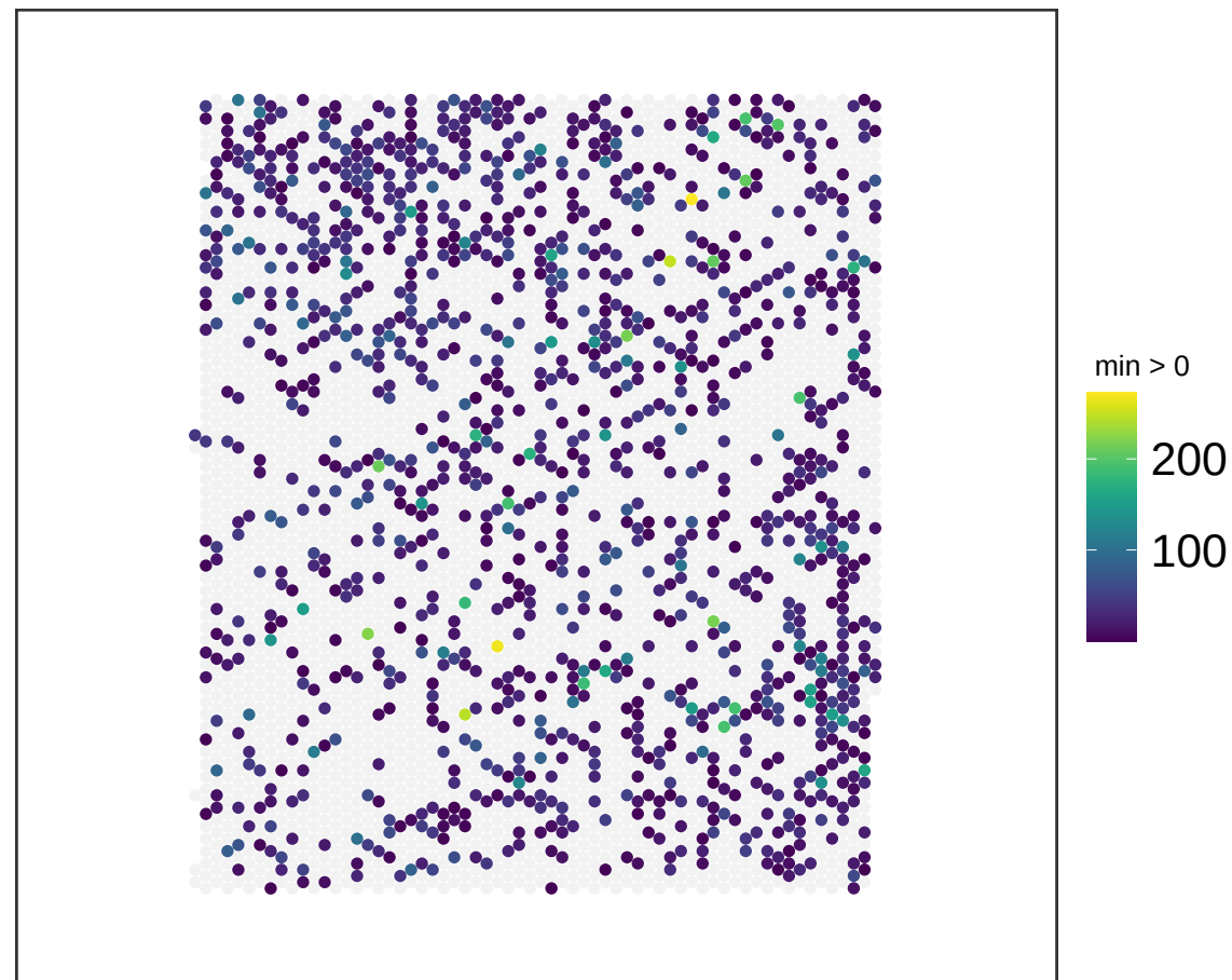
V13M06-388_D1 NMF_63
