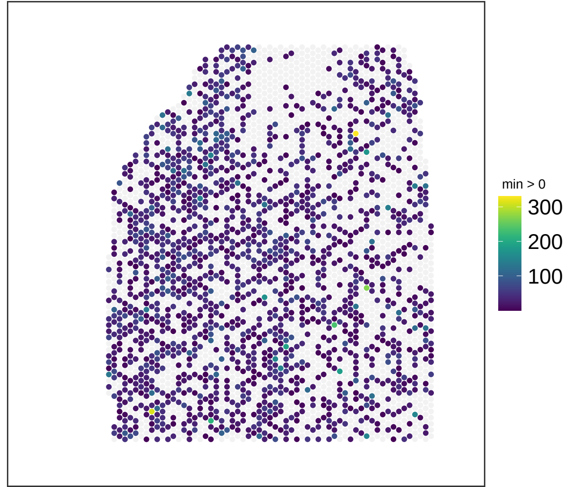
V13M06-388_B1 NMF_63
