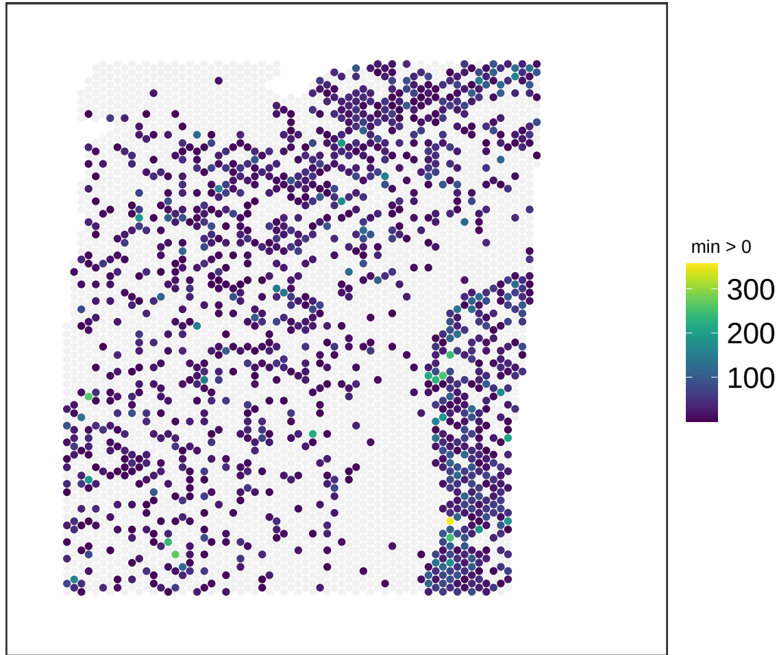
V13M06-388_A1 NMF_63
