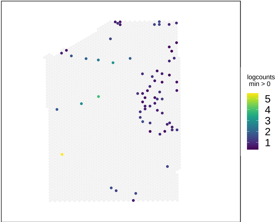
V13M06-387_D1 TMEM132D
