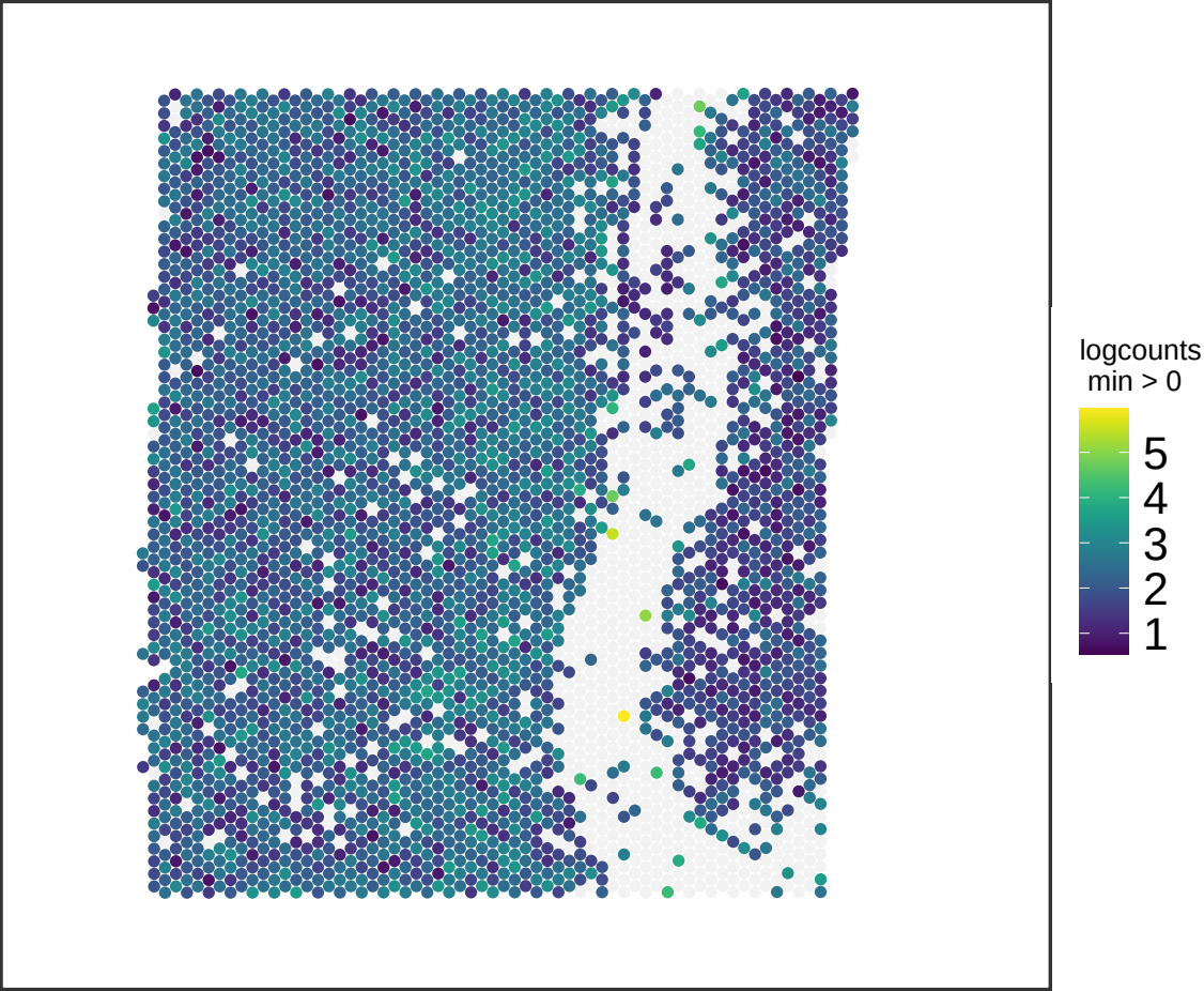
V13M06-388_C1 PCSK1N
