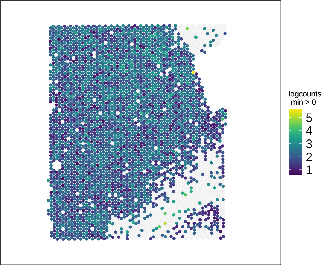
V13M06-387_A1 PCSK1N
