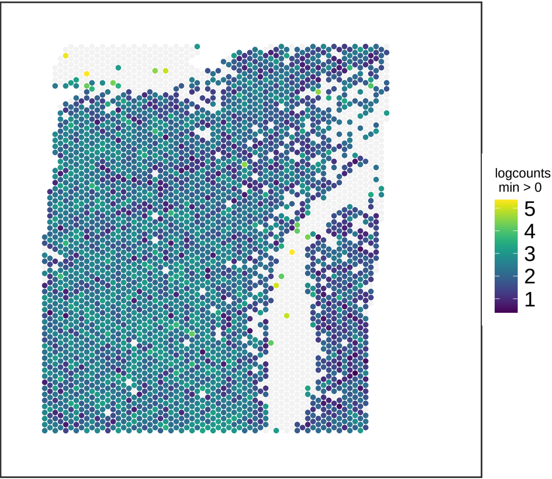
V13M06-388_A1 PCSK1N
