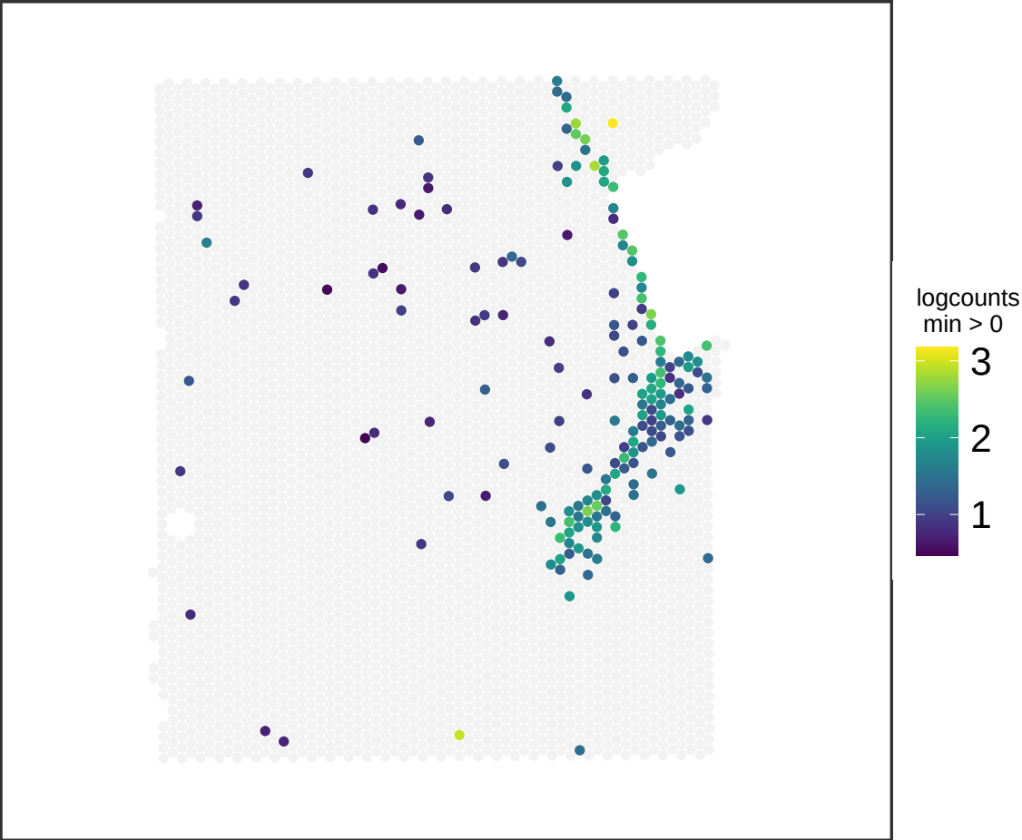
V13M06-387_A1 FAM183A
