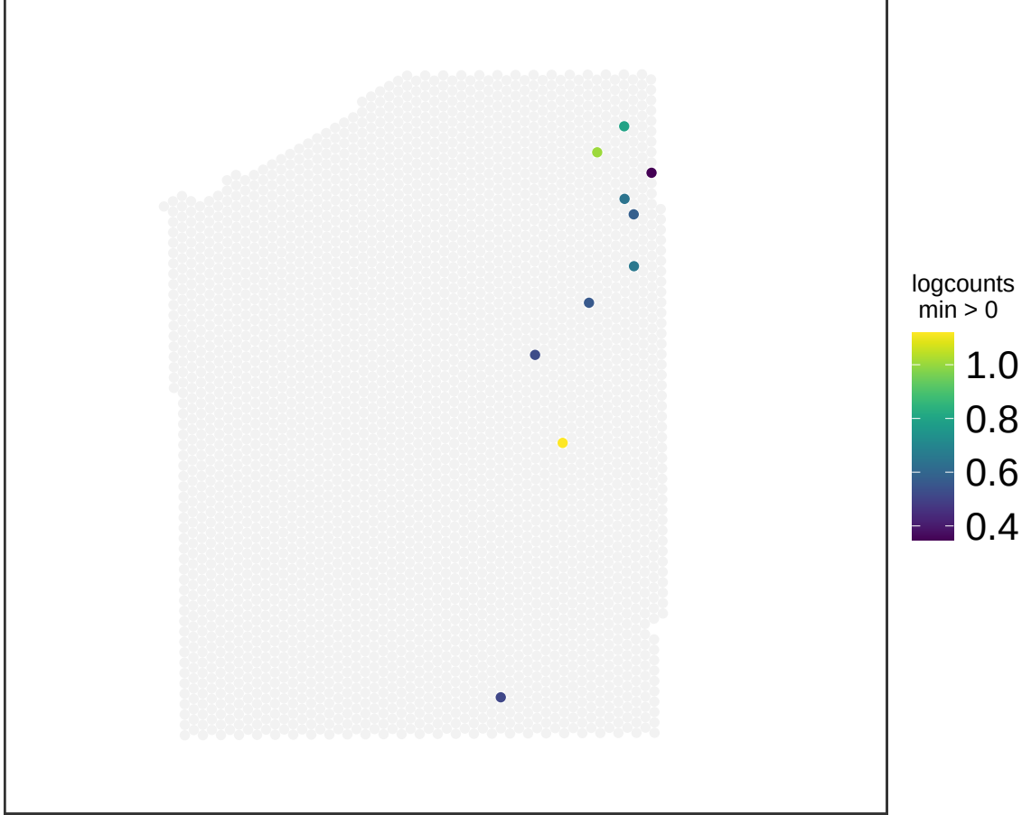
V13M06-387_D1 FAM183A
