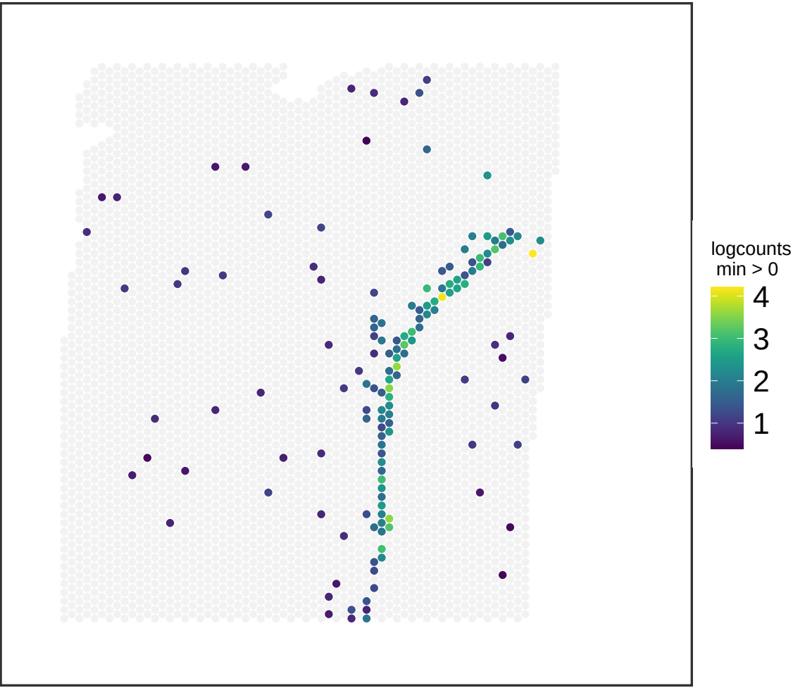
V13M06-388_A1 FAM183A
