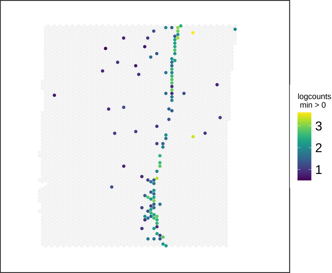
V13M06-388_C1 FAM183A
