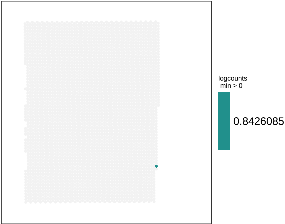
V13M06-387_C1 FAM183A
