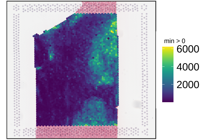
V13M06-387_D1 sum_gene
