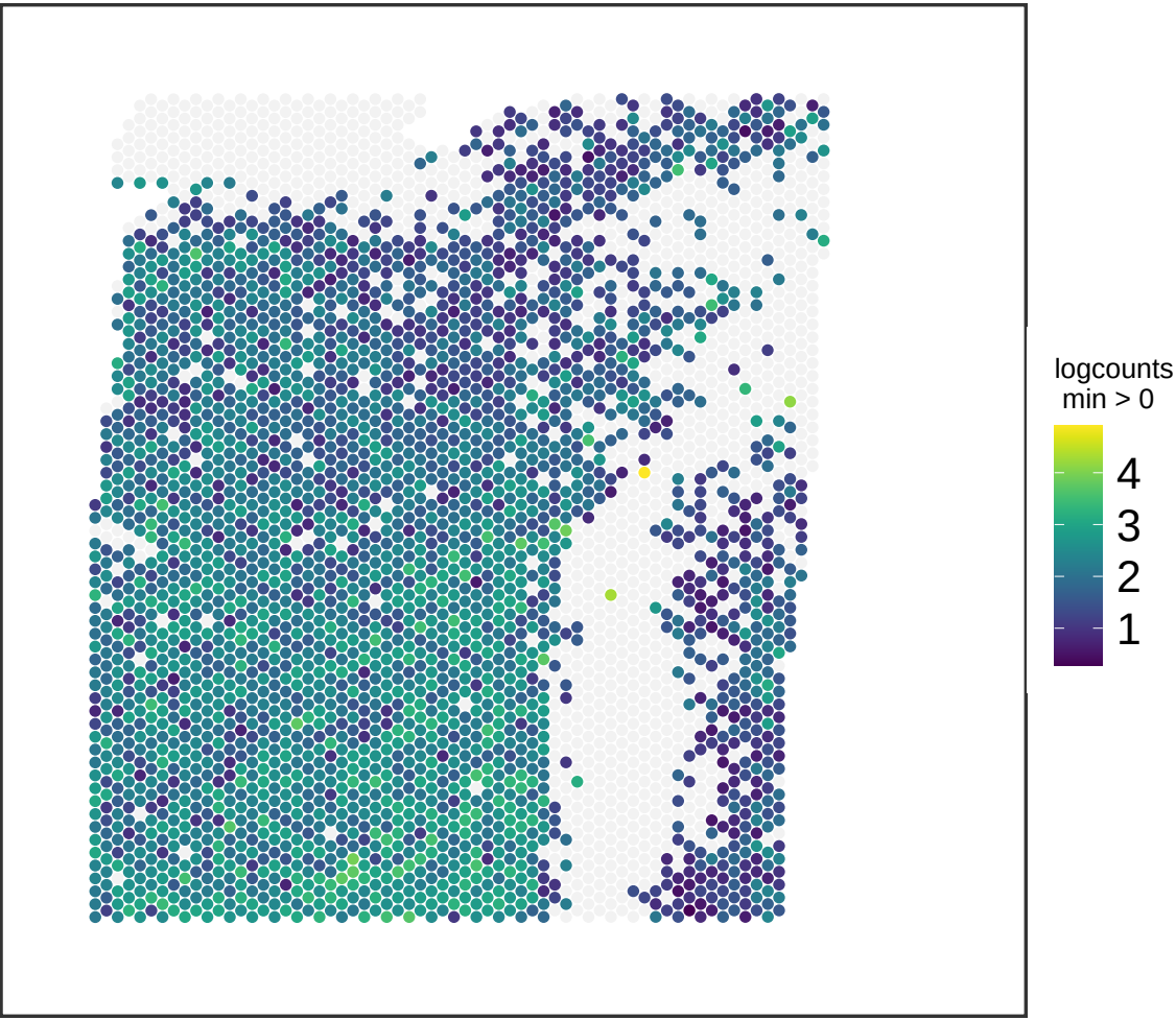
V13M06-388_A1 NPTX1
