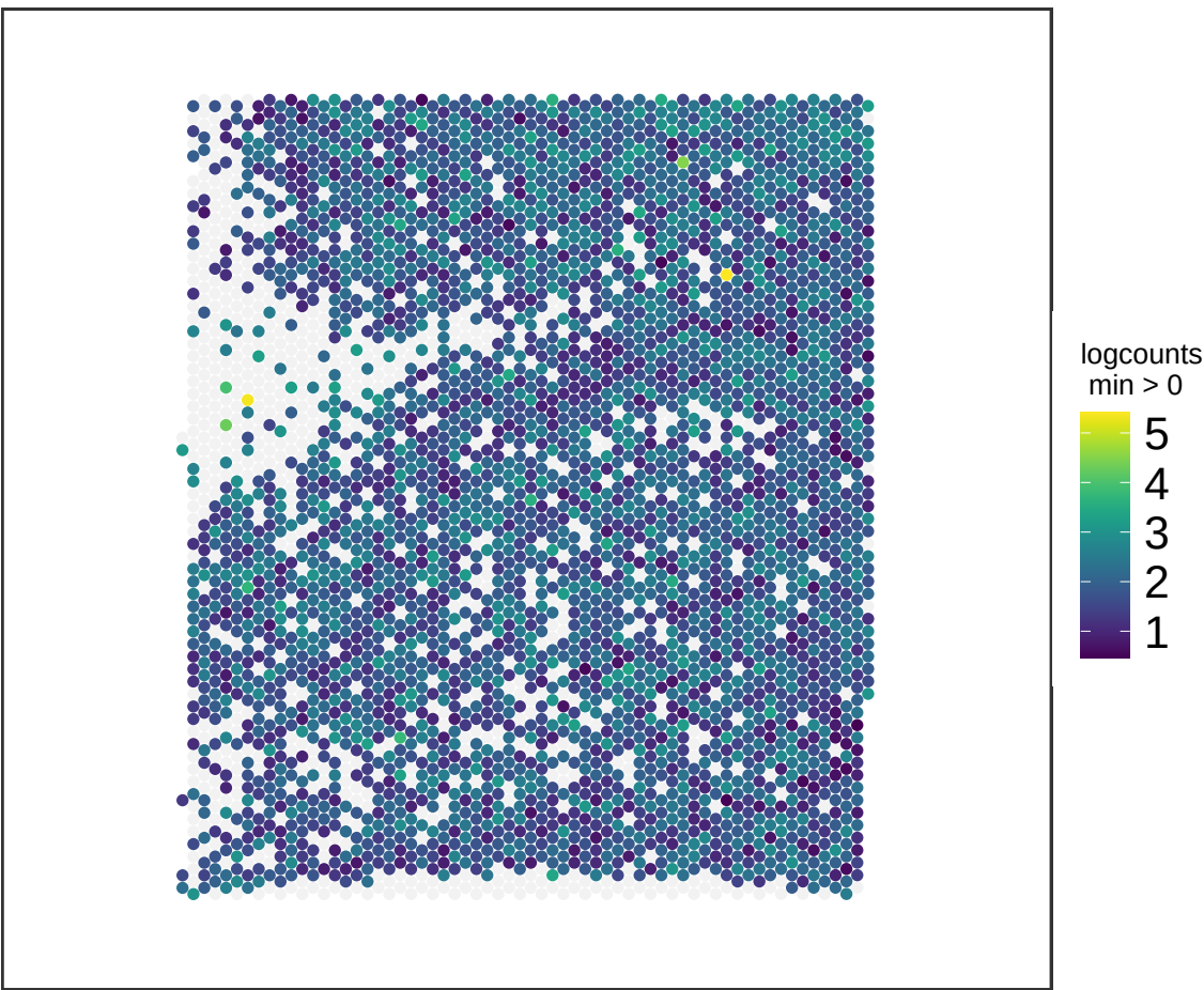
V13M06-388_D1 NPTX1
