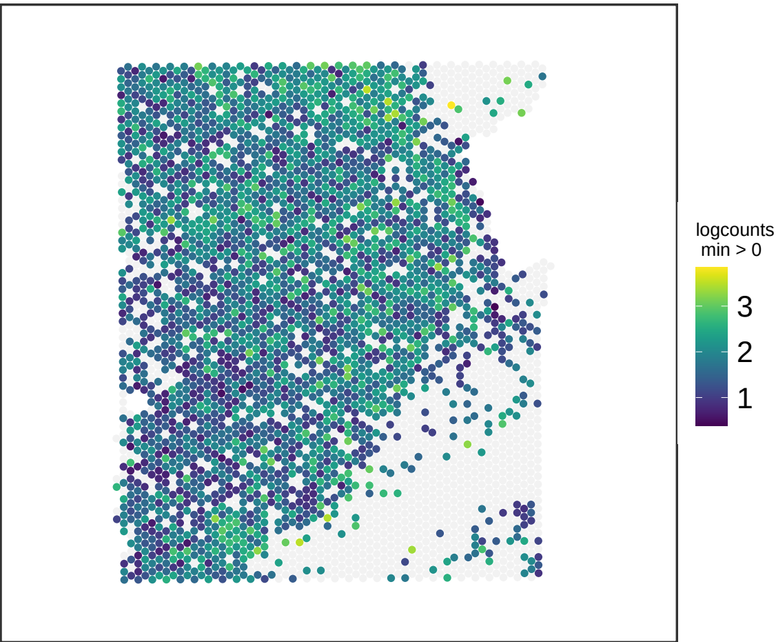
V13M06-387_A1 NPTX1
