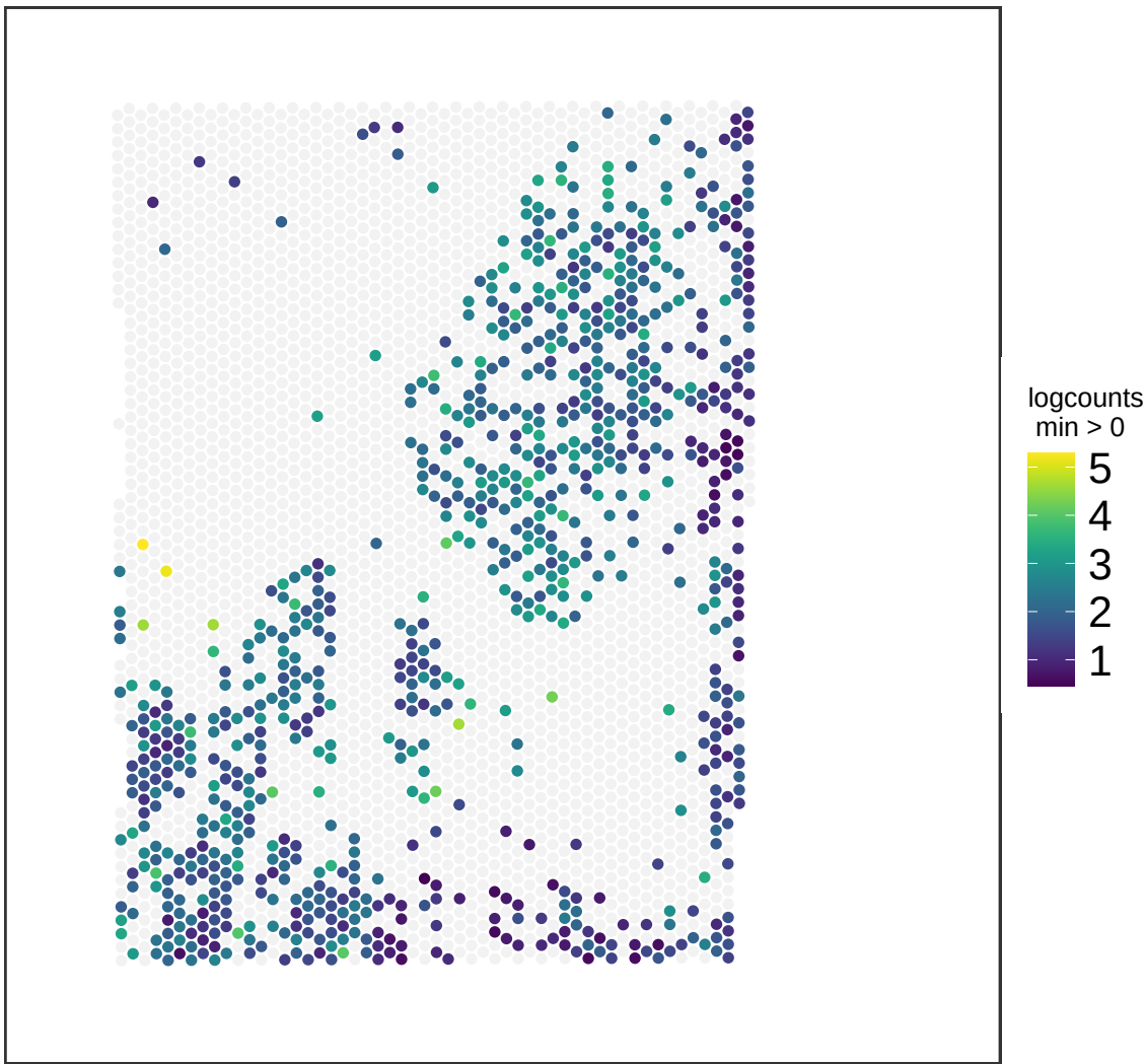
V13M06-387_C1 NPTX1
