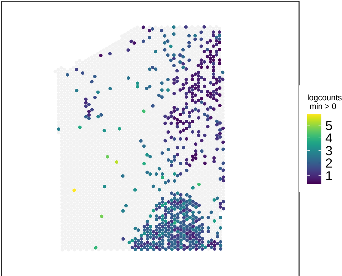
V13M06-387_D1 NPTX1
