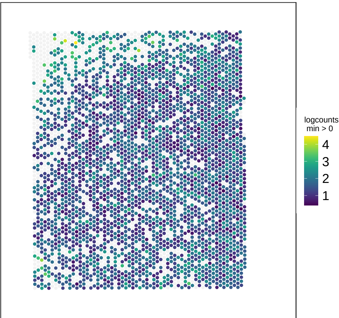
V13M06-387_B1 NPTX1
