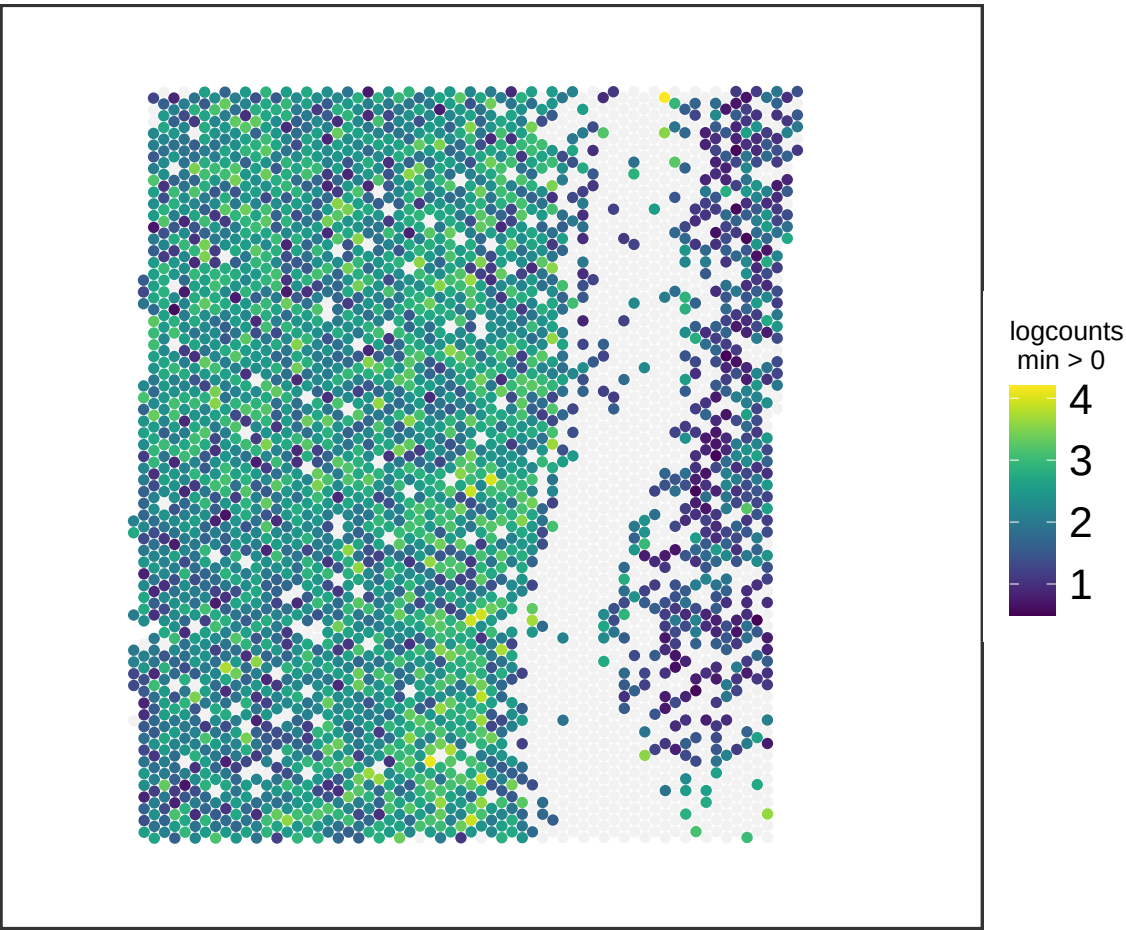
V13M06-388_C1 NPTX1
