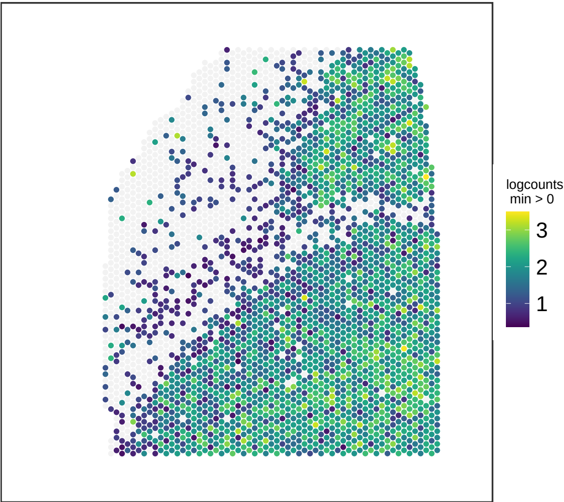
V13M06-388_B1 NPTX1
