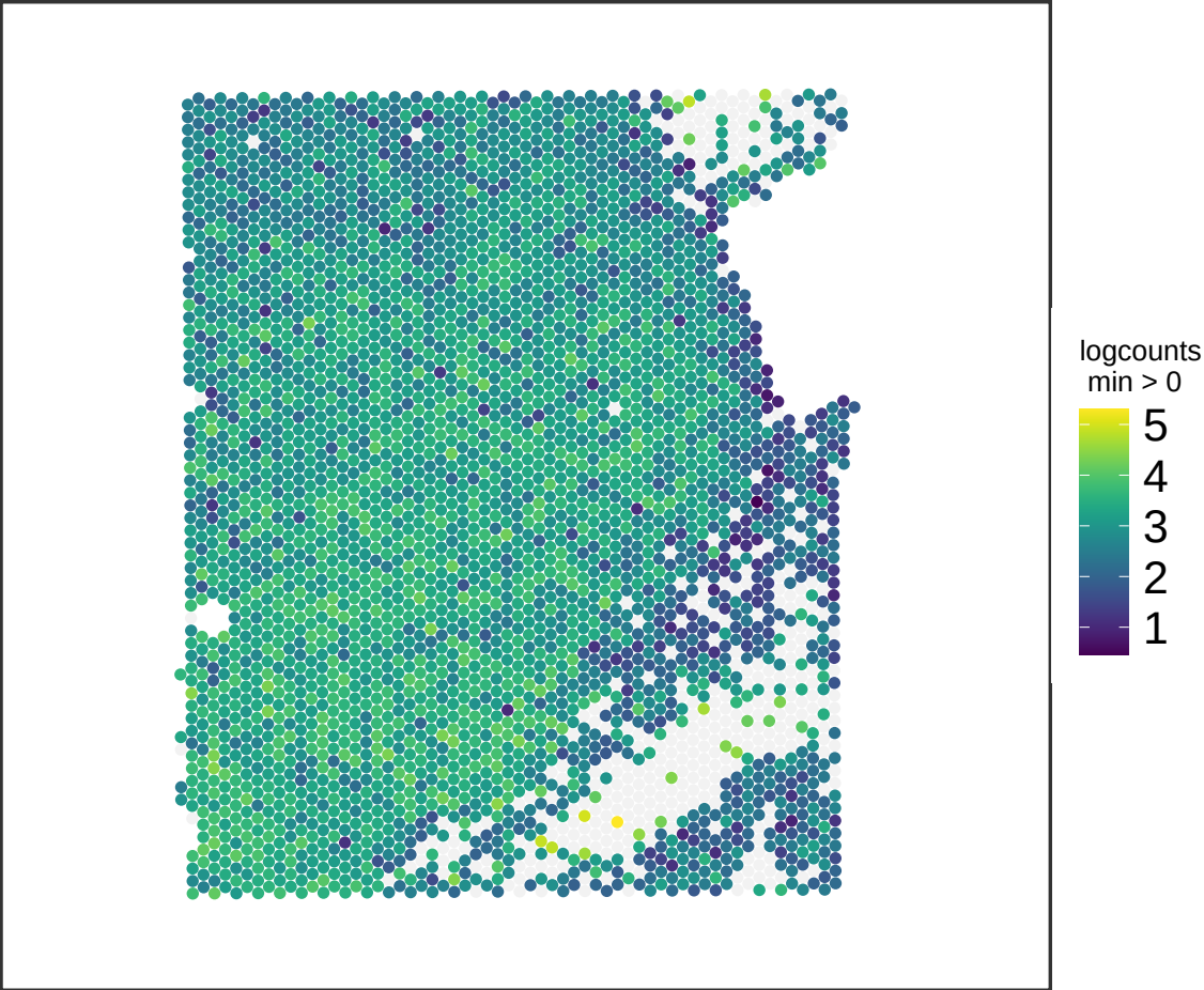
V13M06-387_A1 CAMK2N1
