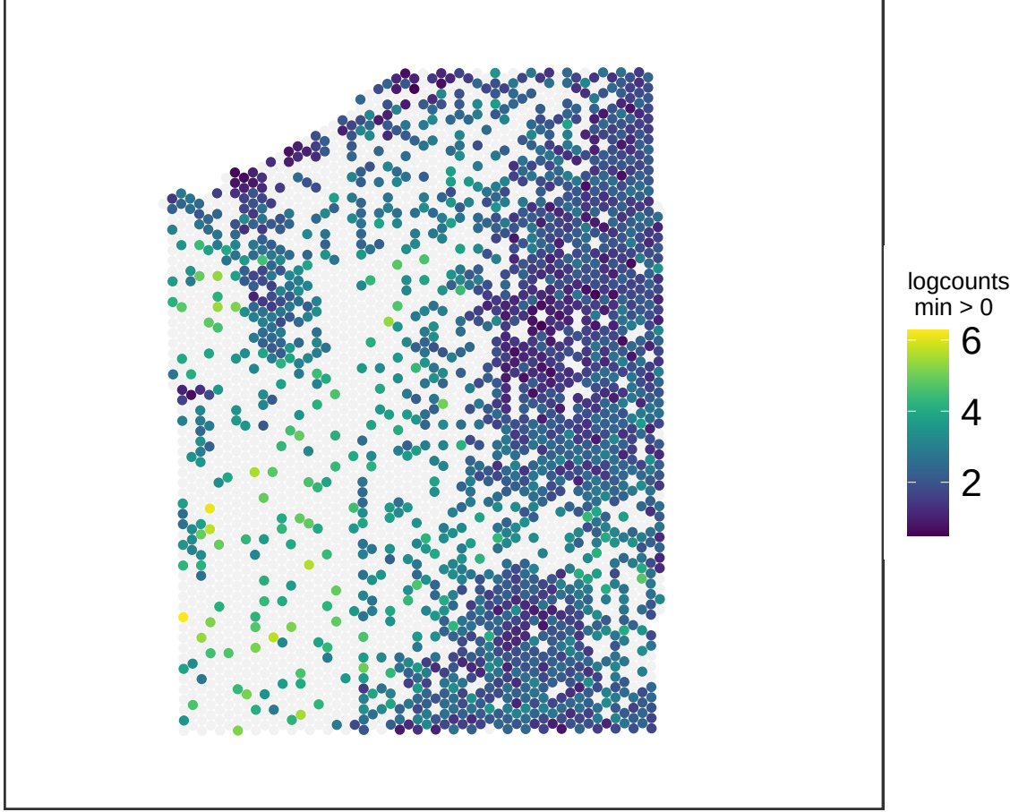
V13M06-387_D1 CAMK2N1
