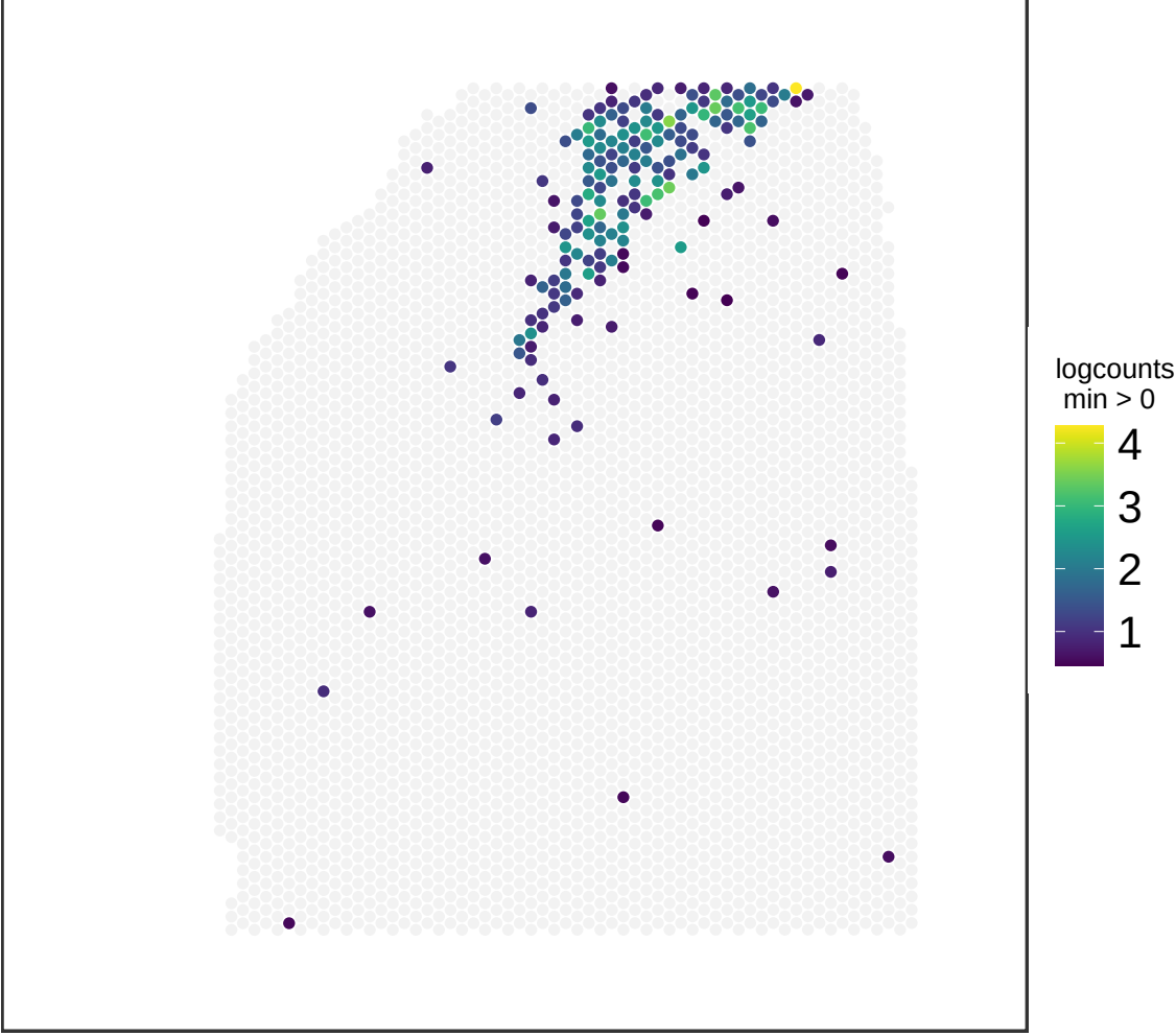
V13M06-388_B1 TTR
