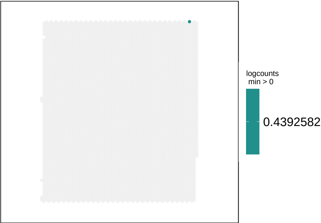
V13M06-388_D1 TTR
