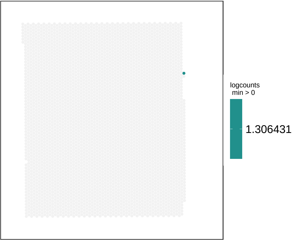
V13M06-387_B1 TTR
