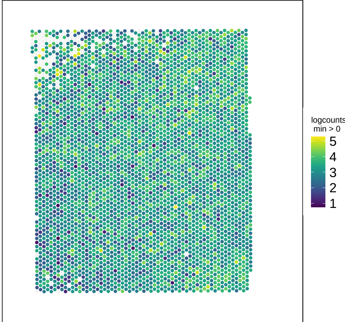
V13M06-387_B1 SPARCL1
