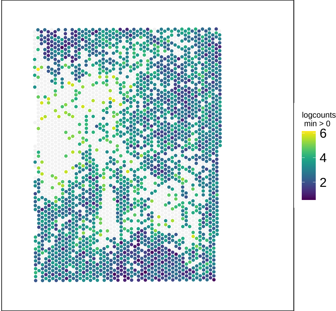
V13M06-387_C1 SPARCL1
