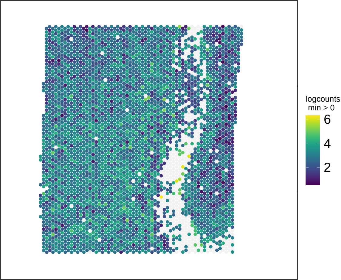
V13M06-388_C1 SPARCL1
