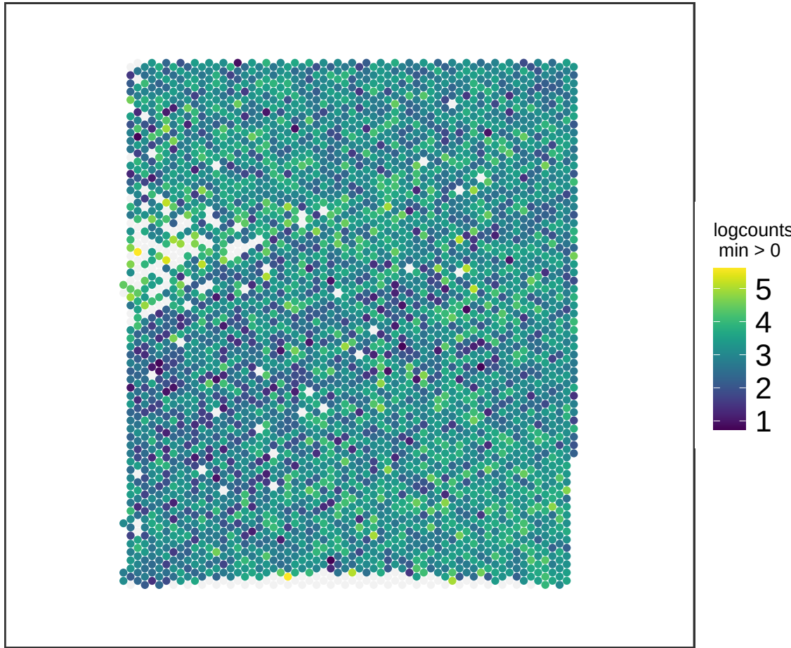
V13M06-388_D1 SPARCL1
