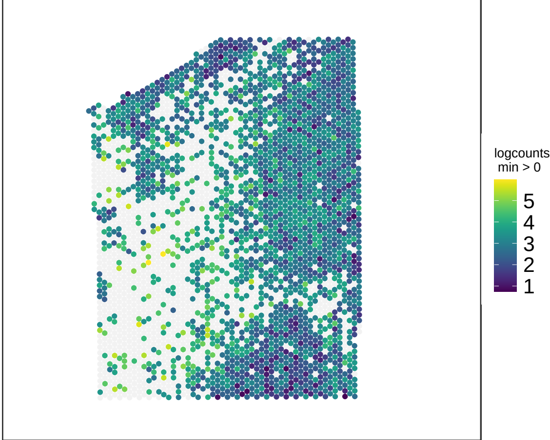
V13M06-387_D1 SPARCL1
