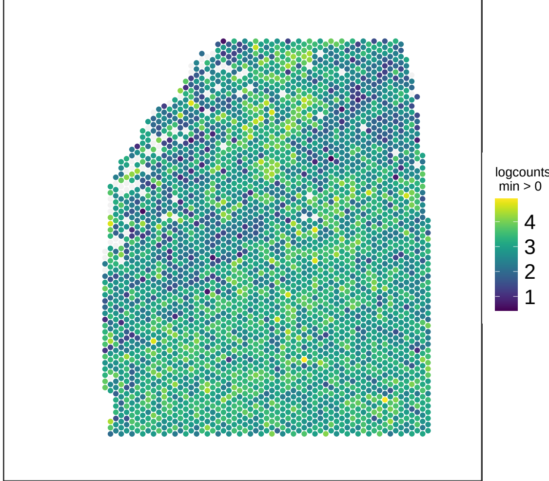
V13M06-388_B1 SPARCL1
