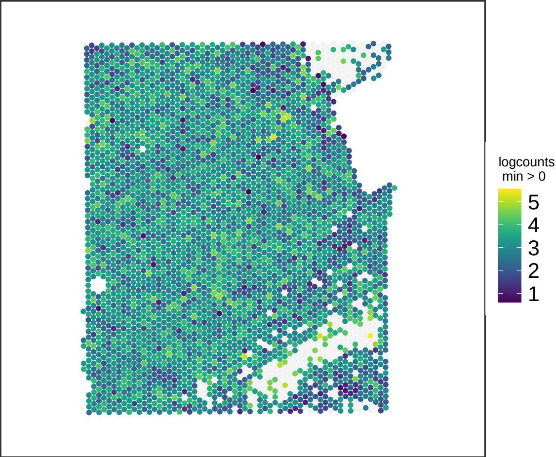
V13M06-387_A1 SPARCL1
