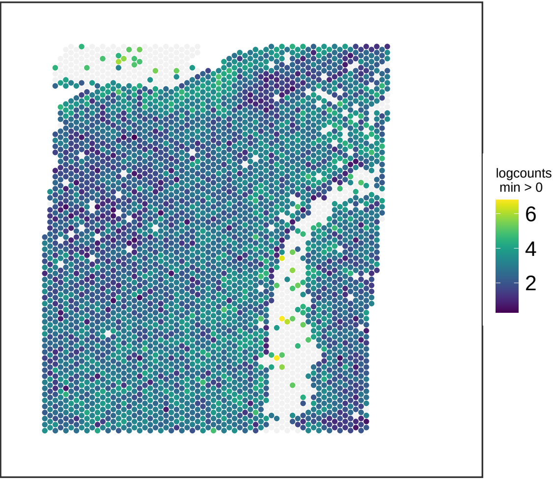
V13M06-388_A1 SPARCL1
