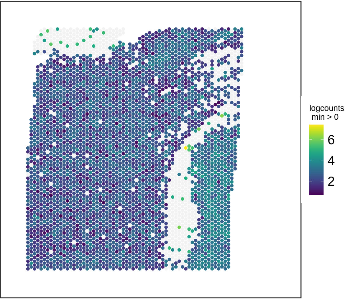
V13M06-388_A1 ATP1B1
