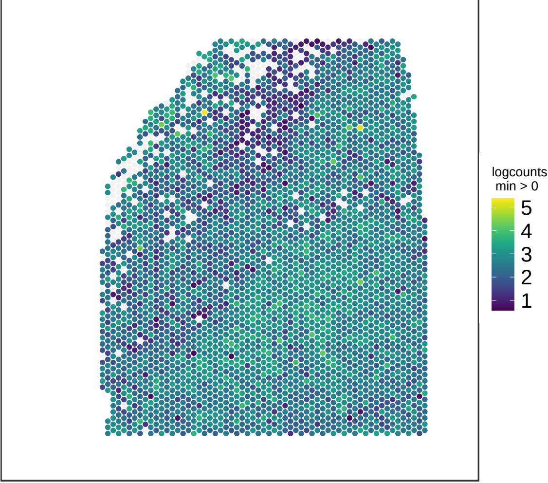
V13M06-388_B1 ATP1B1
