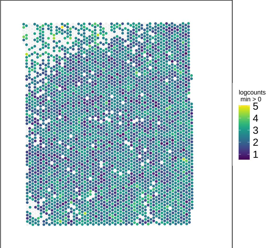
V13M06-387_B1 ATP1B1
