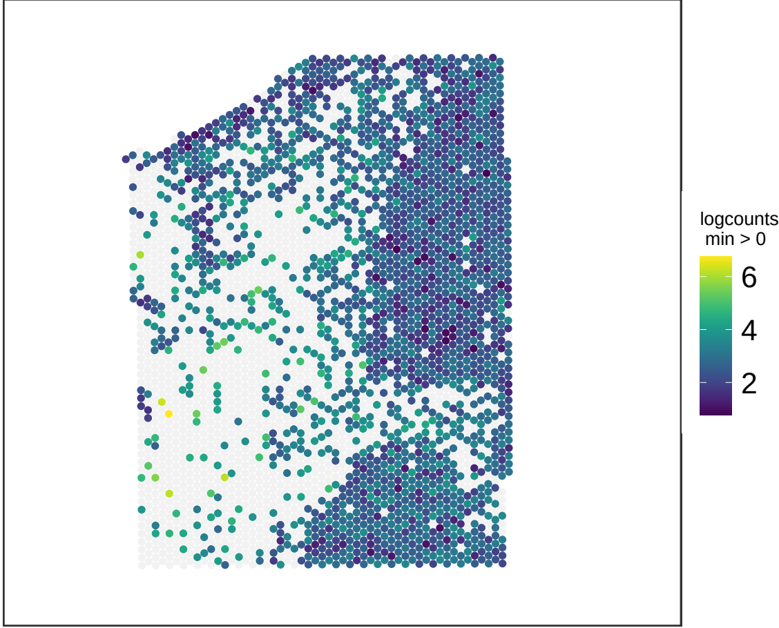
V13M06-387_D1 ATP1B1
