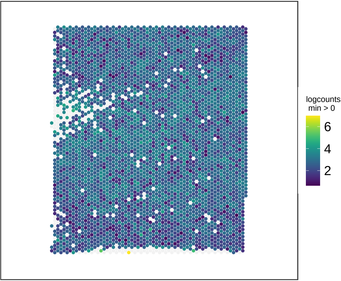
V13M06-388_D1 ATP1B1
