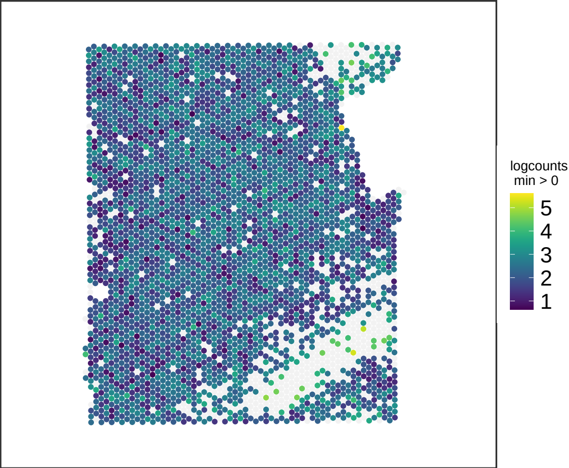
V13M06-387_A1 ATP1B1
