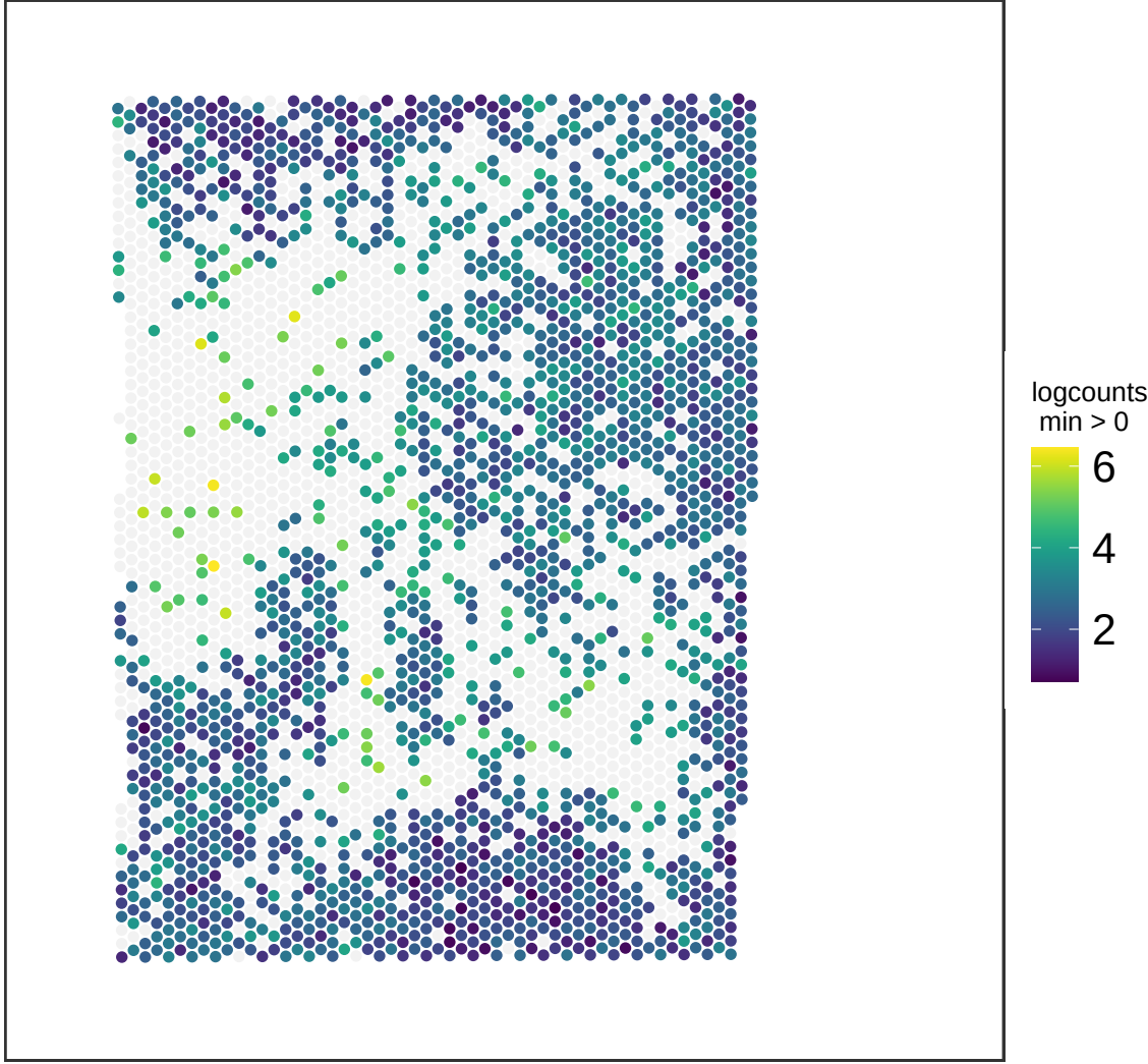
V13M06-387_C1 ATP1B1
