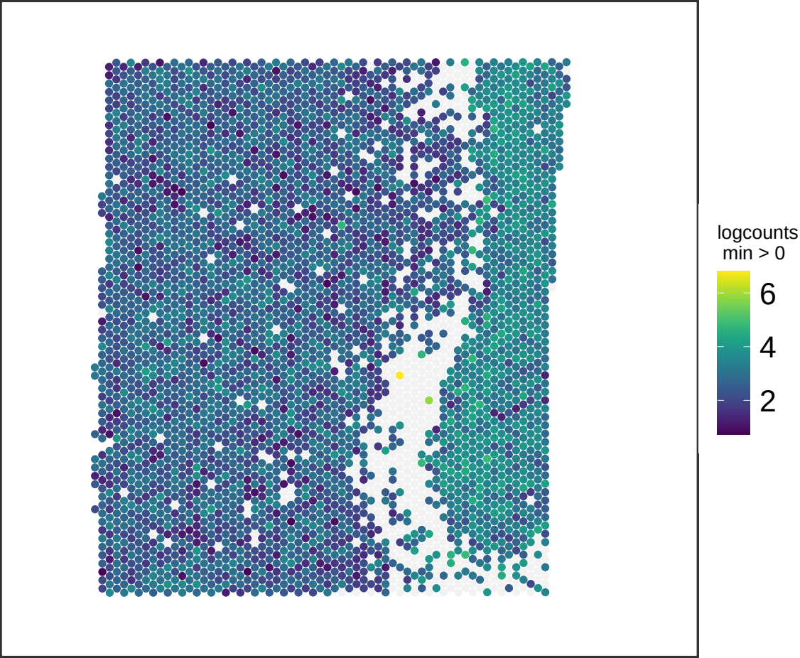
V13M06-388_C1 ATP1B1
