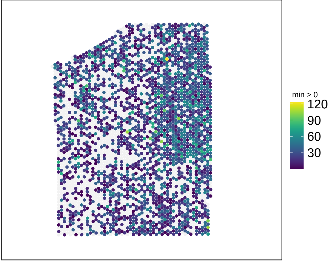
V13M06-387_D1 NMF_10
