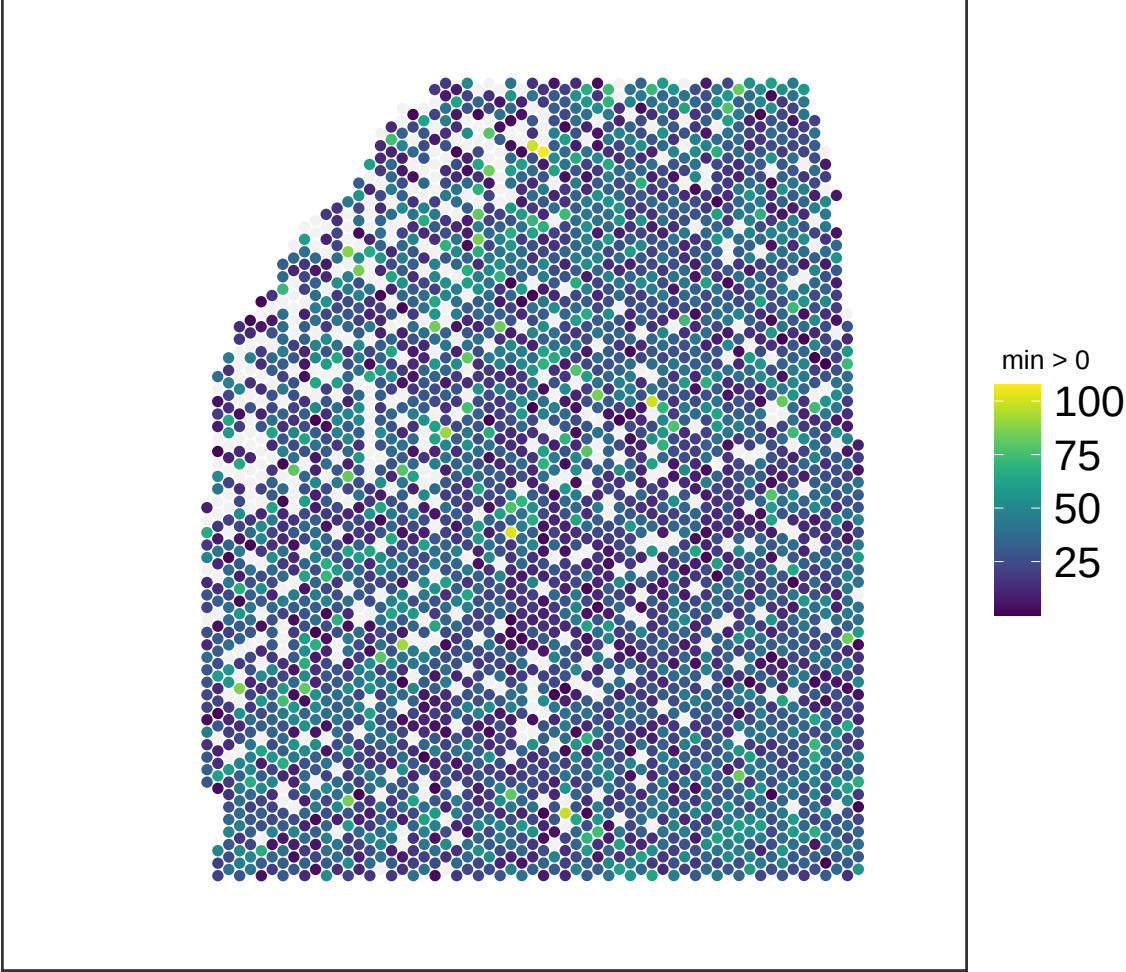
V13M06-388_B1 NMF_10
