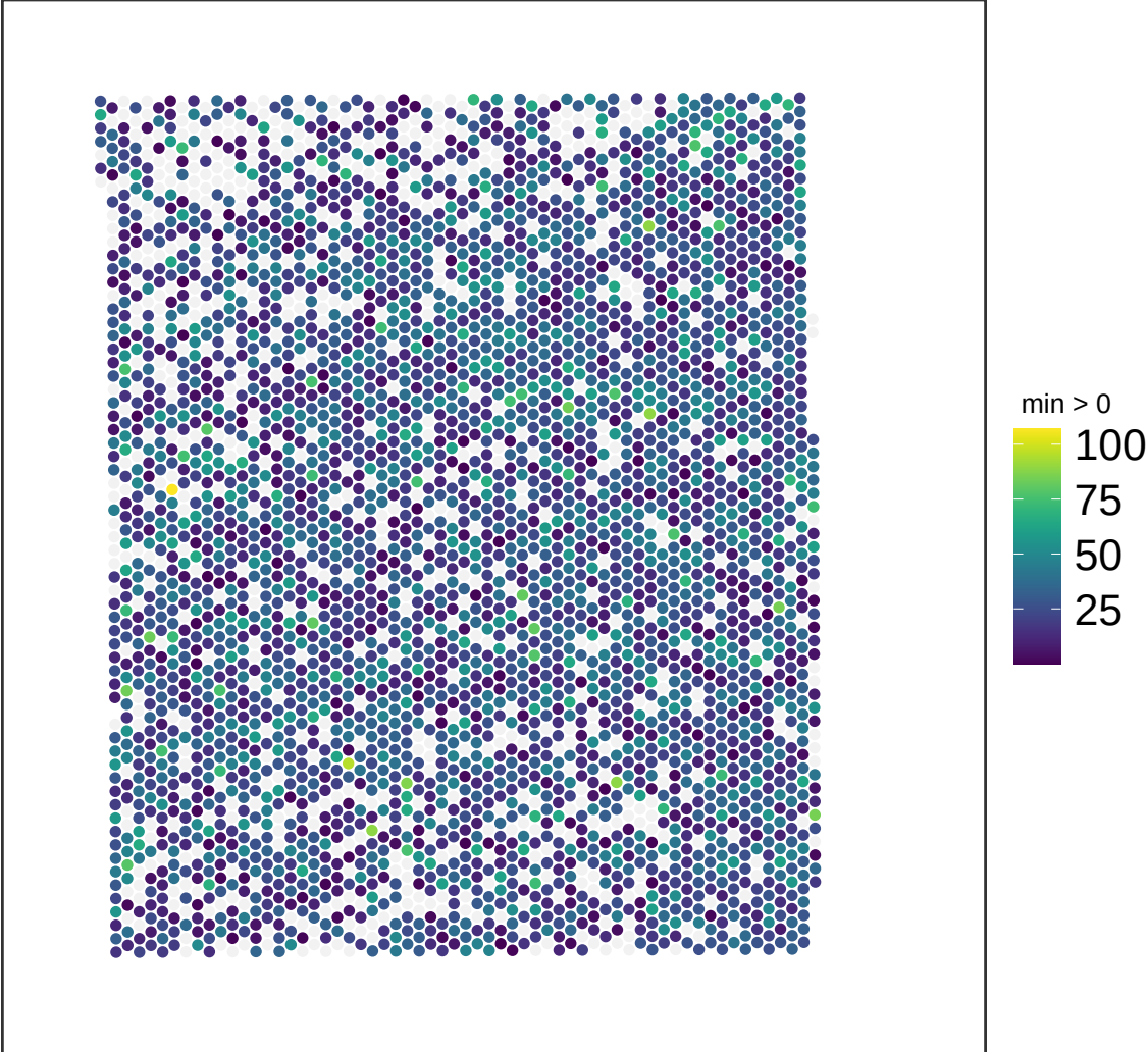
V13M06-387_B1 NMF_10
