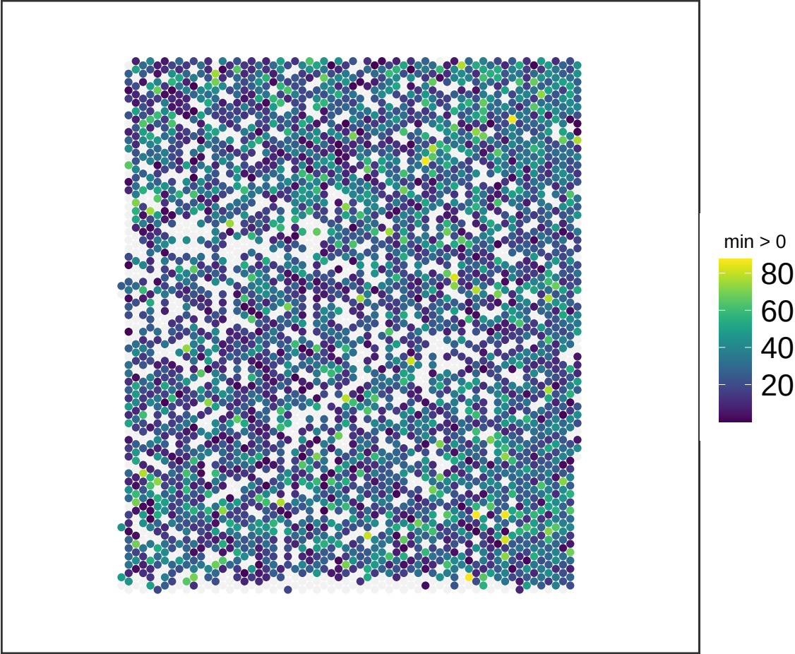
V13M06-388_D1 NMF_10
