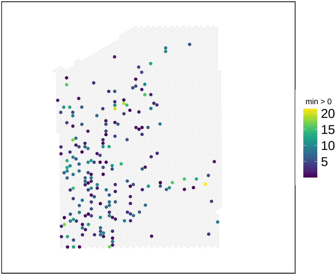
V13M06-387_D1 NMF_66
