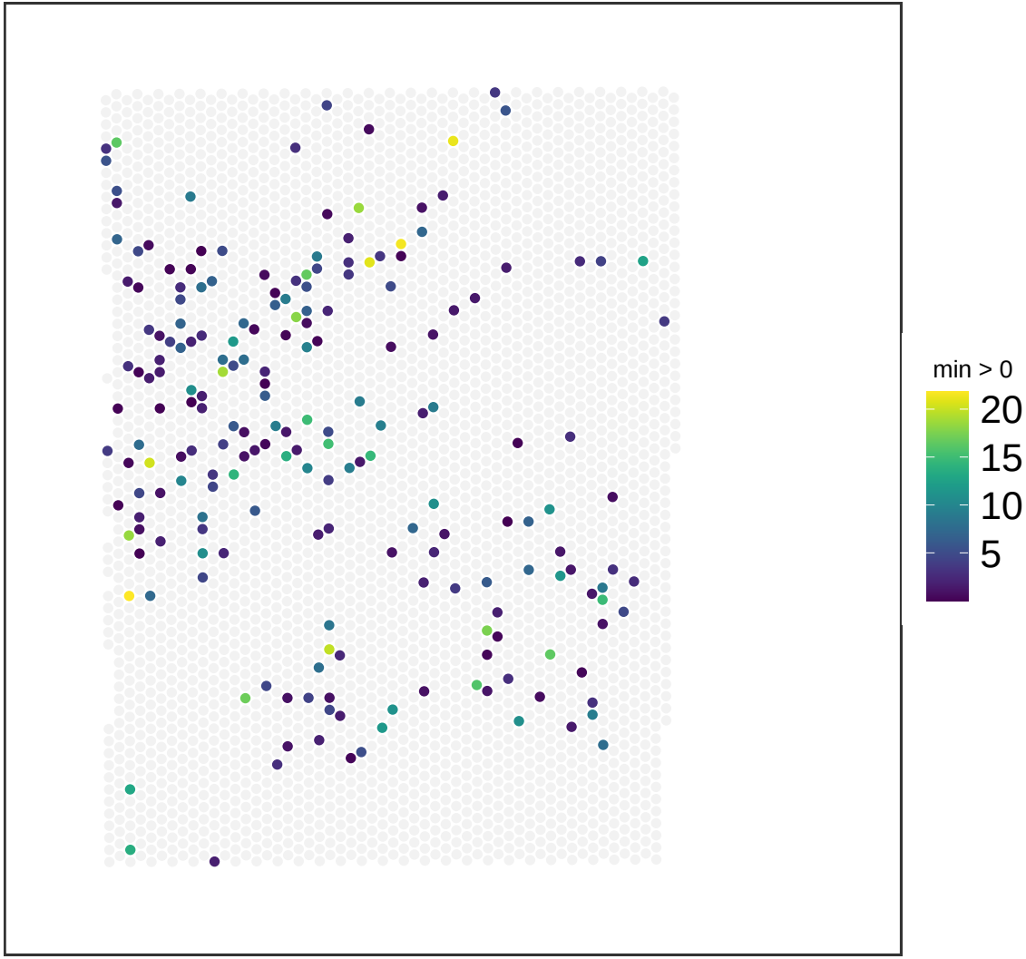
V13M06-387_C1 NMF_66
