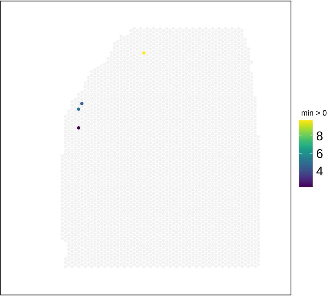
V13M06-388_B1 NMF_66
