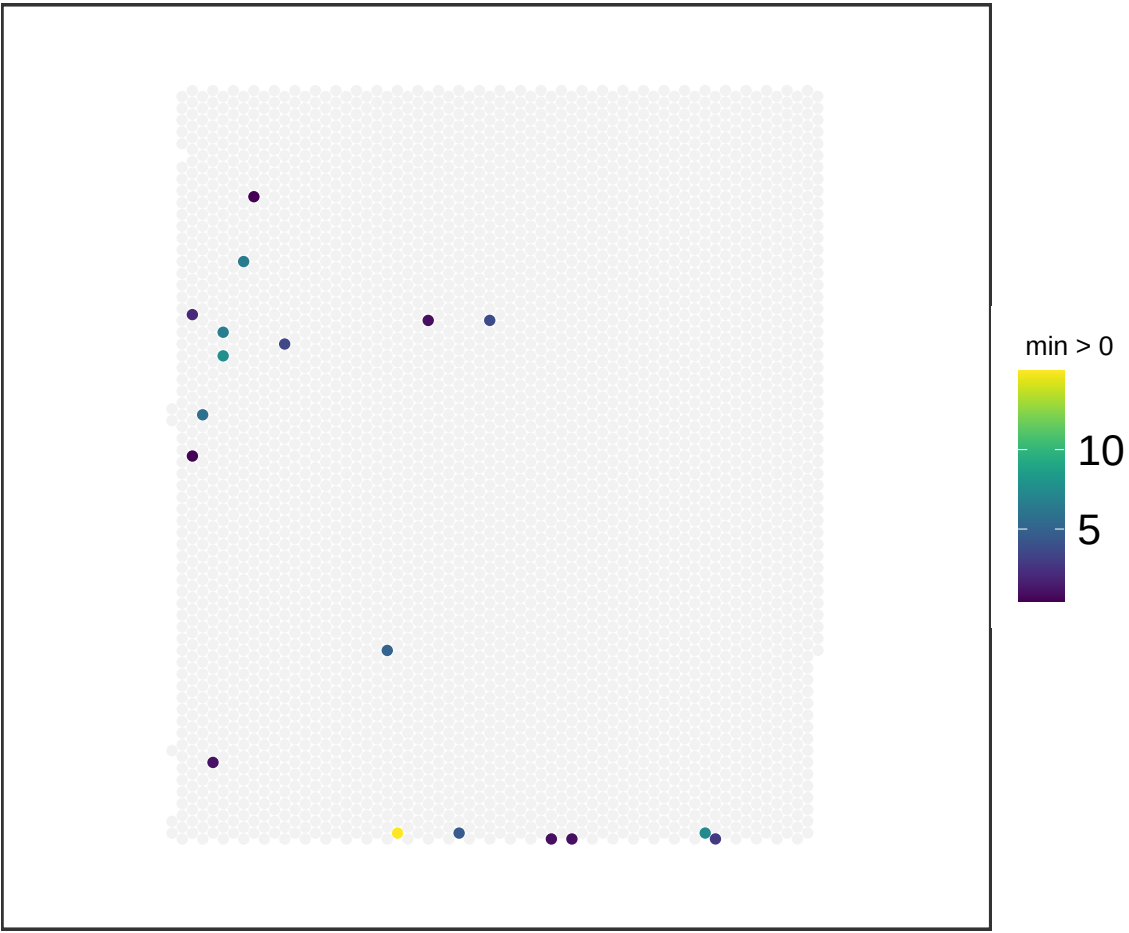
V13M06-388_D1 NMF_66
