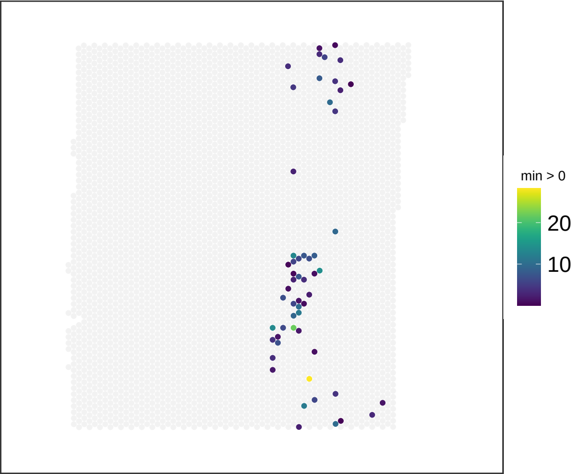
V13M06-388_C1 NMF_66
