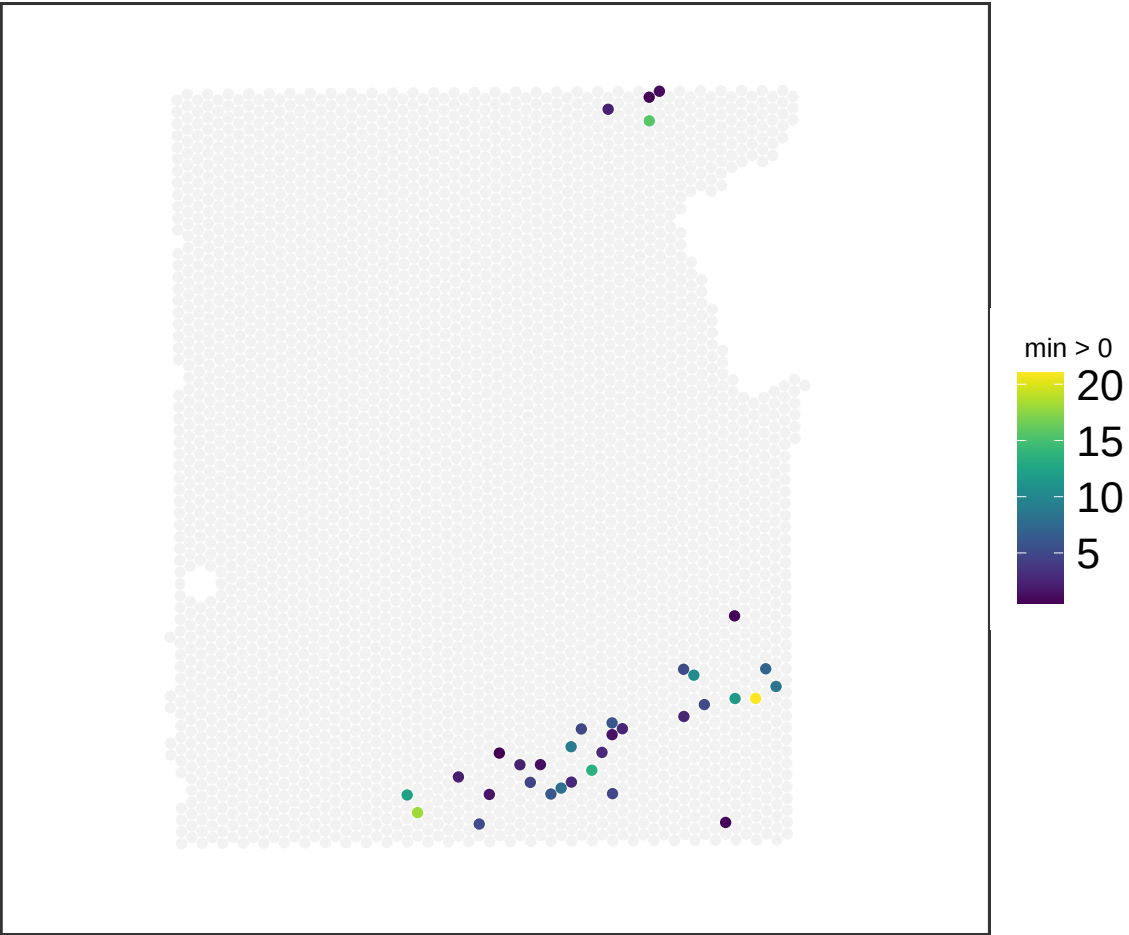
V13M06-387_A1 NMF_66
