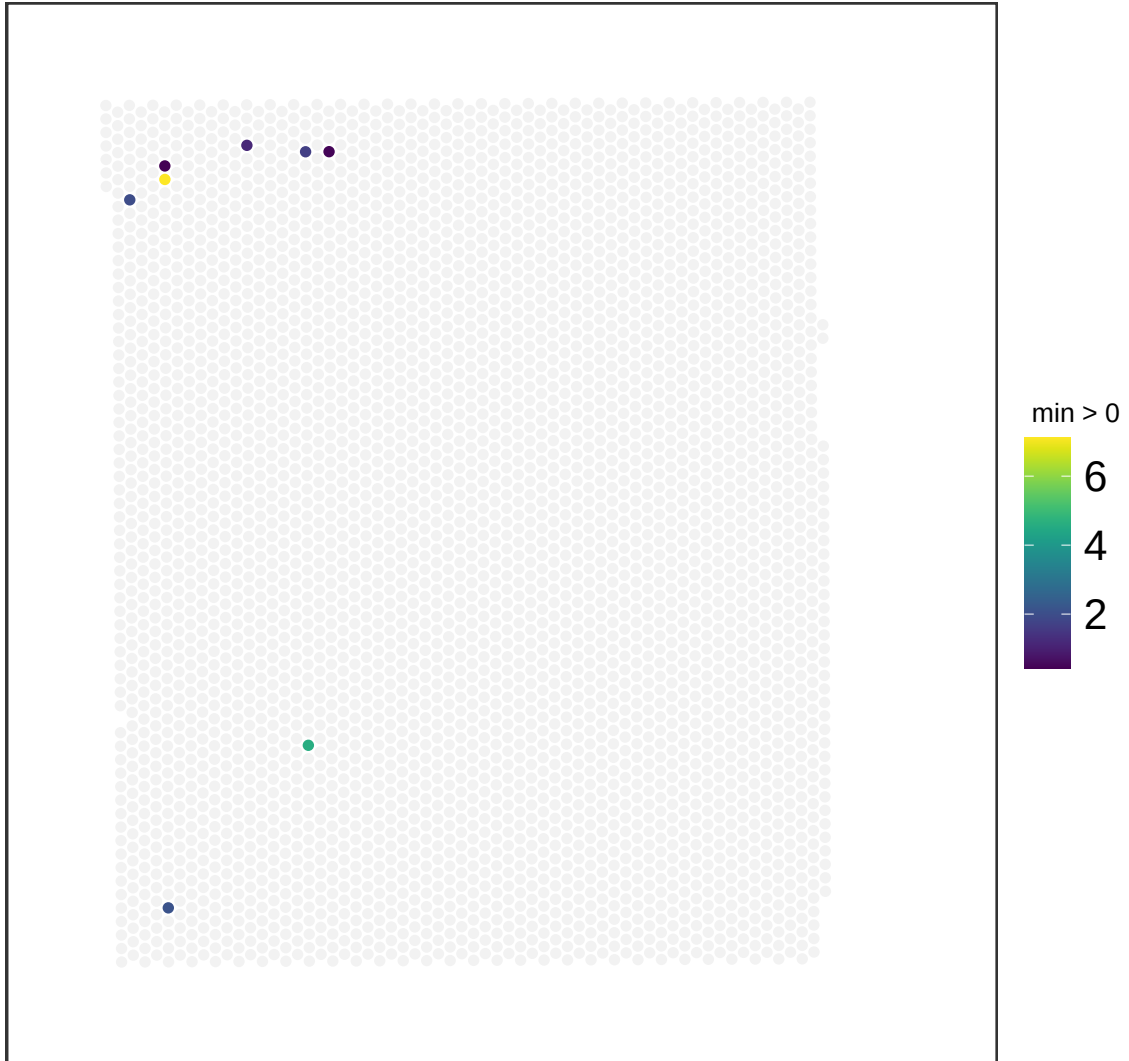
V13M06-387_B1 NMF_66
