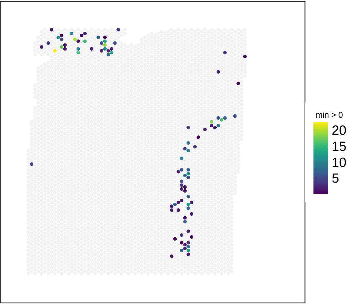
V13M06-388_A1 NMF_66
