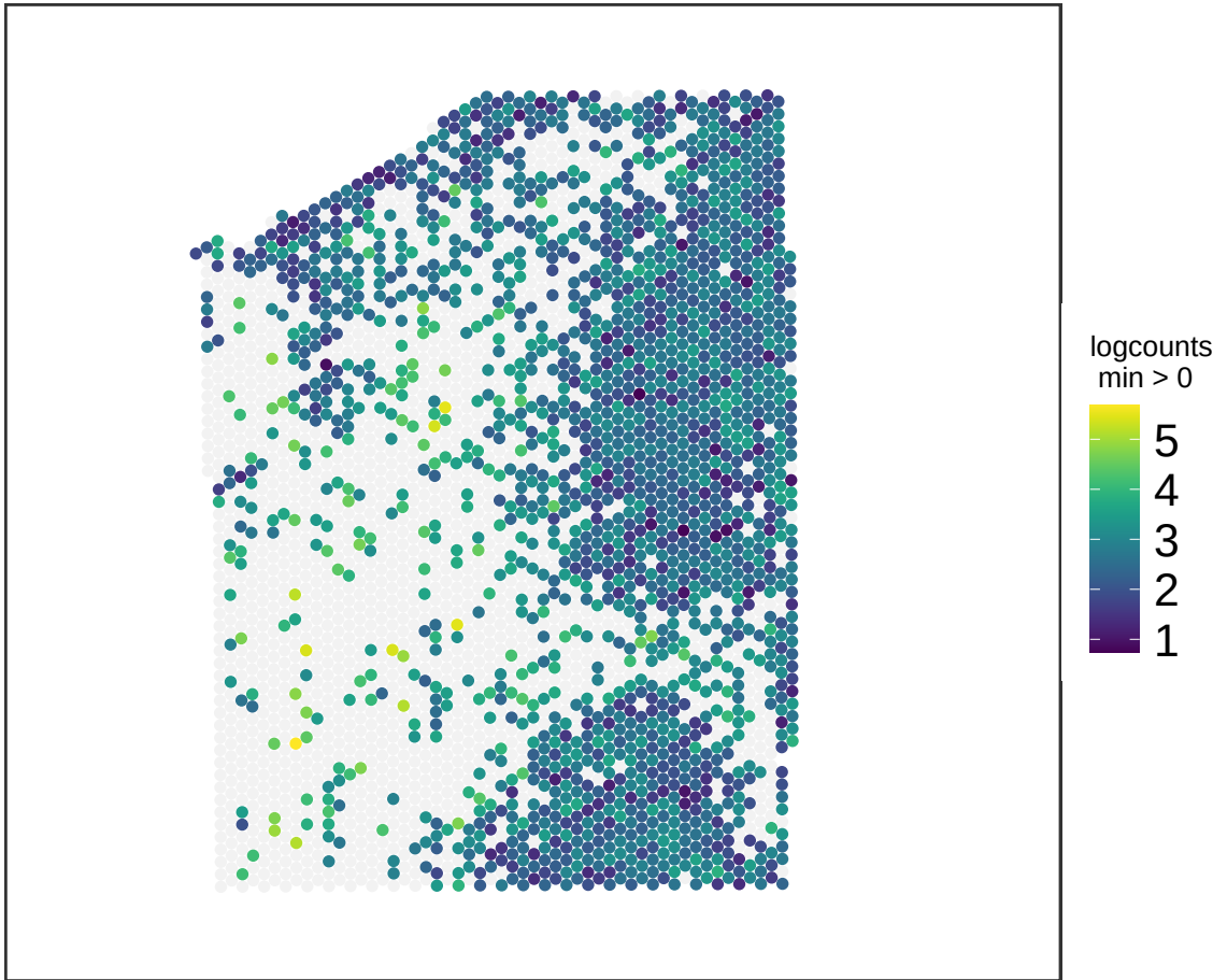
V13M06-387_D1 RTN1
