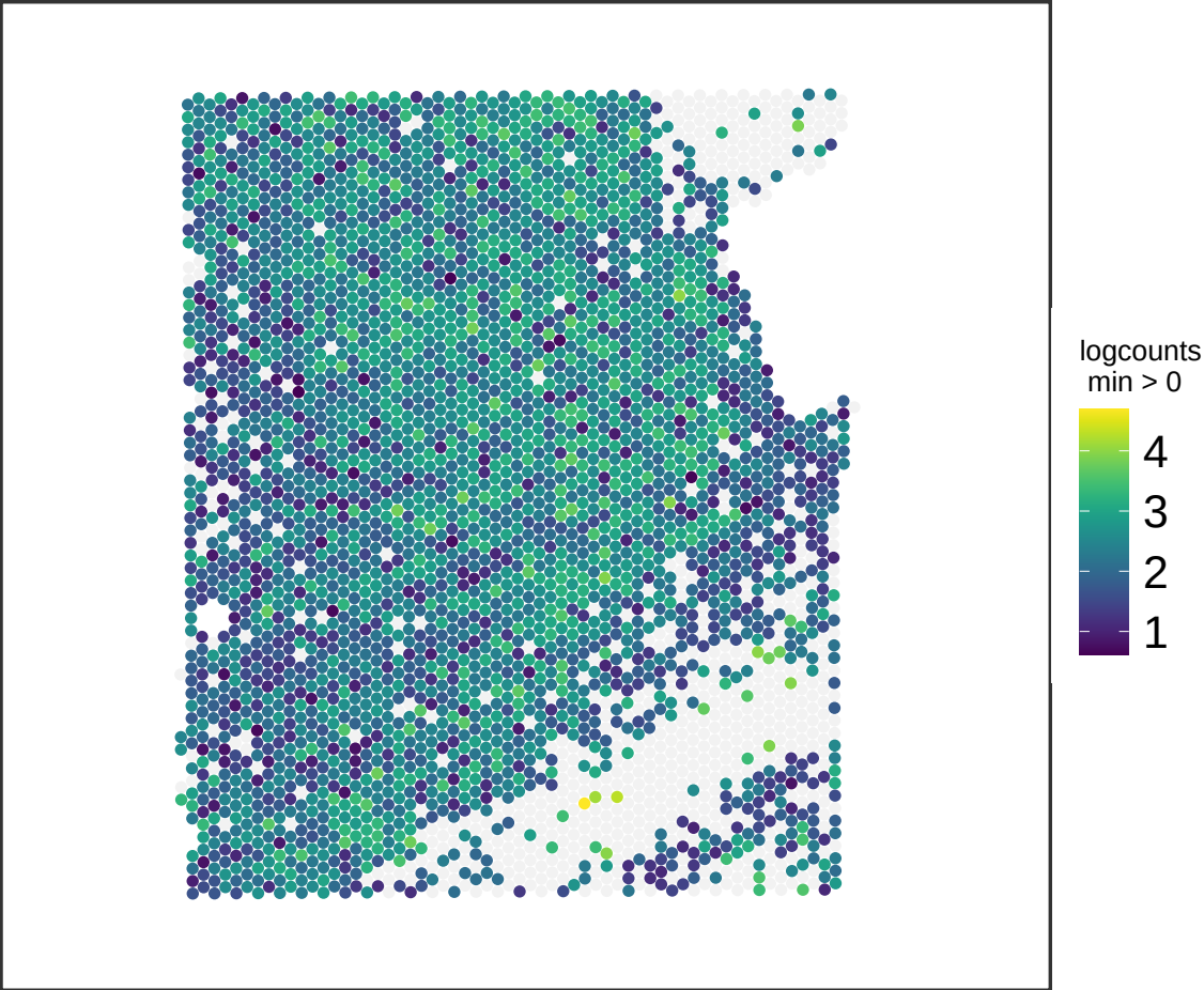
V13M06-387_A1 RTN1
