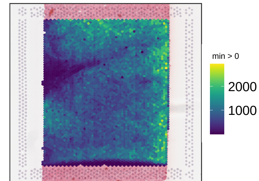
V13M06-388_D1 expr_chrM
