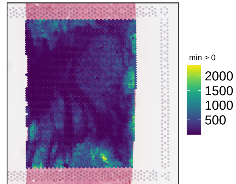
V13M06-387_C1 expr_chrV
