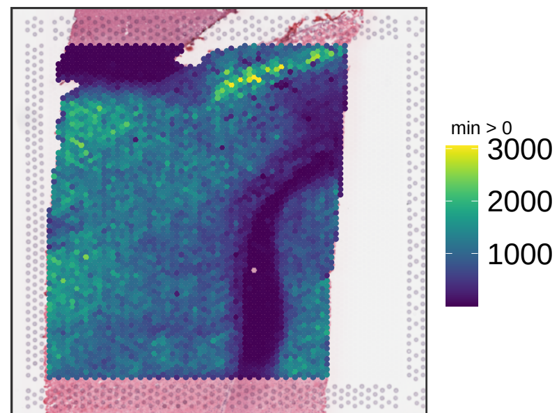
V13M06-388_A1 expr_chrM
