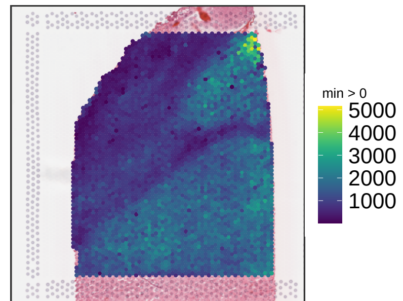
V13M06-388_B1 expr_chrM
