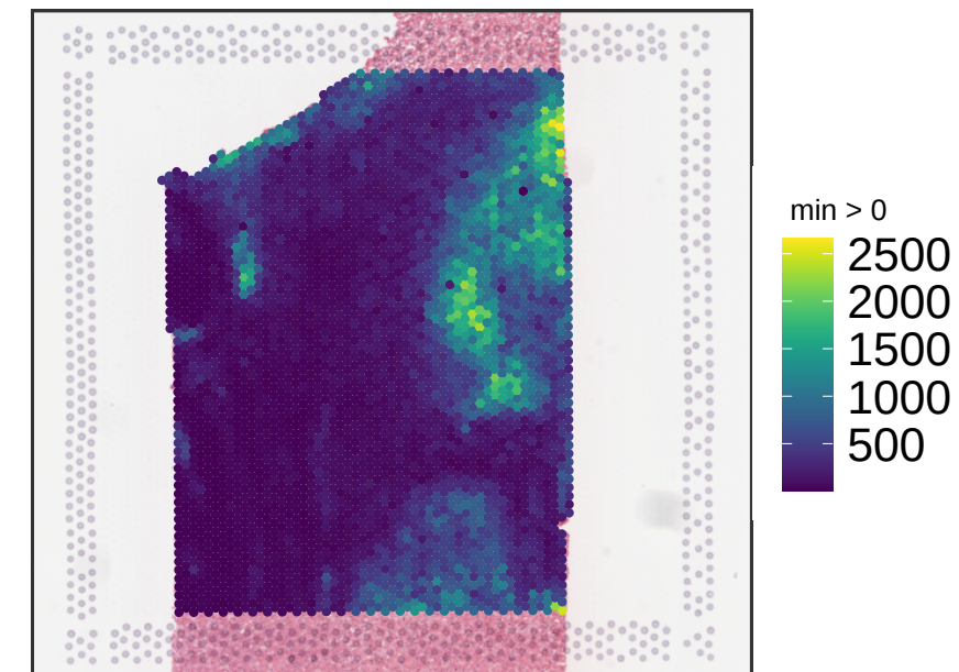
V13M06-387_D1 expr_chrM
