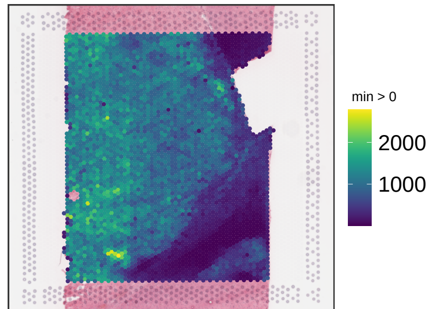
V13M06-387_A1 expr_chrM
