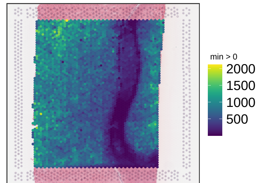
V13M06-388_C1 expr_chrM
