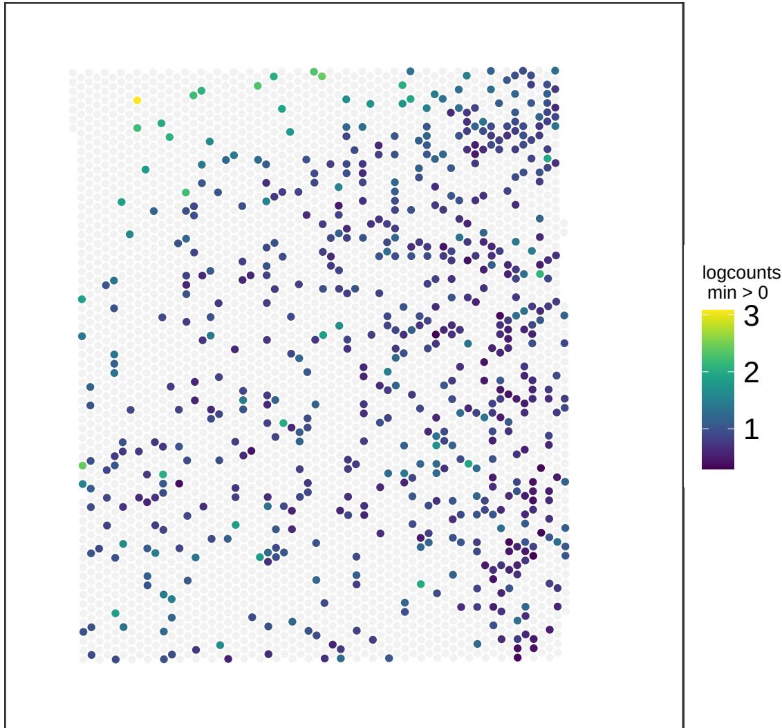
V13M06-387_B1 BHLHE22
