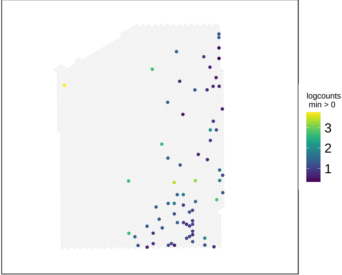
V13M06-387_D1 BHLHE22
