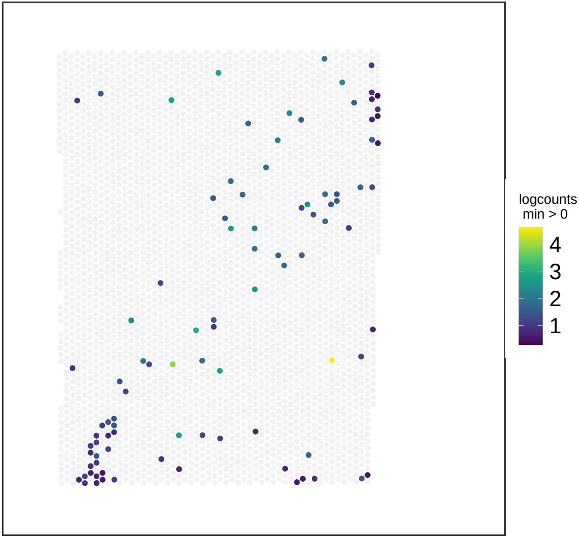
V13M06-387_C1 BHLHE22
