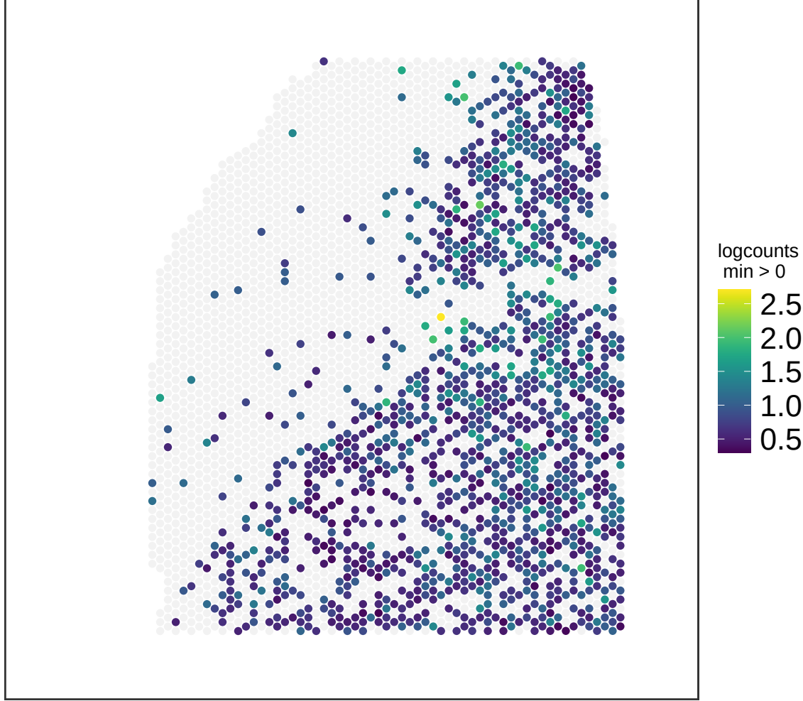
V13M06-388_B1 BHLHE22
