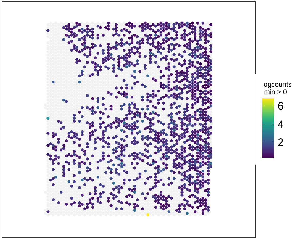
V13M06-388_D1 BHLHE22
