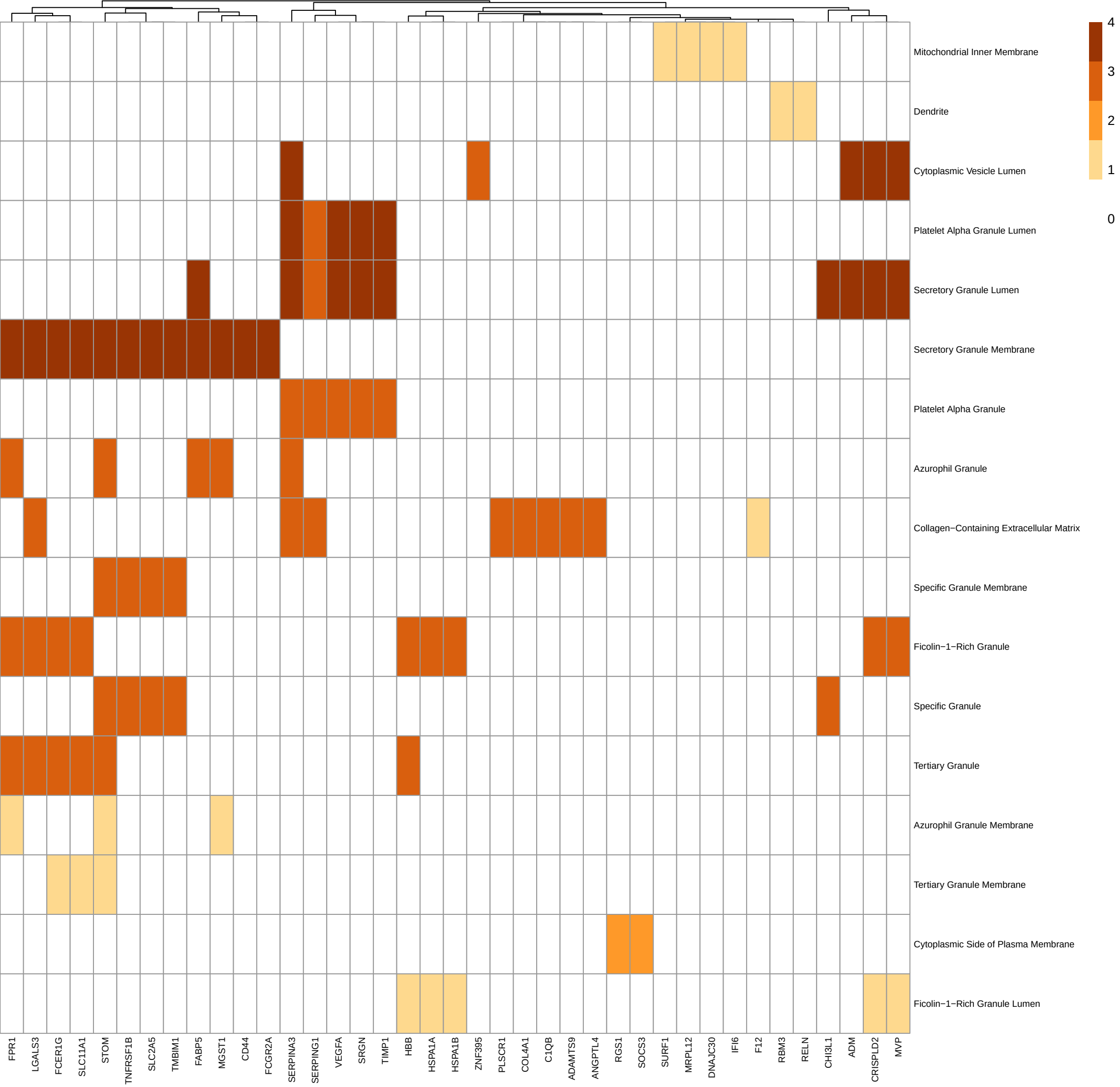
NTC.MDD F GO-CC Fill: # clusters
