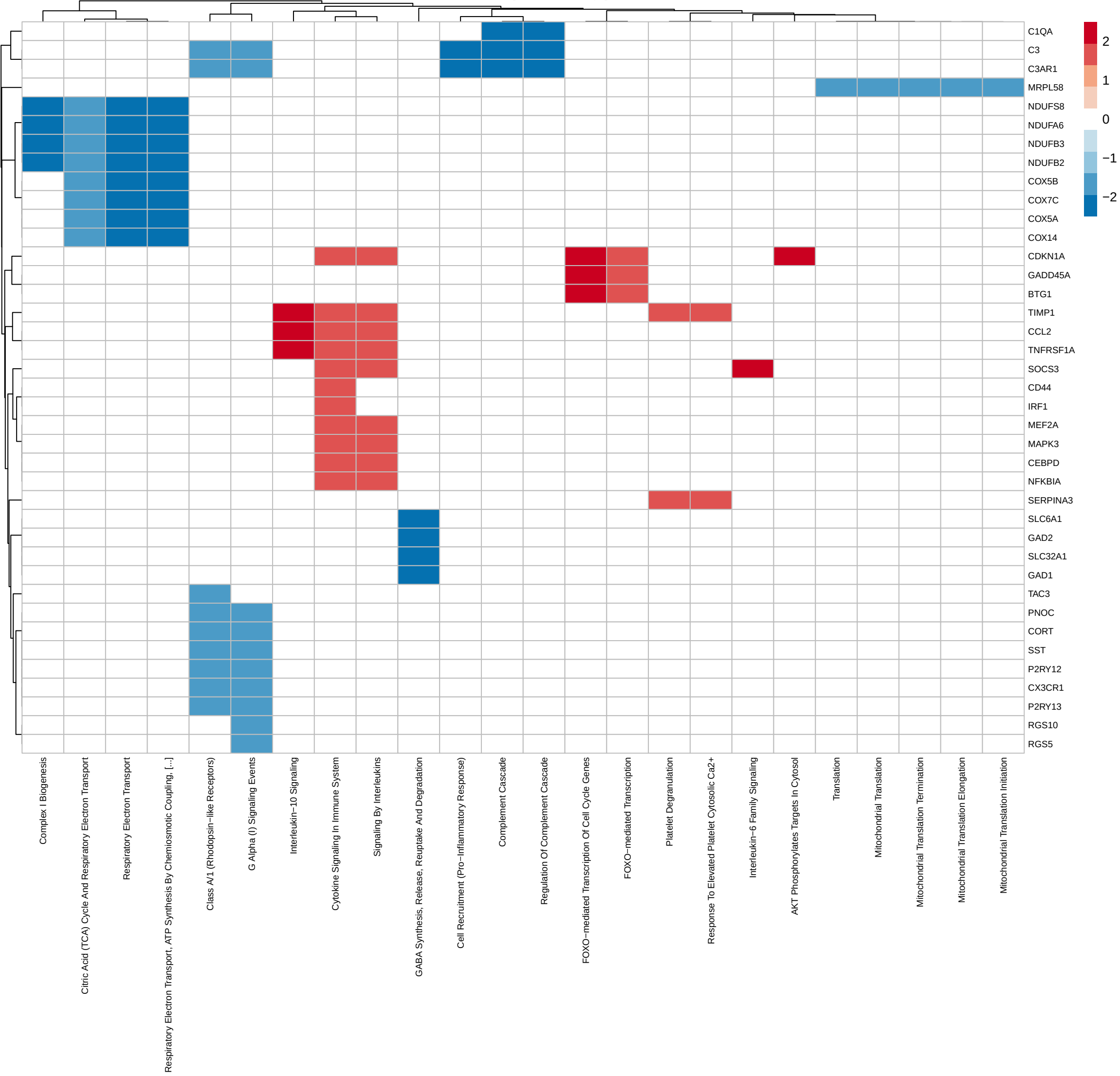
NTC.BPD M Reactome Fill: NES (0 if not sig.)
