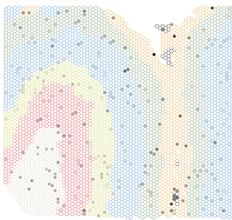
EDN1
