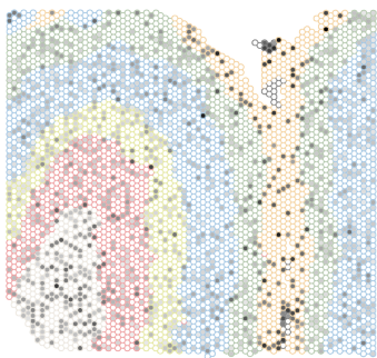
CD34
