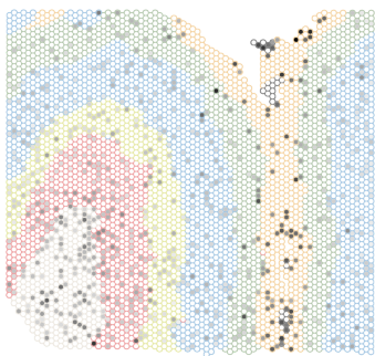
SLCO4A1
