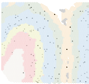
A2M
