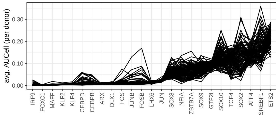
Initial regulons (n=119)
