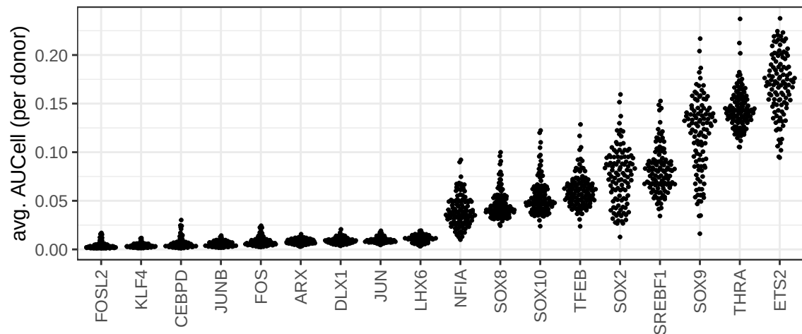
Final regulons (n=109)
