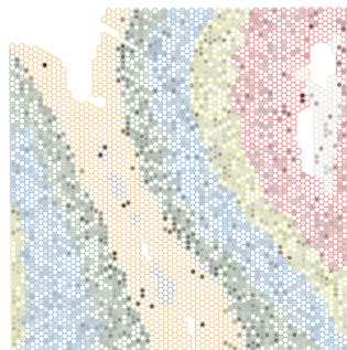
V13B23-334_C1
