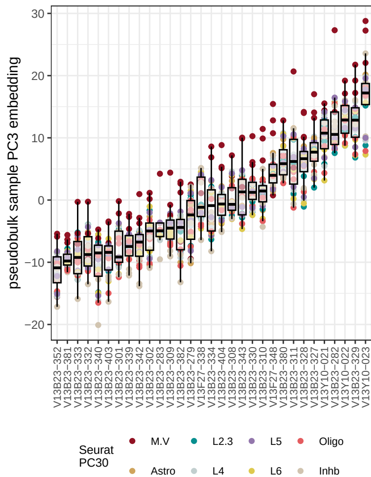
Seurat PC30
