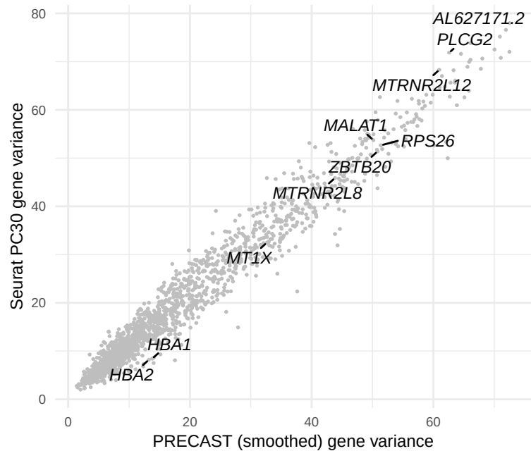
Seurat PC30
