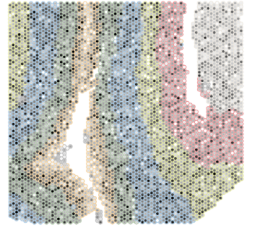
MDD M
