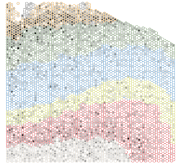
MDD F
