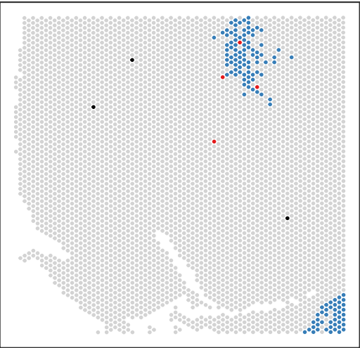
sum.outlier_f
