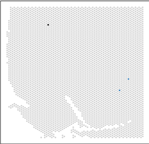
chrM.outlier_f
