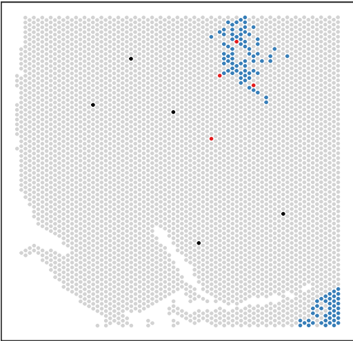
genes.outlier_f
