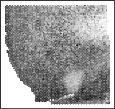
expr_chrM_ratio
