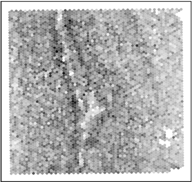
expr_chrM_ratio
