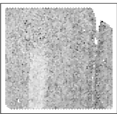
expr_chrM_ratio
